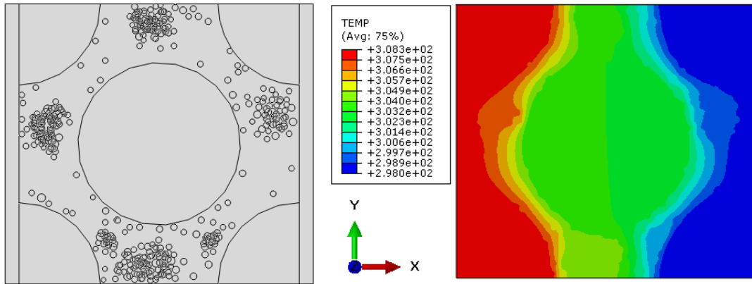
Şekil 5.44 %10 CNT ilavesi yapılmış ve aglomerasyon oluşmuş modelin analiz sonucu.
