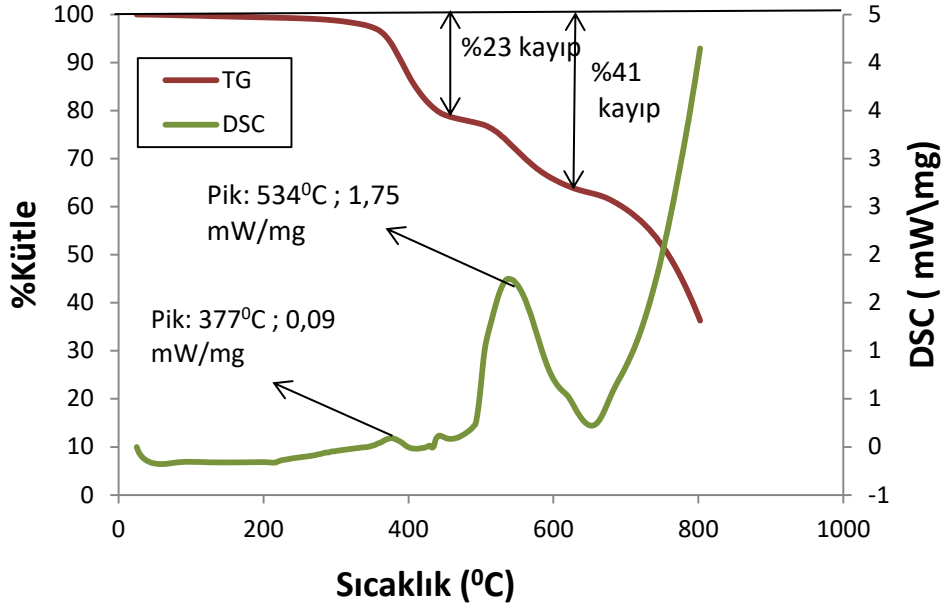
Şekil 5.12 CNT katılı T800/M21 numunelerin 5 °C/ dak ısıtma hızında TG-DSC diyagramları.
