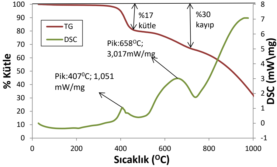
Şekil 5.10 T800/M21 numunelerin 20 0 C/ dak ısıtma hızında TG-DSC diyagramları.
