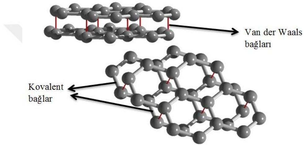
Şekil 2.5 Grafitin atom yapısı (İnt.Kyn.6).
