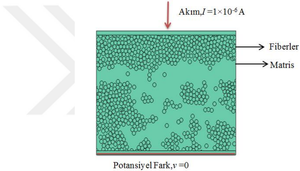
Şekil 5.33 500 büyütmeye sahip mikro yapı görüntüsünden elde edilen model.
