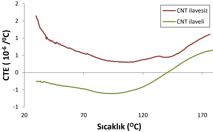
Şekil 5.16 CNT ilavesiz/ilaveli T800/M21 numunelerin X doğrultusunda termal genleşme katsayıları.
