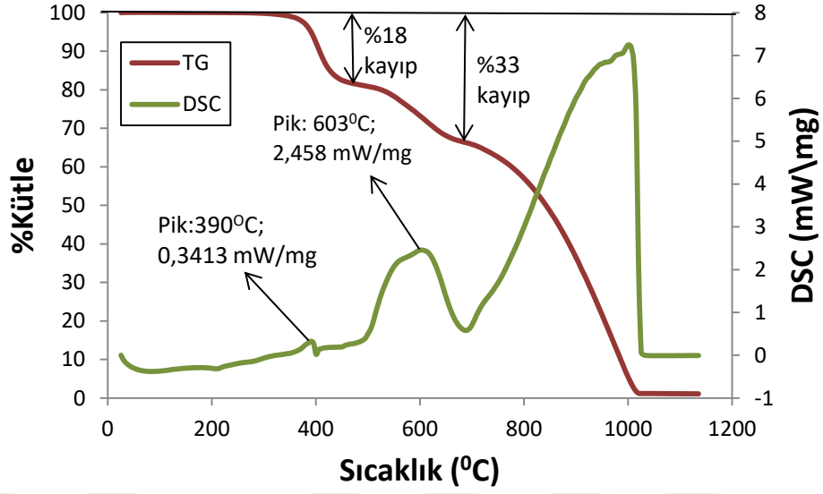
Şekil 5.9 T800/M21 numunelerin 10 0 C/ dak ısıtma hızında TG-DSC diyagramları.
