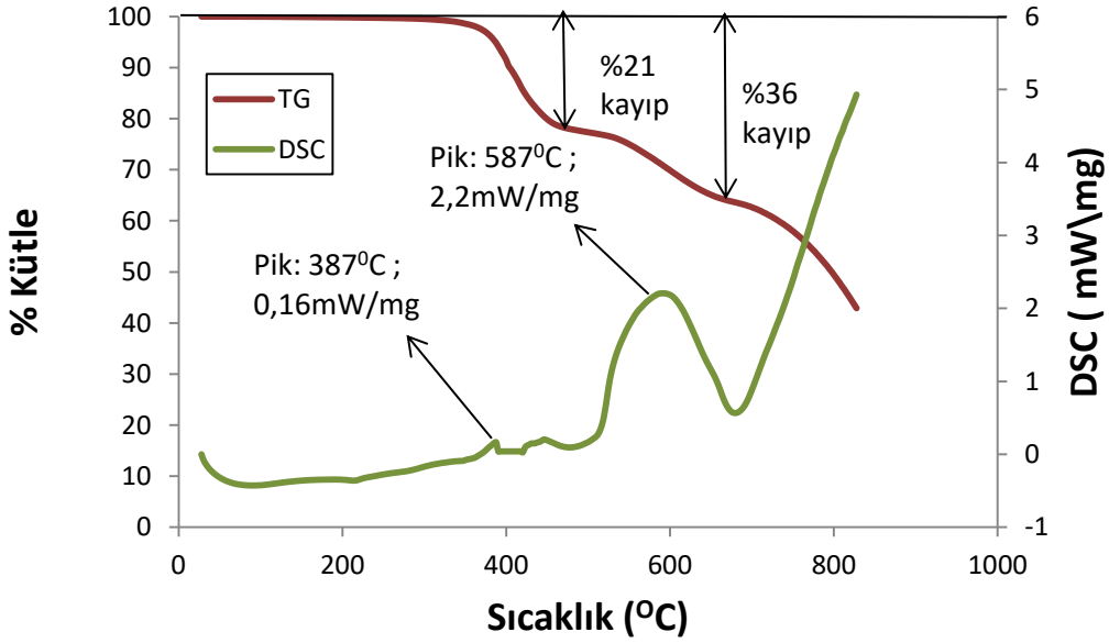
Şekil 5.13 CNT katılı T800/M21 numunelerin 10 °C/dak ısıtma hızında TG-DSC diyagramları.
