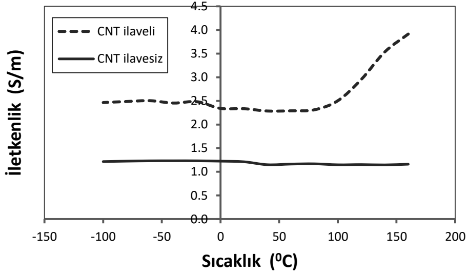
Şekil 5.19 -100 +160°C aralığında CNT ilaveli ve ilavesiz numunelerin elektriksel iletkenlik ölçümleri.
