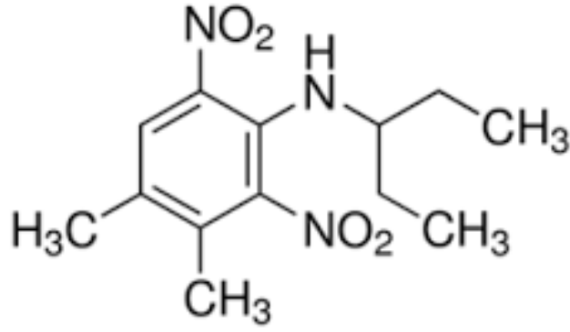
Şekil 2.4 PM herbisitinin kimyasal yapısı.
