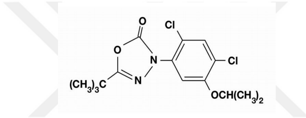
Şekil 2.3 OD herbisitinin kimyasal yapısı.
