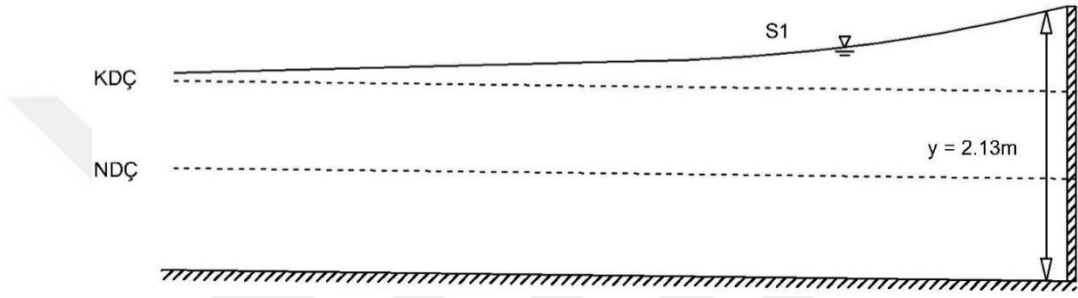
Şekil 4.13: Uygulama 4 için kanal boy kesiti
