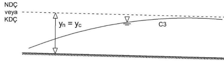
Şekil 1.20: C3 Profili
