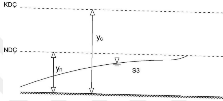
Şekil 1.14: S3 Profili
