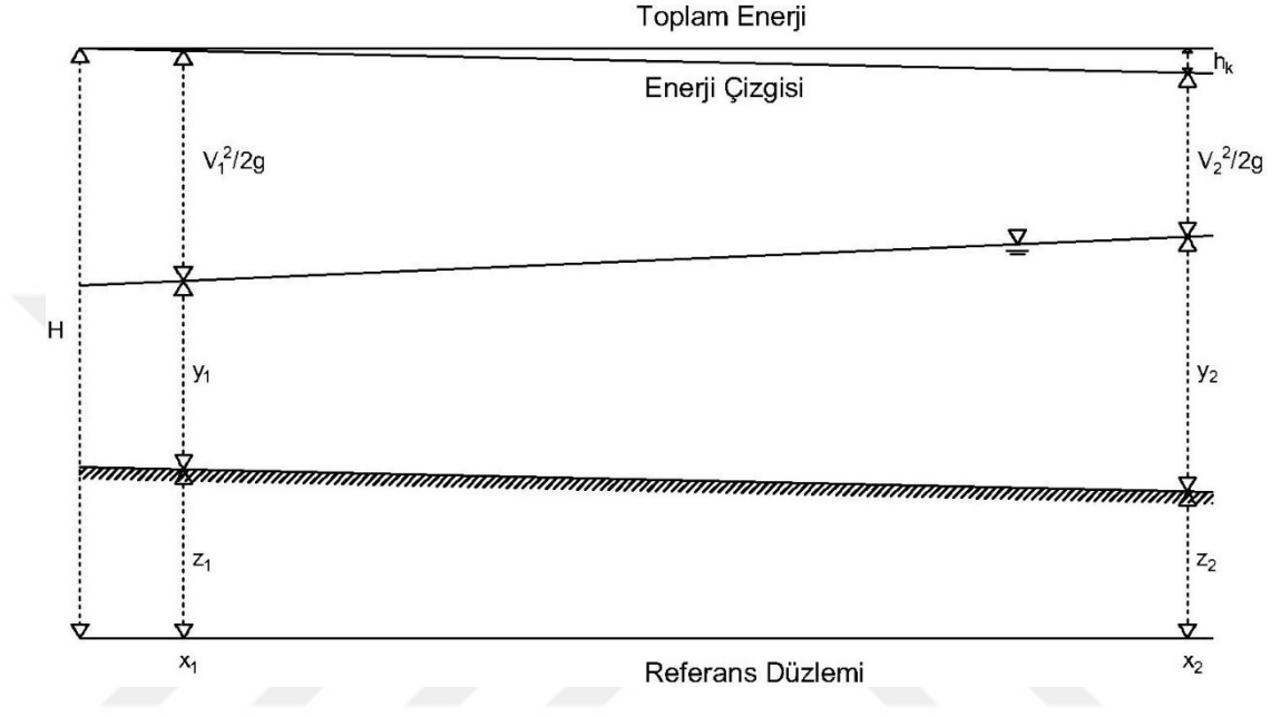
Şekil 3.2: Yatay mesafenin hesaplanması
