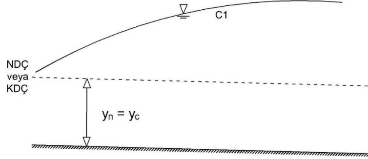
Şekil 1.19: C1 Profili
