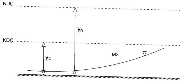
Şekil 1.11: M3 Profili
