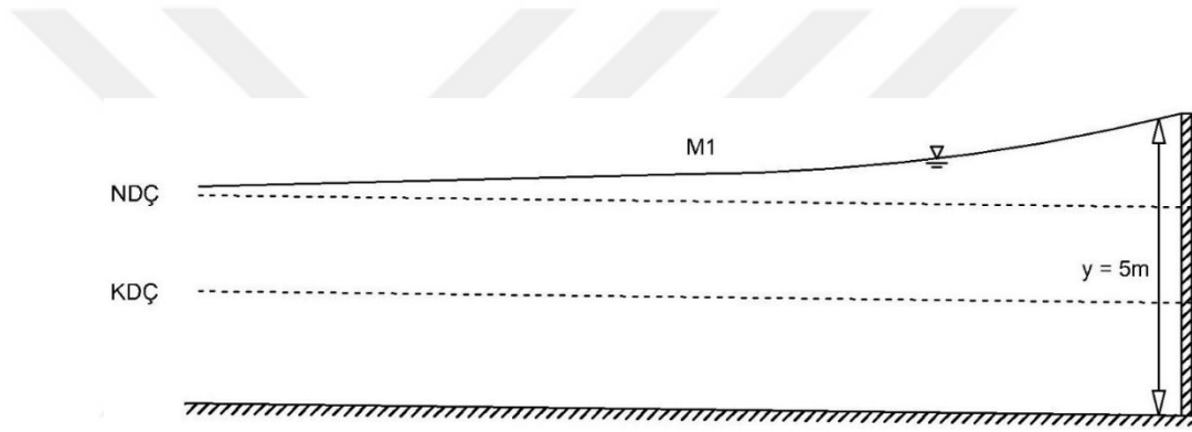
Şekil 4.1: Uygulama 1 için kanal boy kesiti
