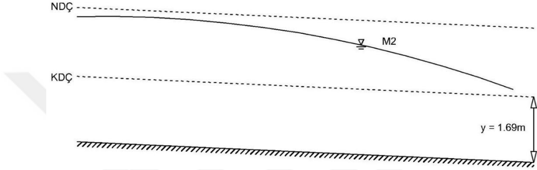
Şekil 4.9: Uygulama 3 için Kanal Boy Kesiti
