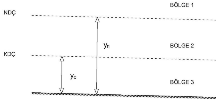
Şekil 1.4: Küçük eğimli kanal tipi (M)
