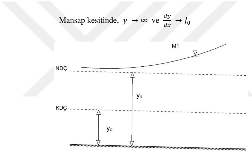
Şekil 1.9: M1 Profili
