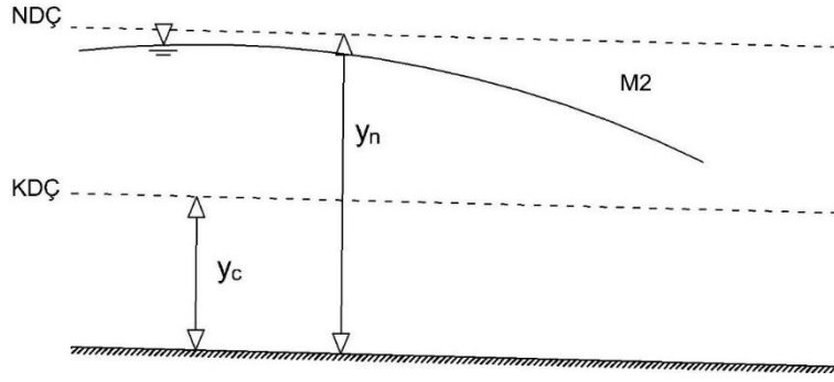
Şekil 1.10: M2 Profili
