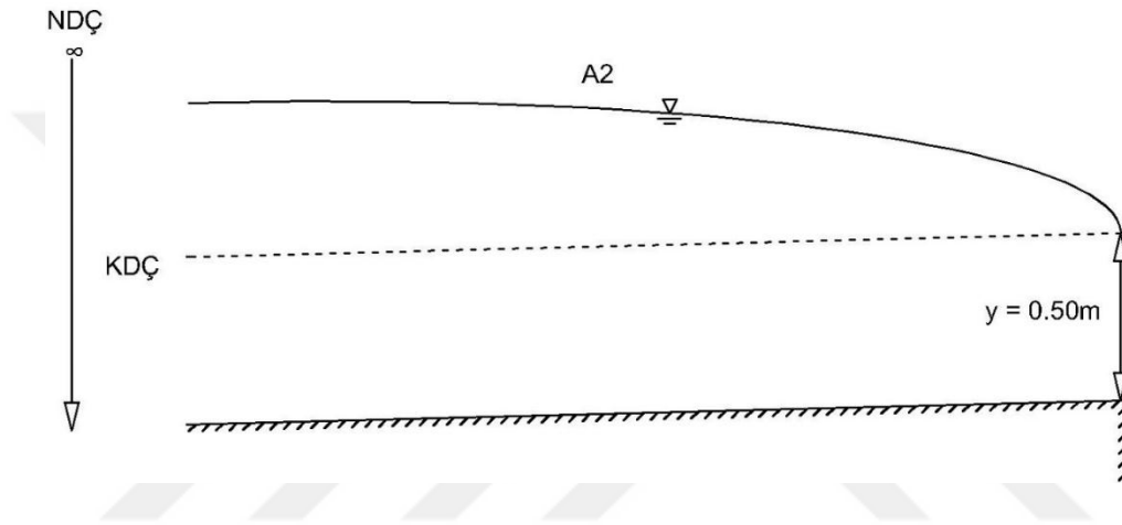
Şekil 4.21: Uygulama 6 için kanal boy kesiti
