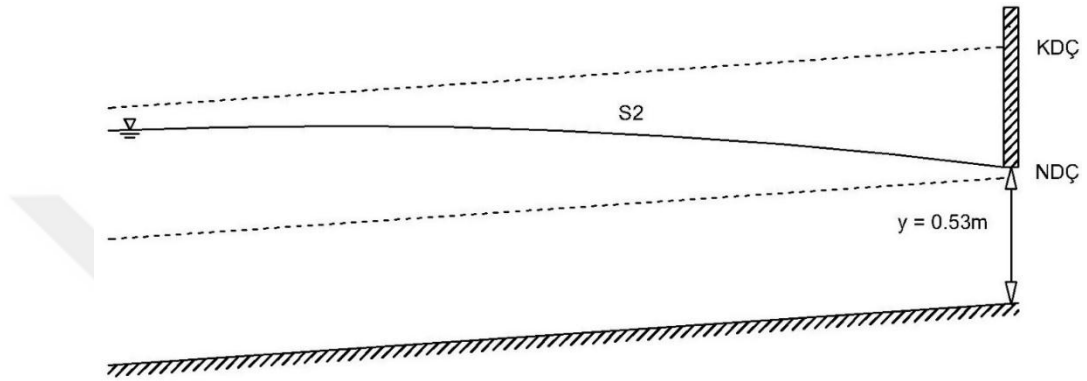
Şekil 4.25: Uygulama 7 için kanal boy kesiti
