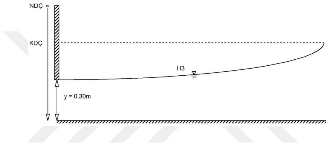
Şekil 4.29: Uygulama 8 için kanal boy kesiti
