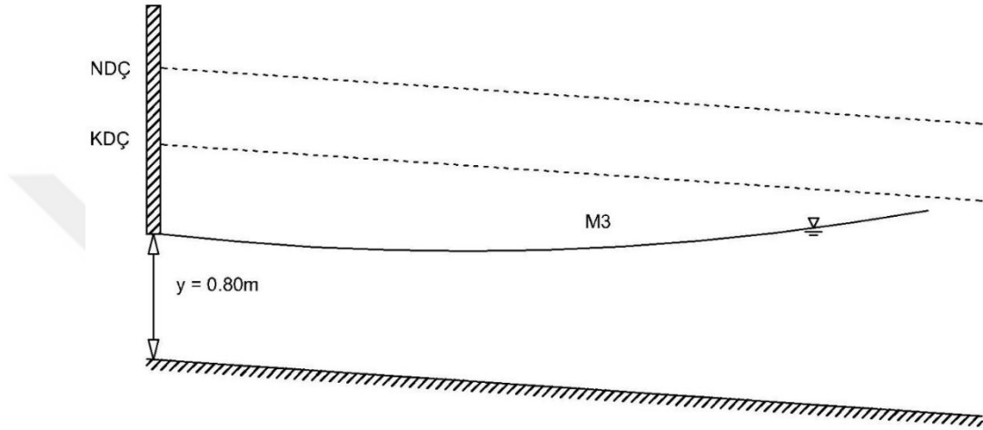
Şekil 4.17: Uygulama 5 için kanal boy kesiti
