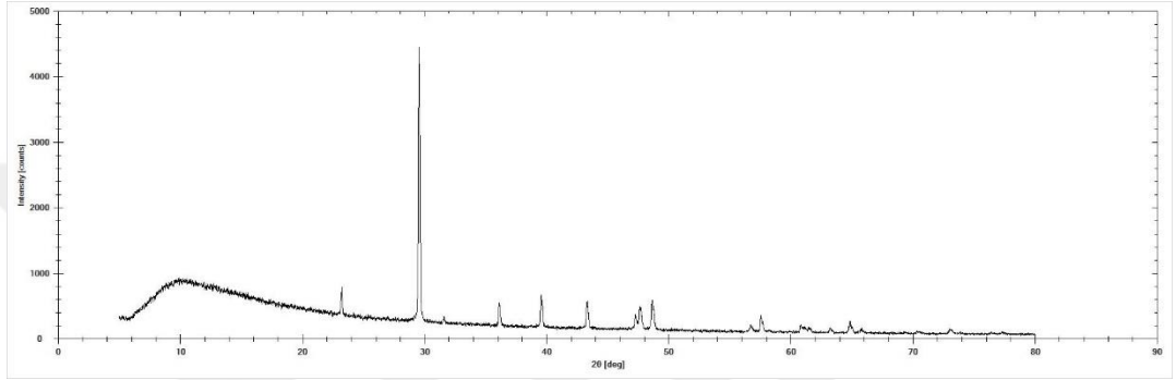
Şekil 4.100: MSA-8 Grafiği
