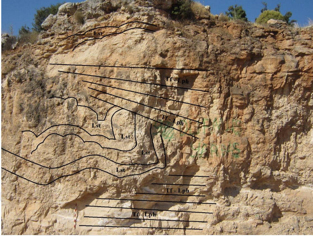
Şekil 3.34: Varsak 2 Kesitinin genel görünümü
