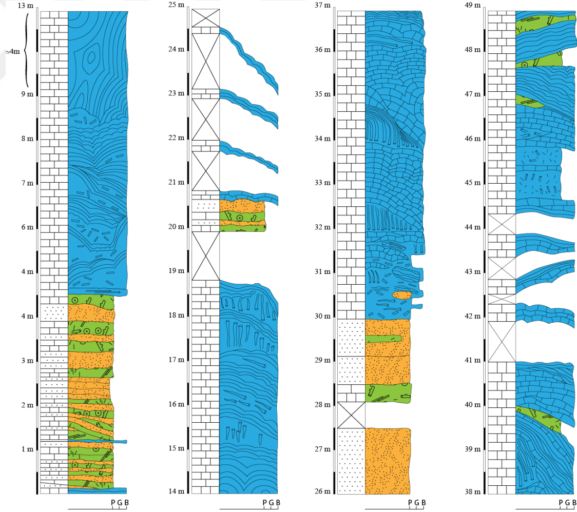
Şekil 3.67: Varsak 7 Ölçülü Kesiti (1)
