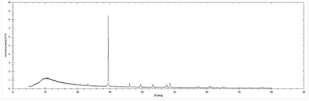
Şekil 4.99: MSA-6 Grafiği
