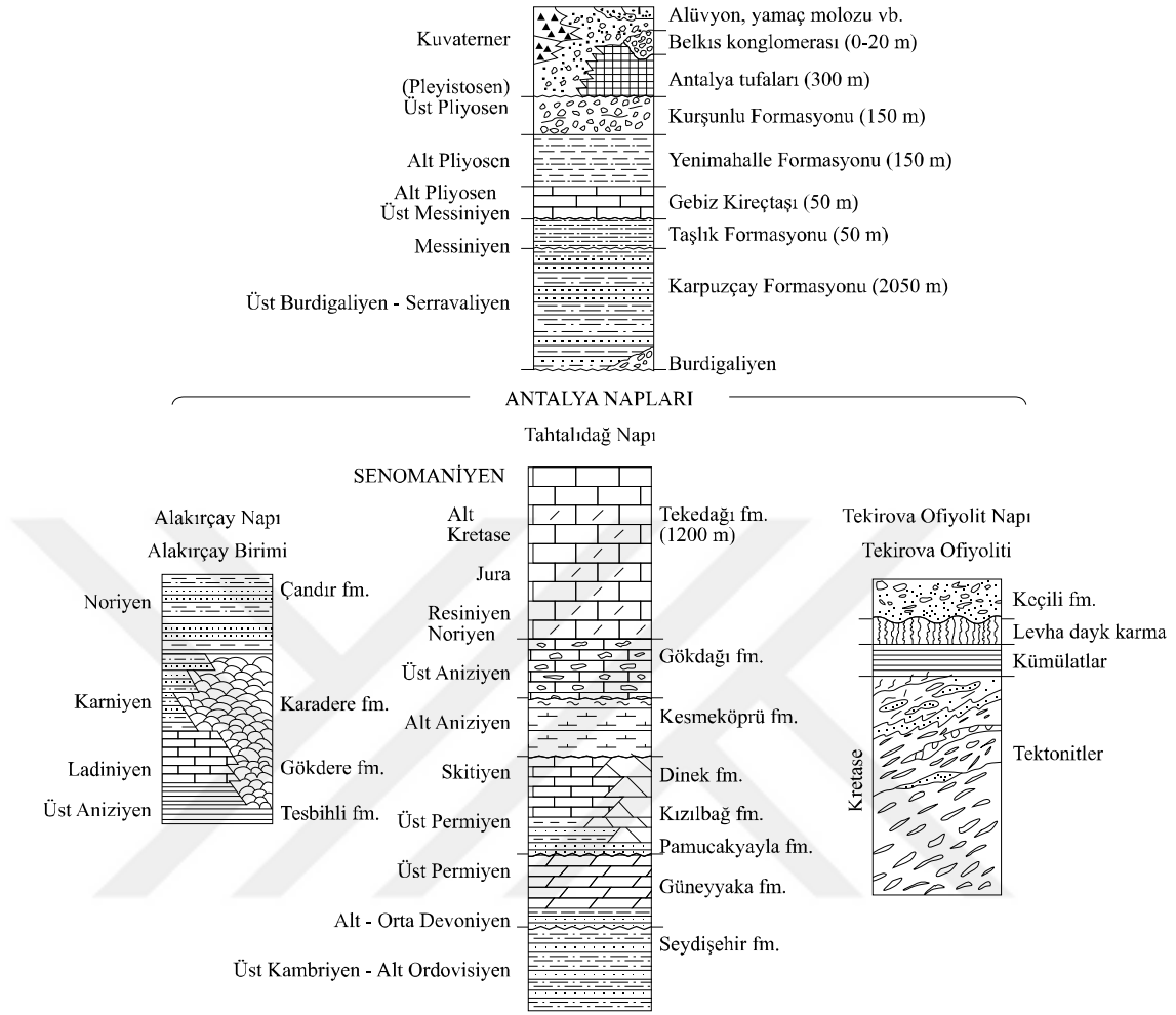
Şekil 2.6: Genelleştirilmiş stratigrafik kesit (MTA'nın raporundan basitleştirilerek yeniden çizilmiştir)
