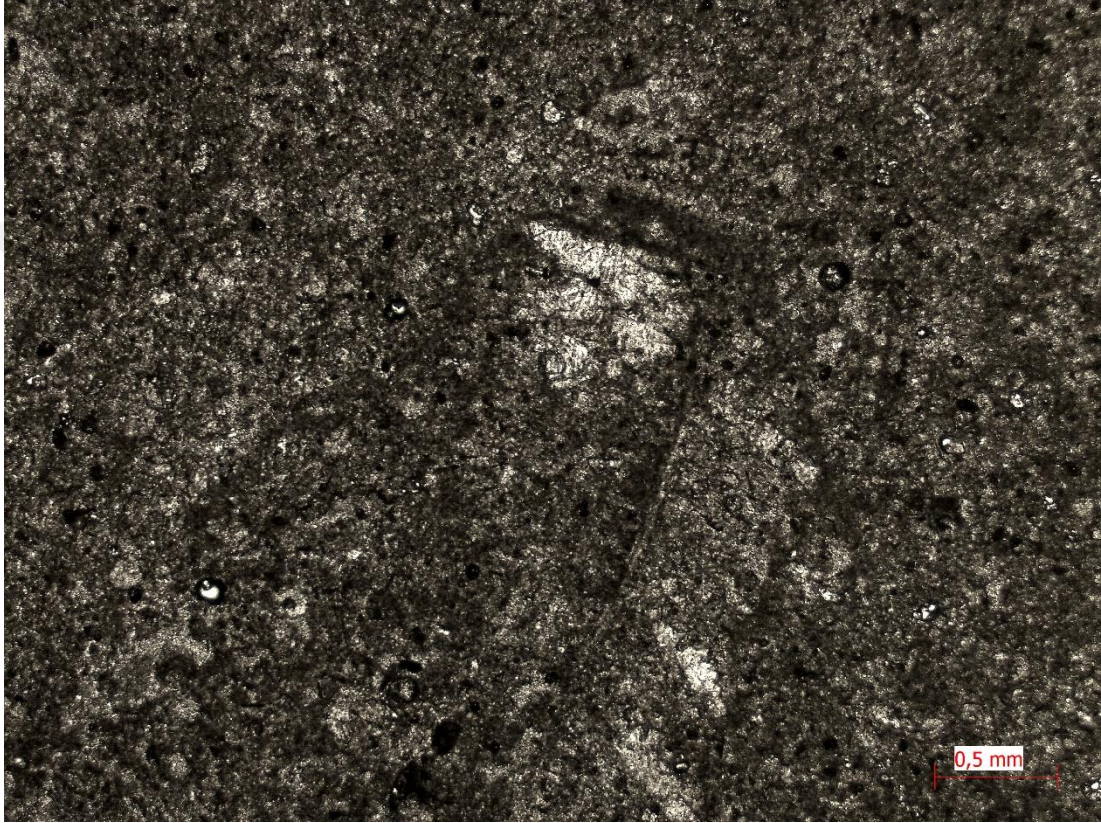
Şekil 3.36: MSA-13 ince kesit görüntüsü
