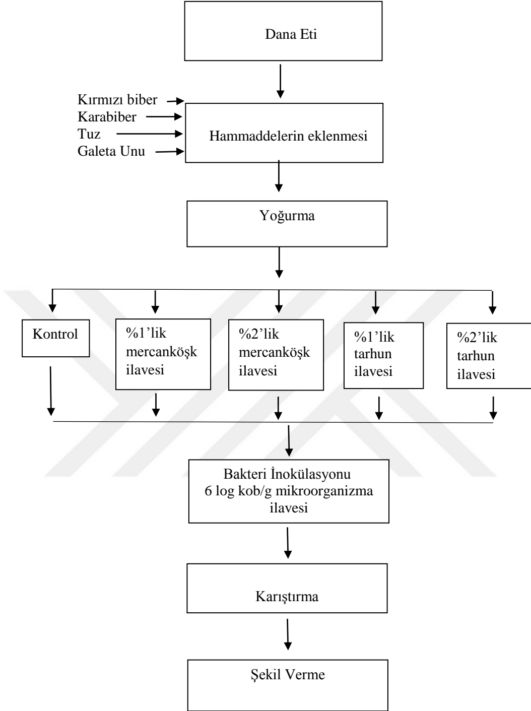
Şekil 3.1 Hamburger Köftesi Üretimi Akış Şeması.
