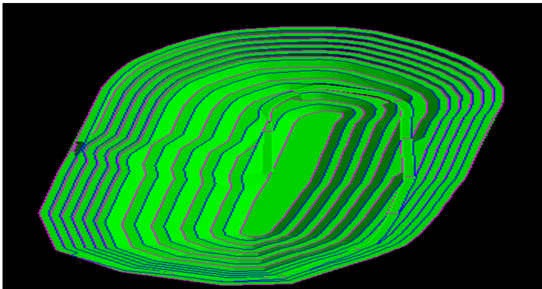
Őekil 3.32 Proje 3 boyutlu modeli.
