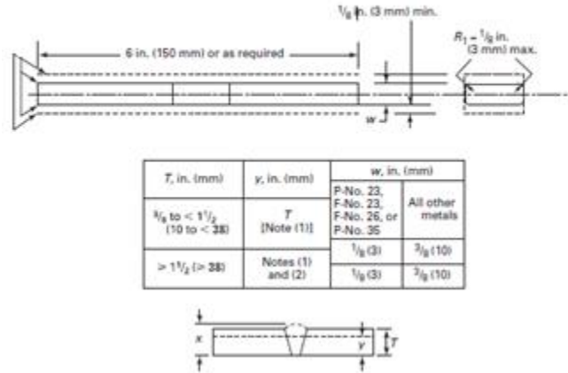
Şekil 3.12 Eğme Testi Hazırlama Ölçüleri.
