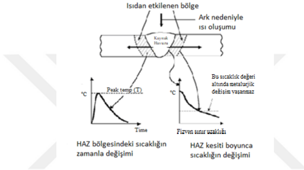
Şekil 2.11 Isı Tesiri Altında Kalan Bölge (ITAB) (İnt.Kay.2).
