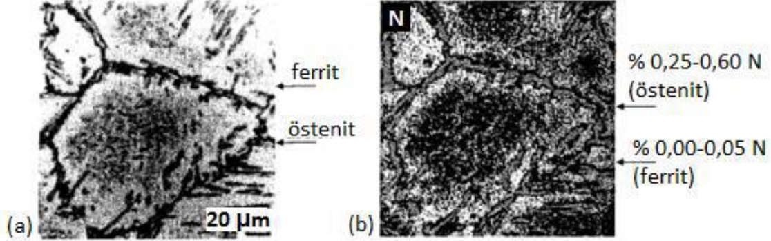
Resim 2.8 Düşük Azot İçerikli 2205 Alaşımının Kaynağında Oluşan Ergimiş Bölge; a) Ergimiş Bölgenin Mikroyapısı, b) %N Dağılımı; Aydınlık Kontrastlı Alanlar: % 0,00-0,05 N, Siyah ve Gri Alanlar: % 0,05-0,25 N, Koyu Kontrastlı Alanlar: % 0,25-0,60 N (Ogawa and Koseki 1989).
