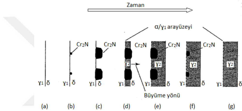
Şekil 2.16 İkincil Östenitin Oluşum Mekanizması (Ramirez et al. 2003).
