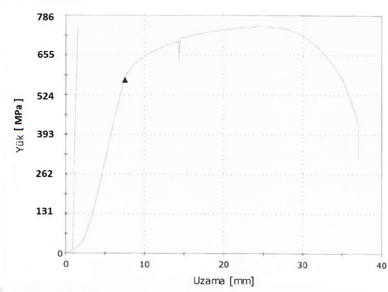
Resim 4.14 Birinci Numune Ait Yük Uzama Grafiđi.
