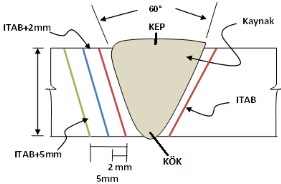
Şekil 3.8 P.T.S 20.191 Standardına Göre Test Yapılacak Bölgeler.
