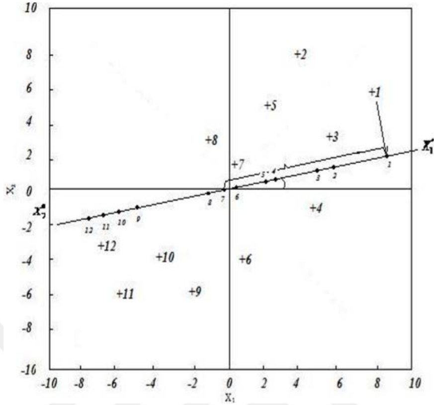
Şekil 2.2. Ortalamaya Göre Düzeltilmiş Birimlerin Değerlerinin X_1^* Eksenindeki İz Düşümleri
