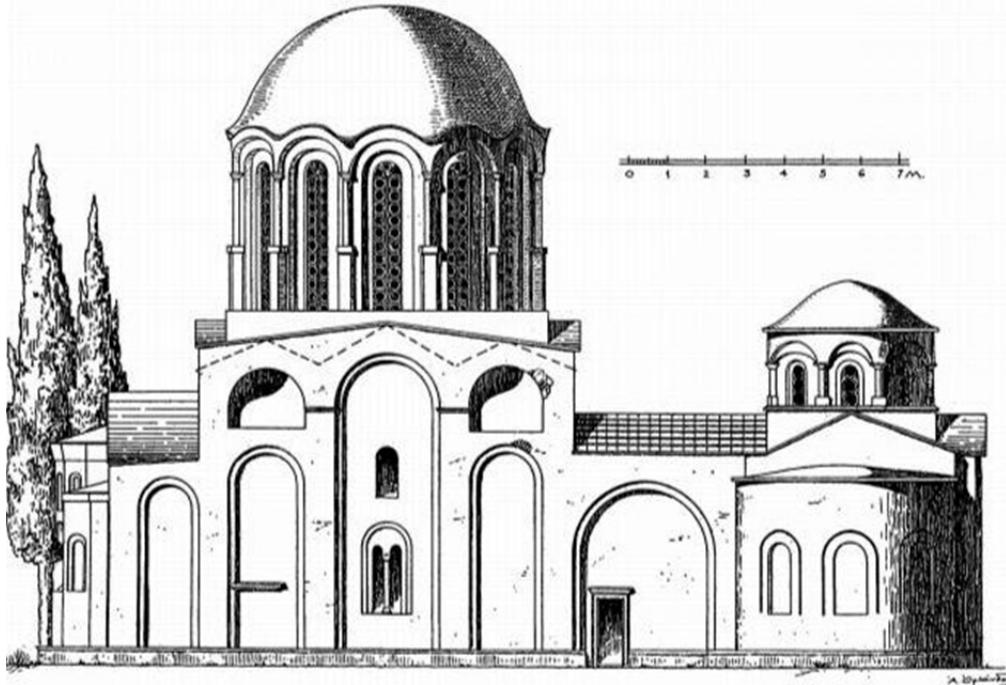
Çizim 3: Nea Moni Theotokos Kilisesi, Batı Cephesi (Ousterhout 1992: 51).
