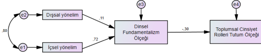
Şekil 3. Yapısal Eşitlik Modeline İlişkin Yol Diyagramı
