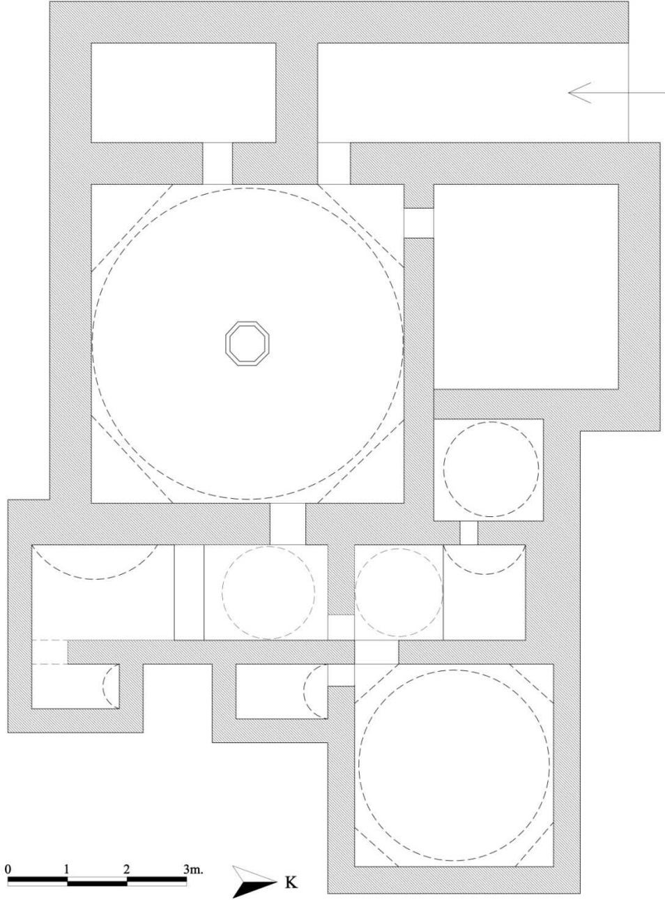
Şekil 1: Erzurum Küçük Hamam Plânı (S. Çınar'dan düzeltilerek).
