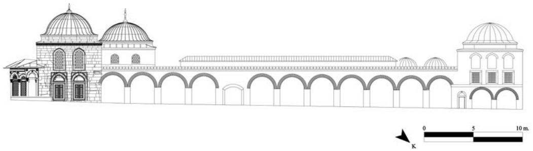
Şekil 13: Murad Paşa Külliyesi Kuzeydoğu Cephe Çizimi (İ4NKVKBK).
