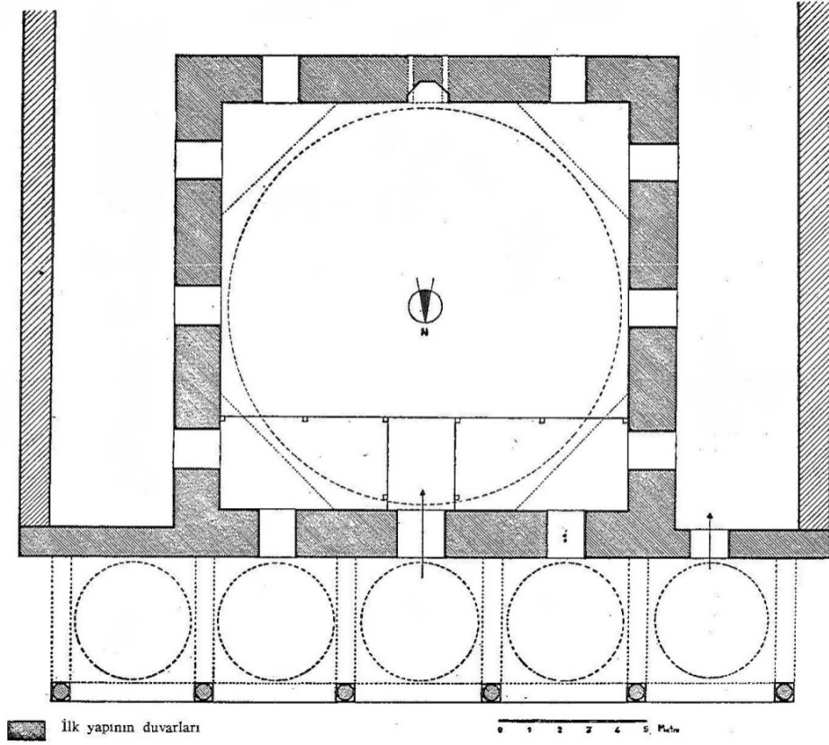
Şekil 7: Erzurum Murad Paşa Cami Plân ( R. Hüseyin. Ünal).
