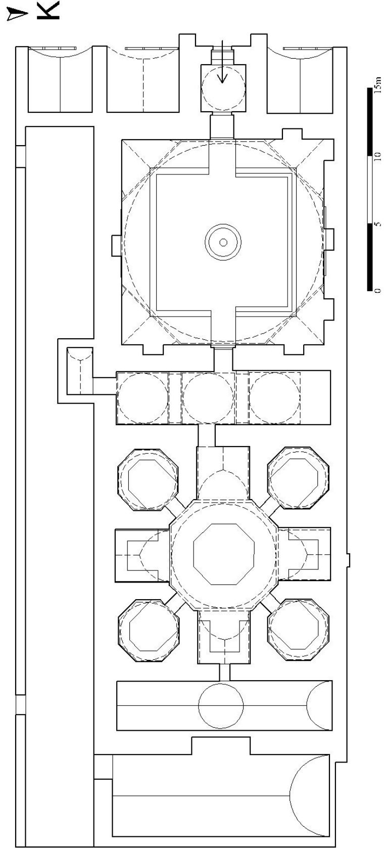
Şekil 3: Murad Paşa Hamamı Plân (S. Çınar).
