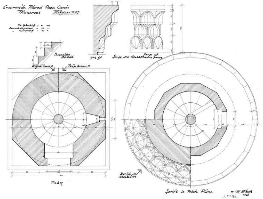
Şekil 9: Murad Paşa Cami Minaresi Plân-Kesit-Detay (VGM).
