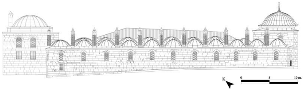
Şekil 14: Murad Paşa Külliyesi Güneybatı Cephe Çizimi (İ4NKVKBK).
