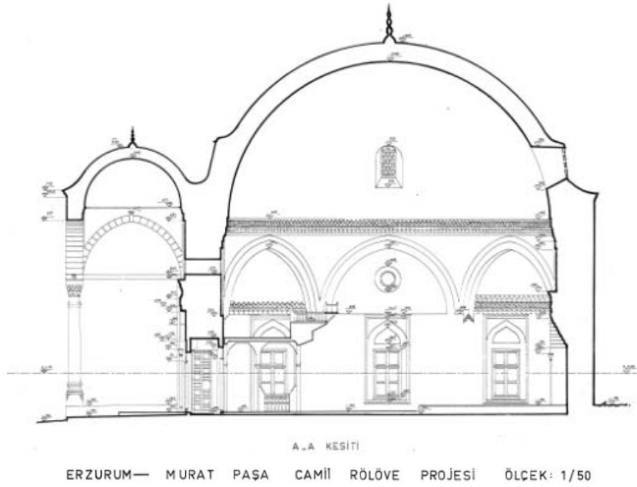
Şekil 8: Murad Paşa Cami Kesit (VGM).
