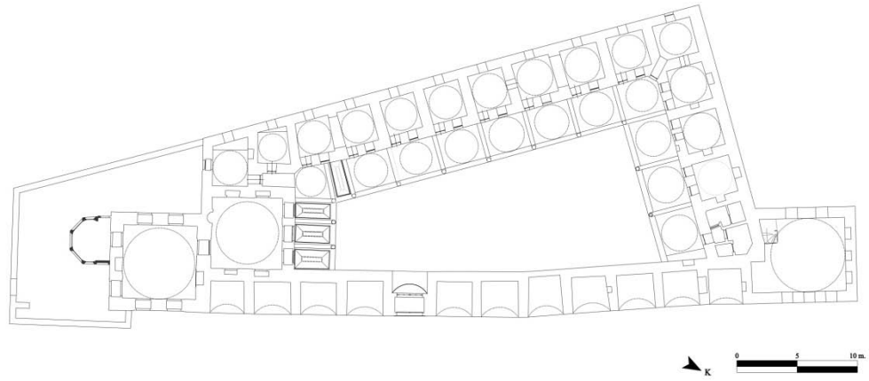
Şekil 12: Murad Paşa Külliyesi (Sıbyan Mektebi) İkinci Kat Planı (İ4NKVKBK).
