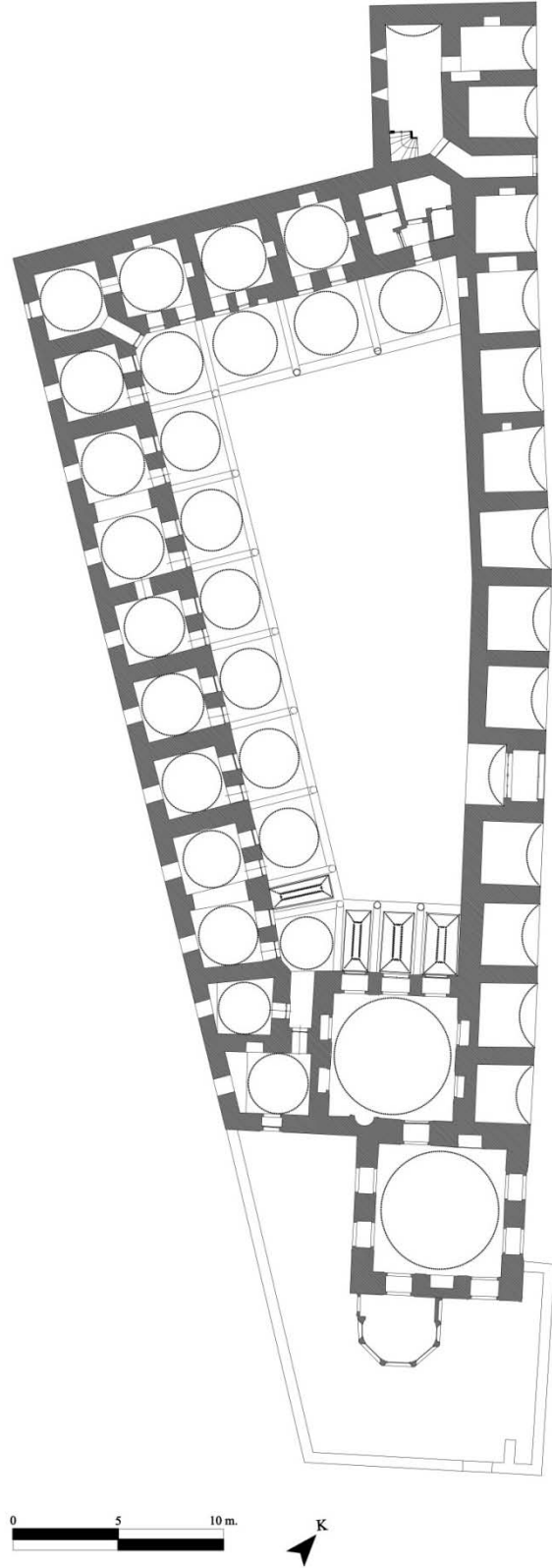
Şekil 11: İstanbul Murad Paşa (Kuyucu) Külliyesi Vaziyet Plânı (İ4NKVKBK).
