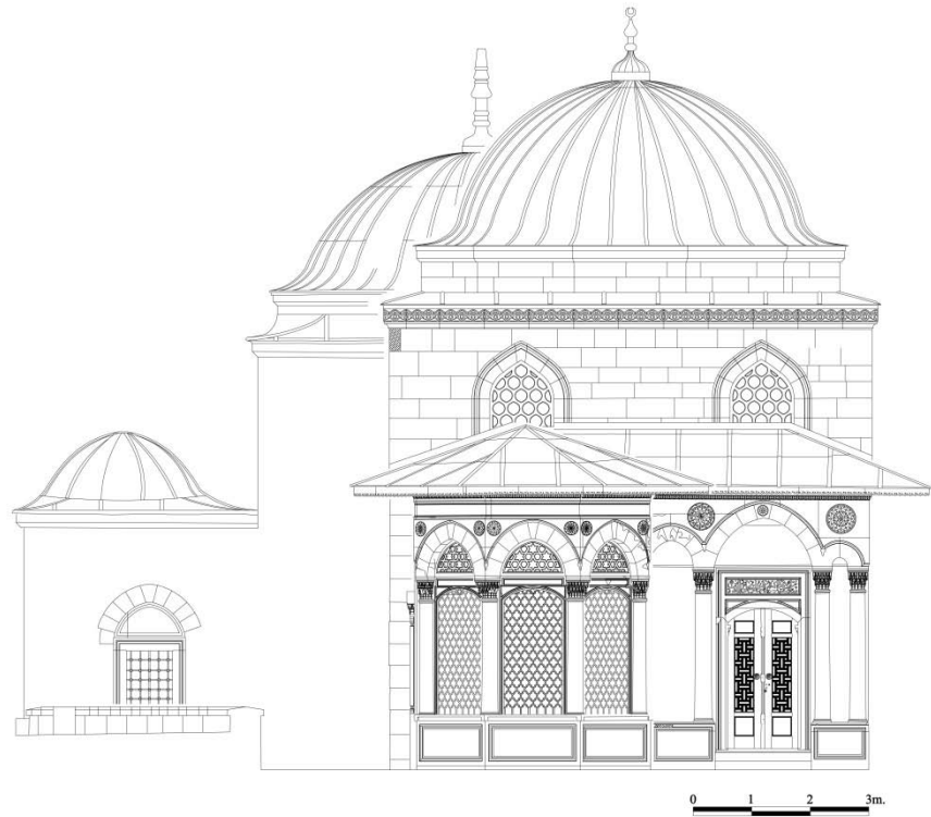
Şekil 16: Murad Paşa Külliyesi Güneydoğu Cephe Çizimi (İ4NKVKBK).
