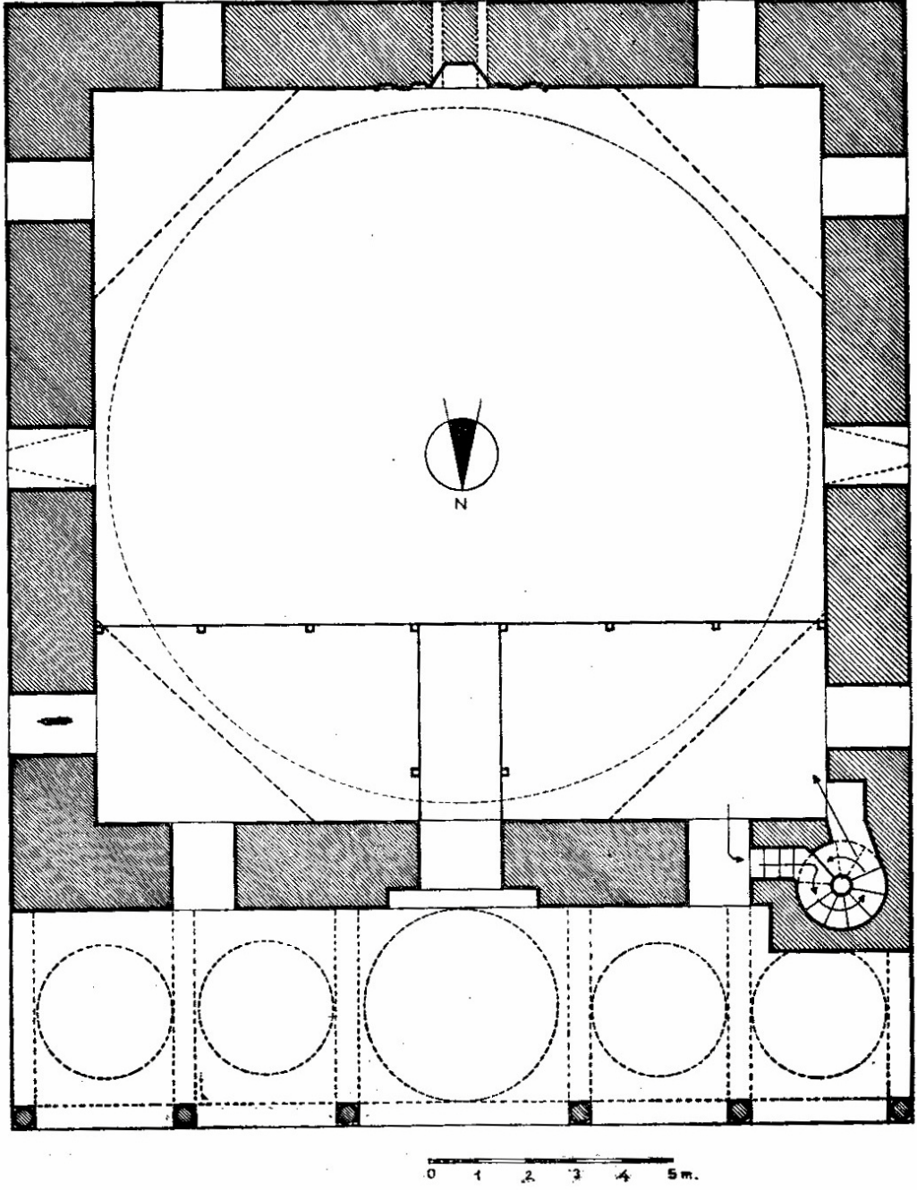
Şekil 10: Erzurum Narmanlı Camii (R. Hüseyin Ünal).
