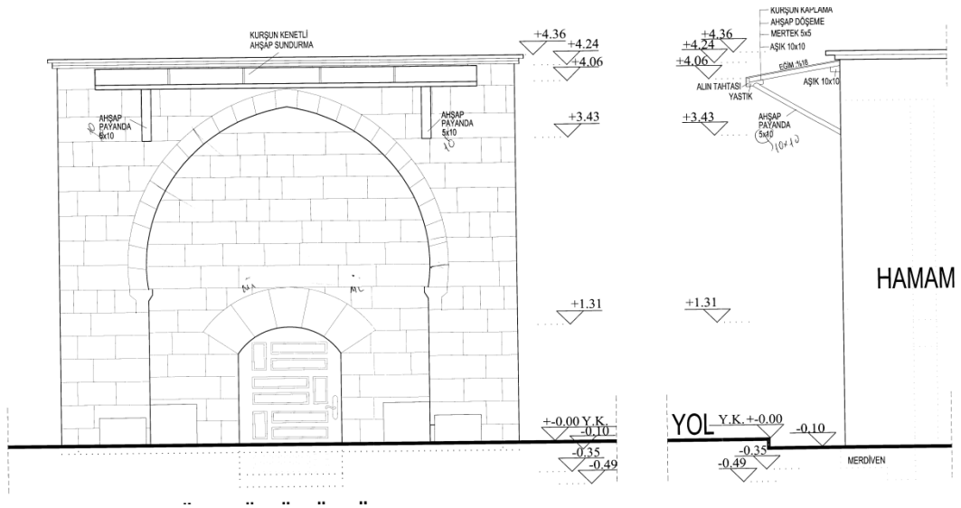
Ön Cephe Ö: 1/50
