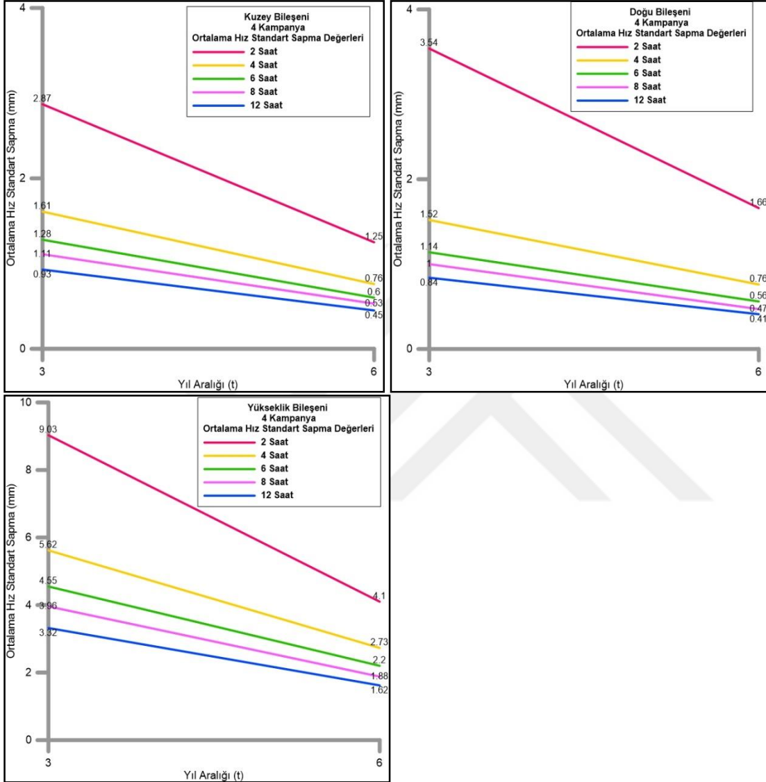
Şekil 5.14 2-12 saat aralıklarında 4 kampanya doğu, kuzey ve yükseklik bileşenleri ortalama hız standart sapma değerleri.
