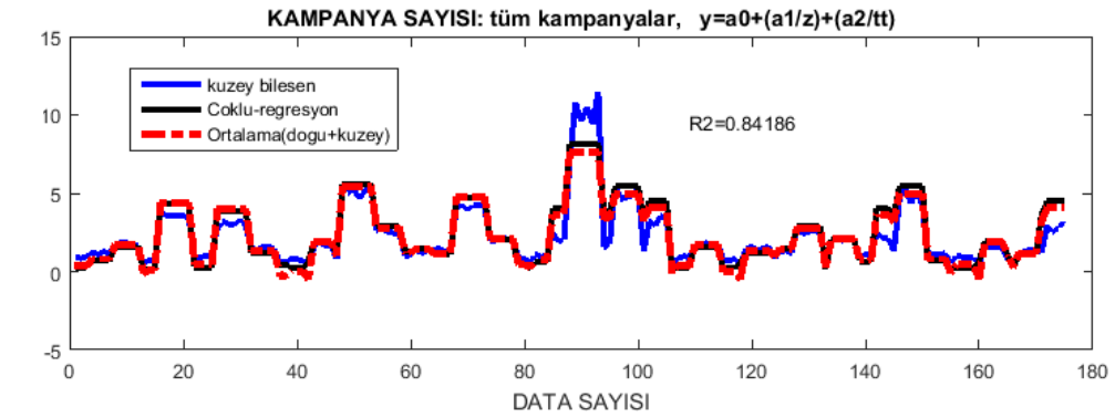
Şekil 5.23 2 parametrelı fonksiyon tüm kampanya sayısındaki verilerden elde edilen çoklu regresyon analizi grafiđi.
