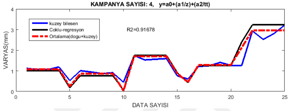
Şekil 5.22 2 parametrelı fonksiyon 4 kampanya verilerden elde edilen çoklu regresyon analizi grafiđi.
