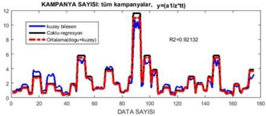
Şekil 5.31 2 parametrelı fonksiyon tüm kampanya sayısındaki verilerden elde edilen çoklu regresyon analizi grafiđi.
