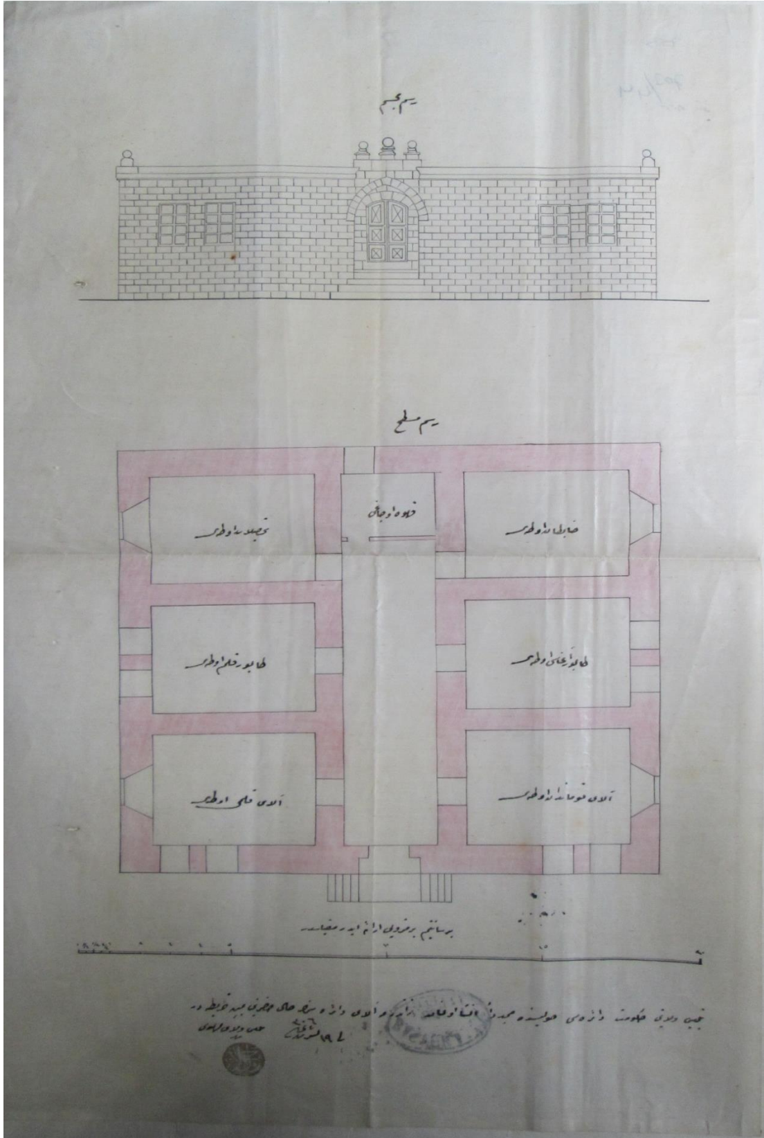
Ek 21 - BOA. ZB. 703/44 19 Şu 1306 (3 Mart 1891) Bitlis Hükümet Dairesi avlusunda yeniden inşa olunan Zabita Dairesi'nin Projesi.
