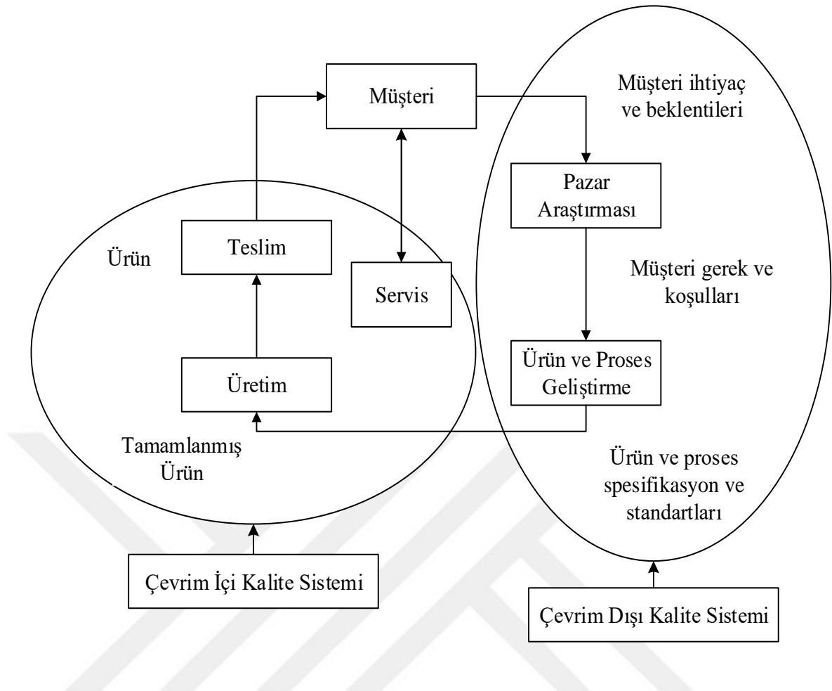
Şekil 2. 6. Çevrim içi ve çevrim dışı kalite kontrol sistemi kapsamı (Şirvancı, 1997: 14)
