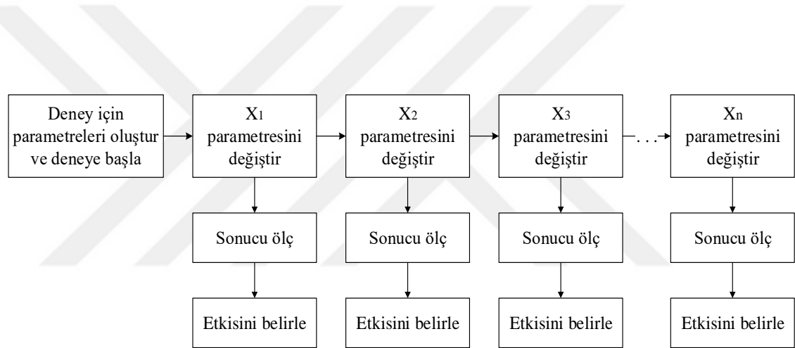
Şekil 2. 4. Geleneksel metodoloji ile yapılan deney tasarımı ve ölçümü (Gökçe ve Taşgetiren, 2009:74)
