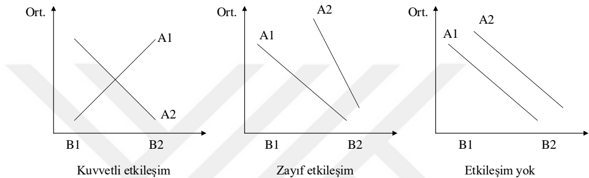
Şekil 2. 12. İki faktör arasındaki etkileşim grafikleri
