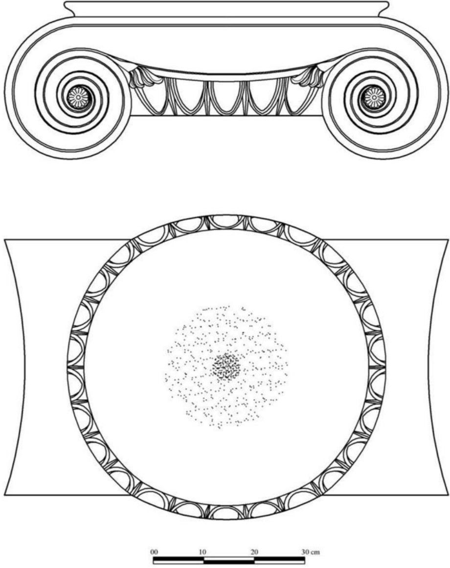
Çizim 25-26: Başlıgın Restitüsyon Çizimi (Kat. Nr. 1)
