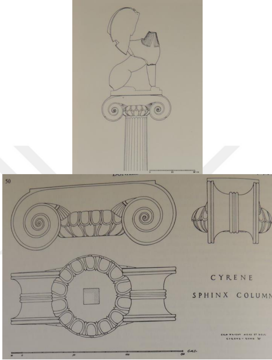
Çizim 10-13: Kyrene Sphenksli Sütunu
