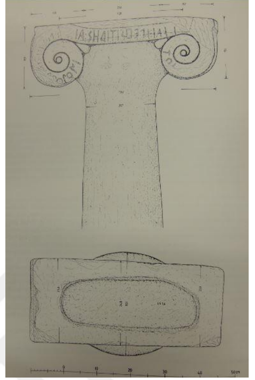
Çizim 6: Sangri Adak Sütunu Çizimi
