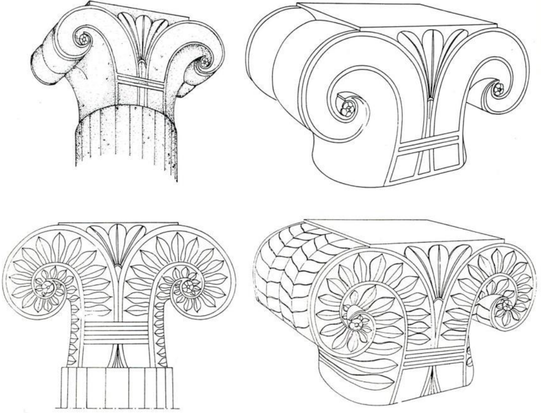
Çizim 1-4: Smyrna Athena Tapınağı Aiol Başlıkları
