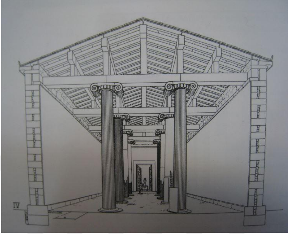
Çizim 8: Naksos Adasındaki Yria Apollon Tapınağı IV. Evre
