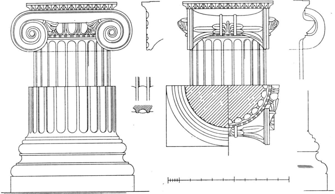
Çizim 36: Magnesia Propylonu
