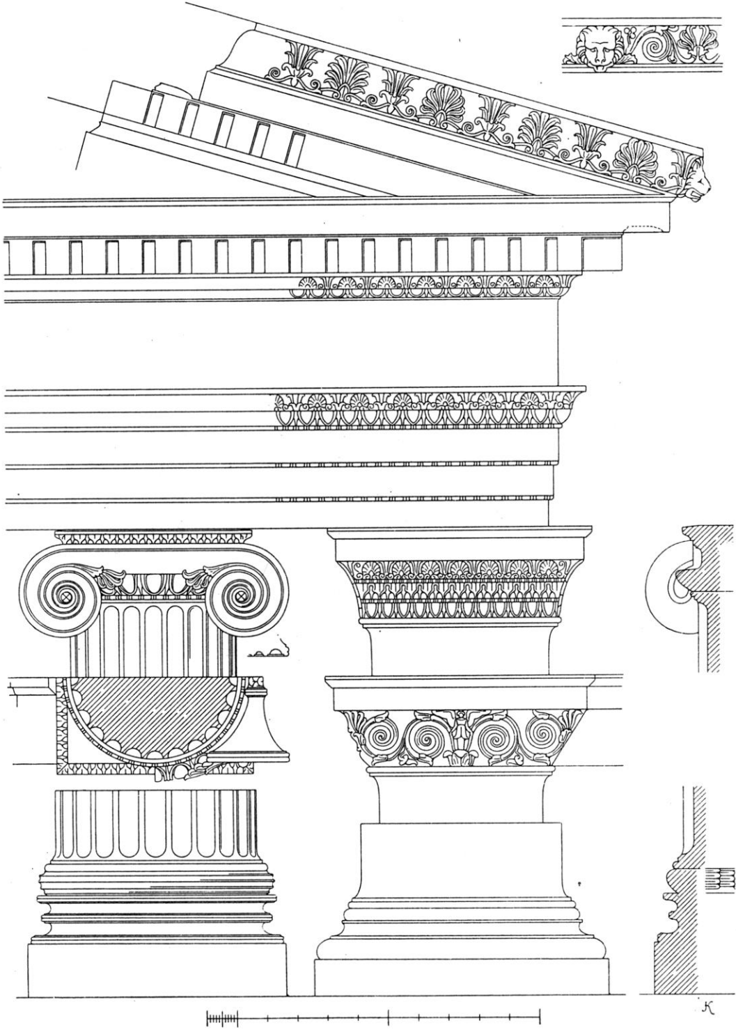
Çizim 38: Magnesia Zeus Tapınağı Kesit ve Görünüş
