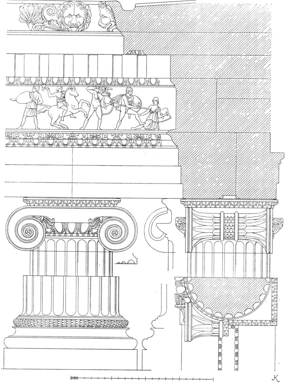
Çizim 37: Magnesia Artemis Tapınağı Kesit ve Görünüş
