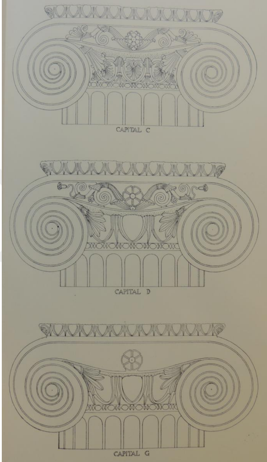
Çizim 32-34: Sardeis Artemis Tapınağı Başlıkları (C,D,G)
