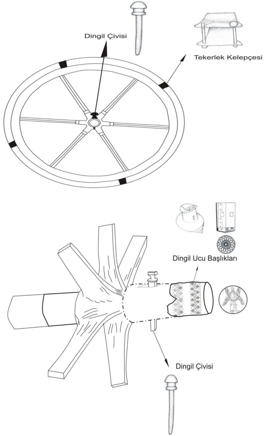
Resim 23: Araba Tekerleđi ve Dingili (Gökçe, 2011: 473)
