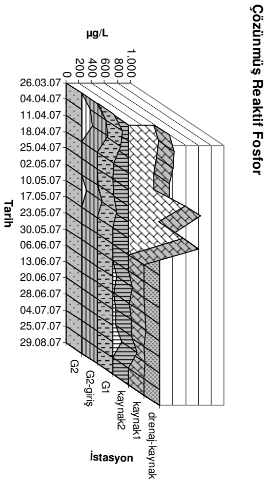
Şekil 3.1.1. Kimyasal değişkenlerin zamana bağlı değişimleri
