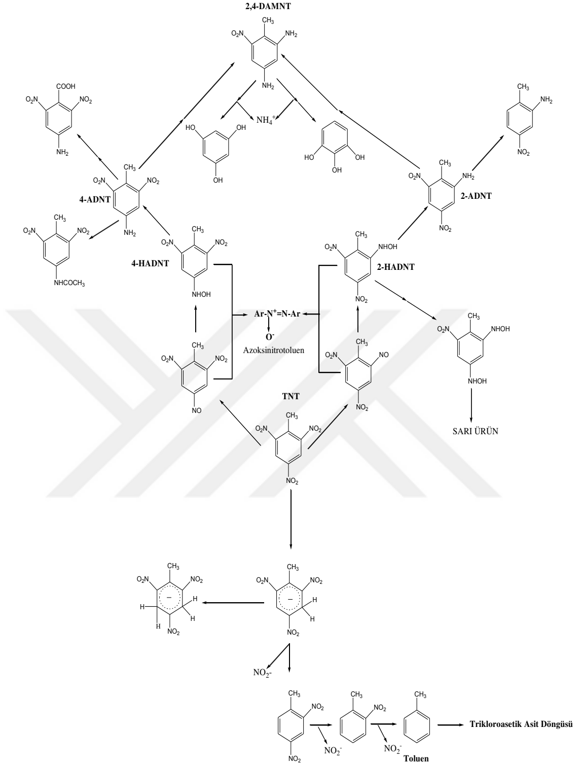
Şekil 1.3. Aerobik bakterilerde TNT'nin parçalanma mekanizması (Esteve-Nuñez vd., 2001'den değiştirilerek)
