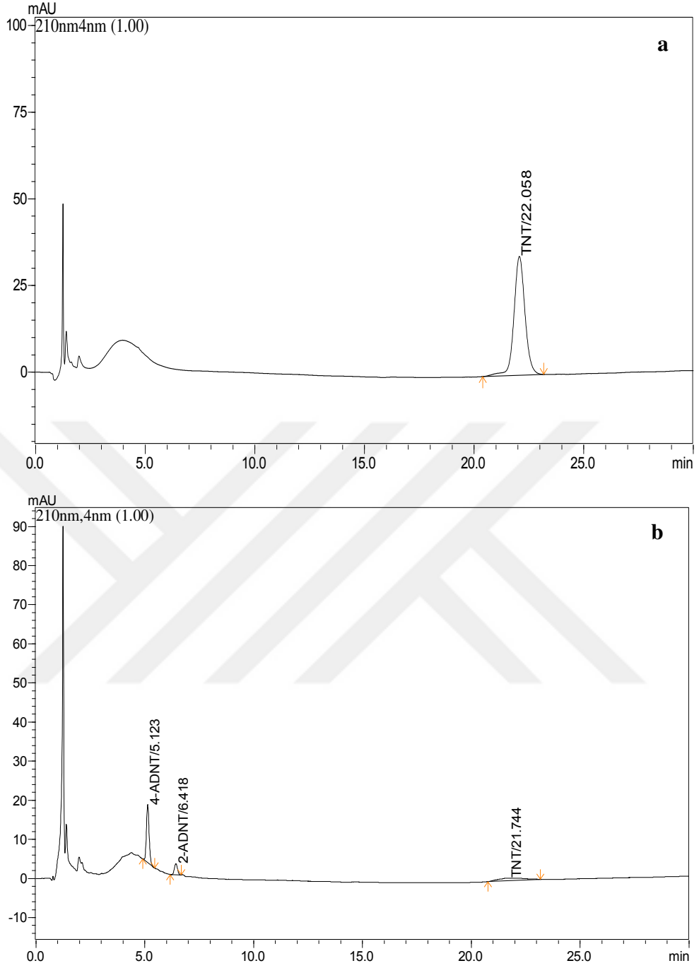
Şekil 3.10. R. planticola SU K4 izolatının (30 °C’de) 0. saatteki (a) ve 24. saatteki HPLC kromatogramları
