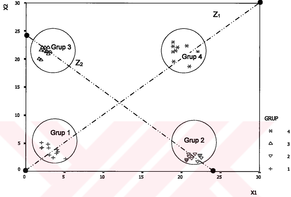
Şekil 2.28: Teorik Serpilme Diyagramı
