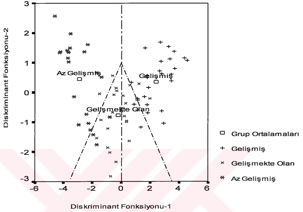
Grafik 3.16: Gelişmişlik Gruplarının Serpilme Diyagramı (1995-02)
