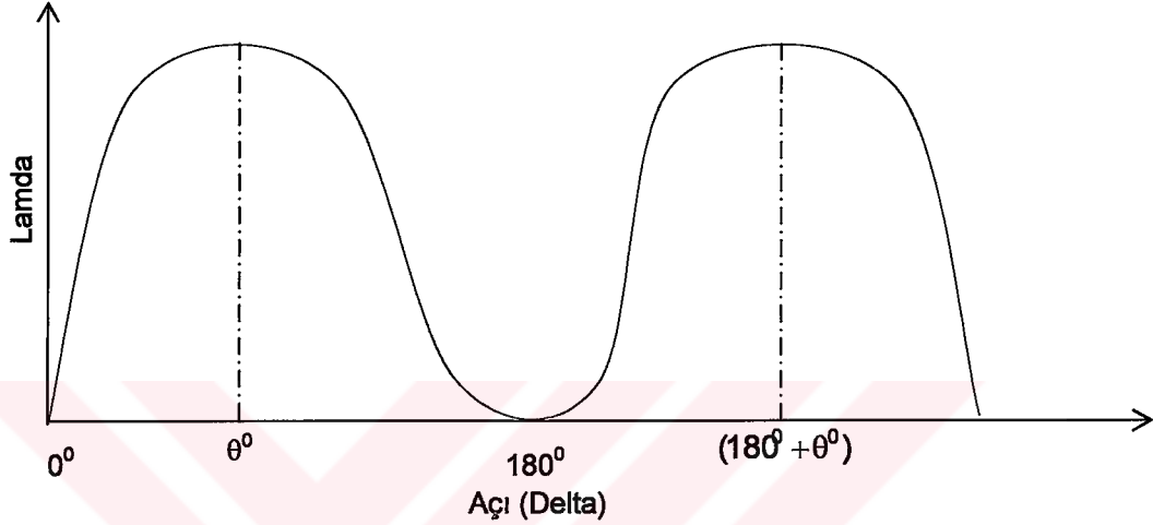
Şekil 2.25: Lamda Değerleri ile Delta Açıları
