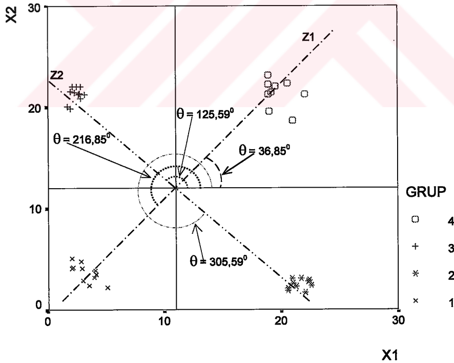
Şekil 2.29: Dört Gruplu ve İki Fonksiyonlu Verilerin Grafiği
