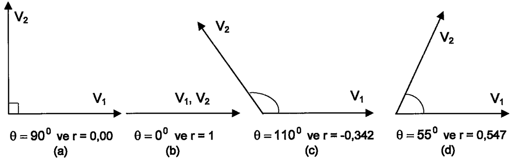
Şekil 2.11: Korelasyon Katsayılarının Açılı ve Vektörlerle Gösterilmesi
