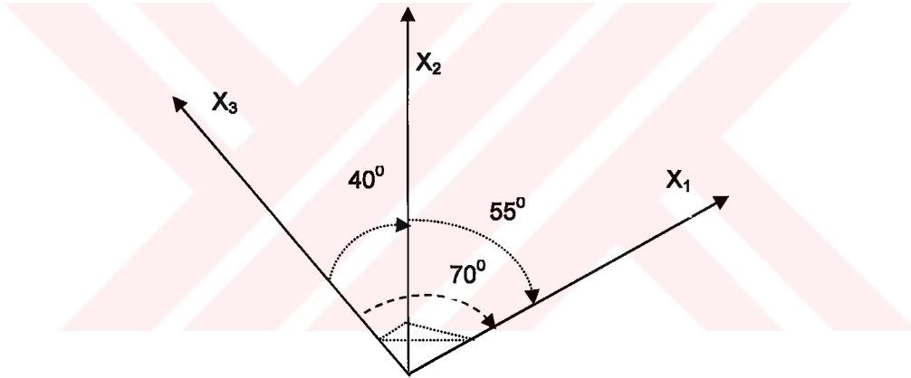
Şekil 2.12: Üç Boyutlu Bir Korelasyon Matrisinin Vektörlerle Gösterilişi
