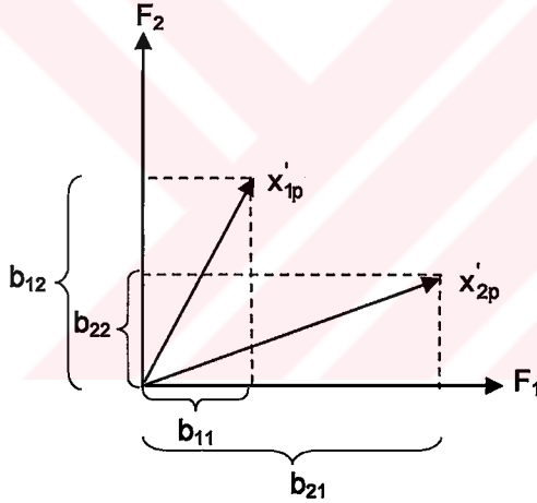
Şekil 2.20: İki Boyutlu Alt Faktör Uzayında Vektörlerin İzdüşümü
