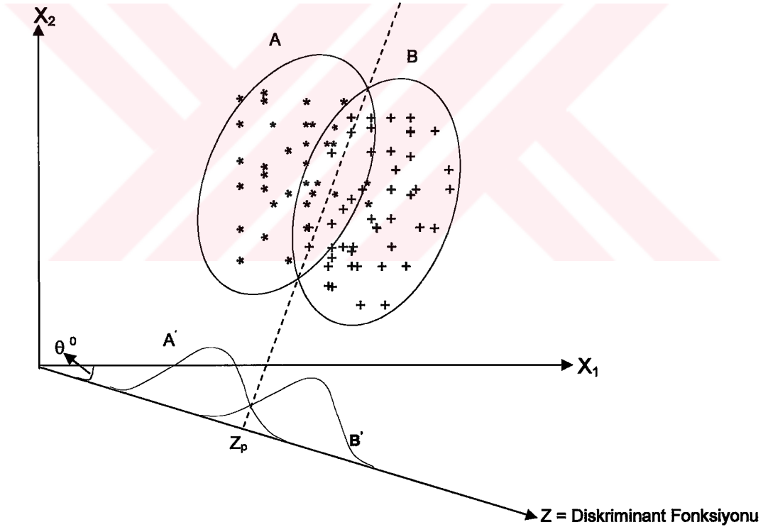
Şekil 2.22: İki Gruplu Diskriminant Analizinin Grafik Gösterimi
