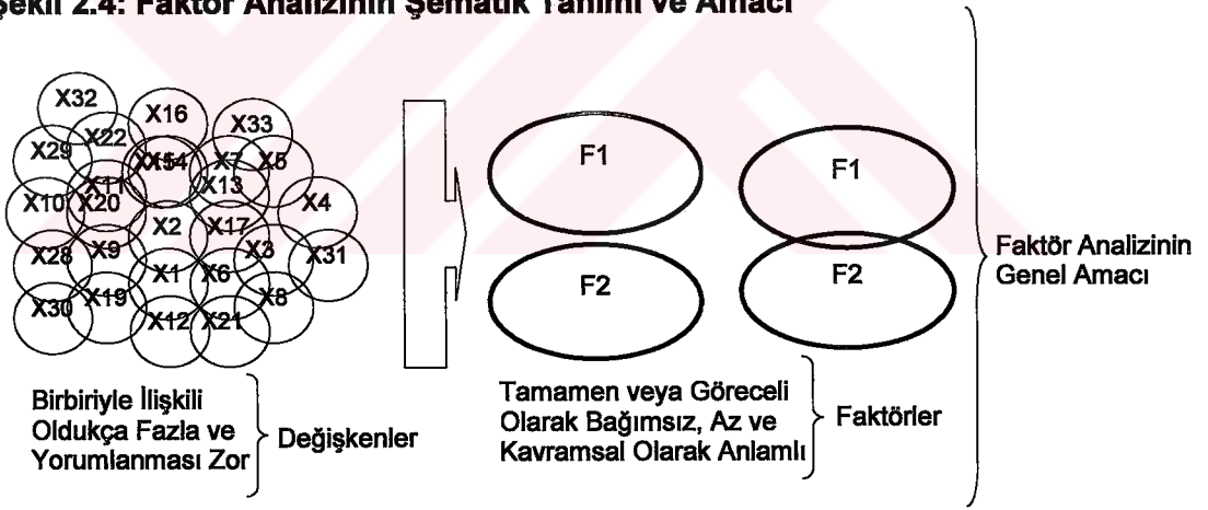
Şekil 2.4: Faktör Analizinin Şematik Tanımı ve Amacı 100
