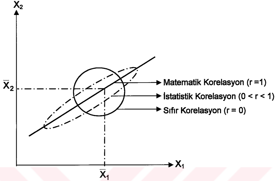
Şekil 2.10: Korelasyon Katsayısının Geometrik Gösterimi
