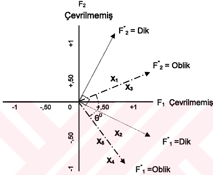
Şekil 2.17: Oblik (Eğik) Faktör Rotasyonu
