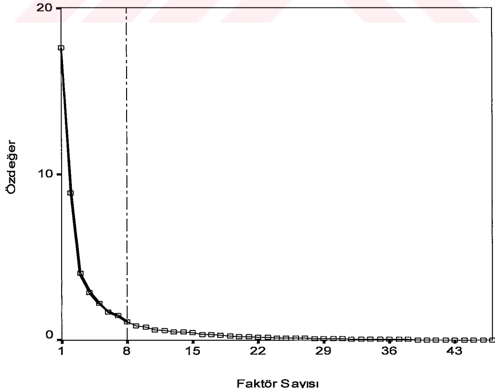
Grafik 3.2: Asal Bileşen Faktör Analizi İçin Scree Grafiği (İkinci Dönem)
