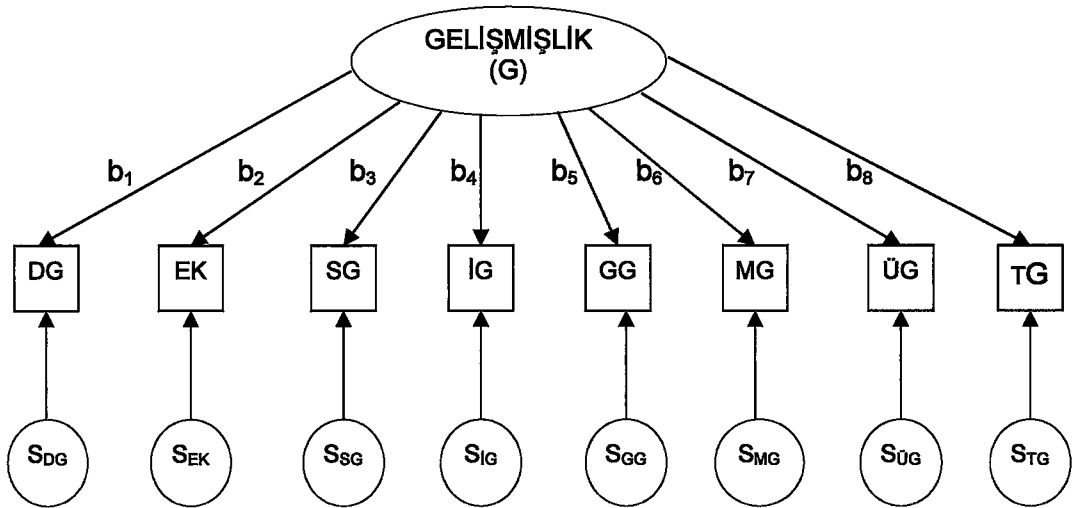
Şekil 2.5: Gelişmişlik ile Göstergeler Arasındaki İlişki (Tek-Faktörlü Model)
