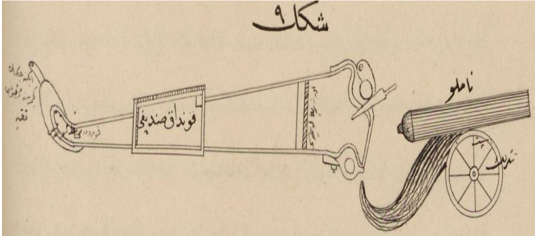
Sayfa-77 Şekil-9 9 Santimetrelık Çemberli Sahrâ Topu
