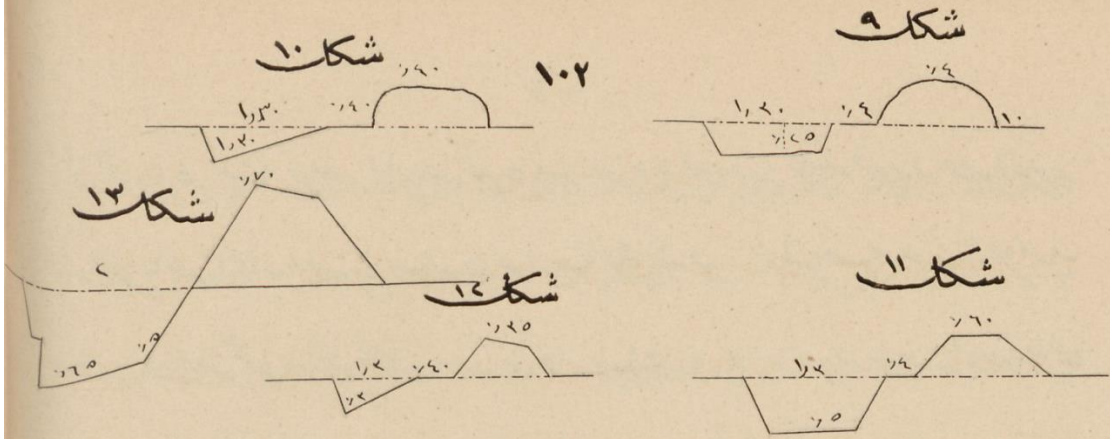
Sayfa-102 Şekil-9, 10, 10, 11 ve 12 Hafr-İmla Hacimleri Müsavi ve en Ziyade Müstamel Maktalar
