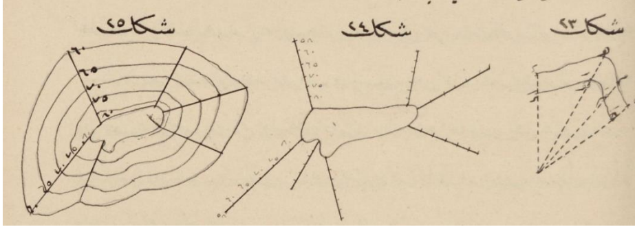
Sayfa-53 Şekiller 23, 24 ve 25 Tesviye Ameliyatı Yani kabarmaların Beyanı
