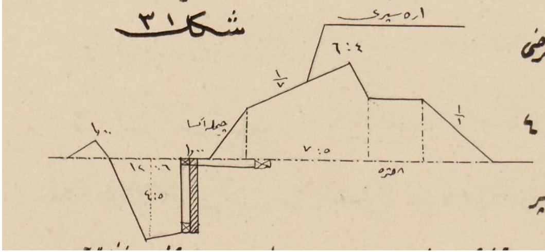
Sayfa-133 Şekil-31 Topçuya Mahsus Omuz Siperi
