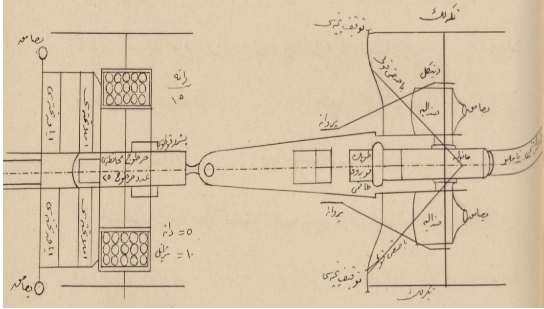
Sayfa-78 Şekil-10 9 Santimetrelik Muhasara Topunun Top yuvarlağ
