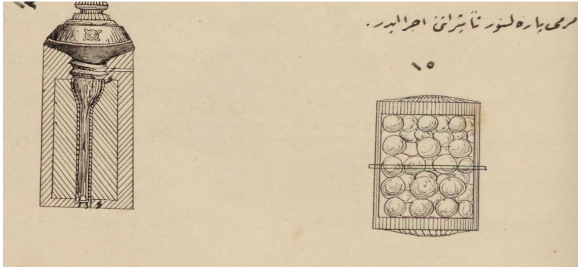
Sayfa-79 Şekil-13 ve 14 Eslihâ-yı Nariyye-i Sakileye Mahsus Mermi Sayfa-80 Şekil-14 Şarapnele Mahsus Tıpa
