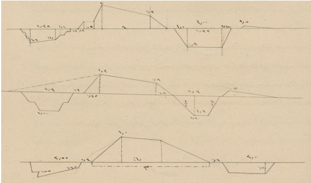
Sayfa-101 Şekil-5, 6 ve 7 Hafr-İmla Hacimleri Müsavi ve en Ziyade Müstamel Maktalar
