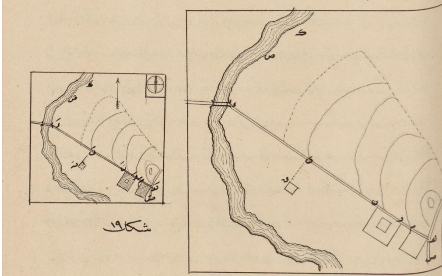
Sayfa-46 Şekil-19 Yol Haritasının Ahzı
