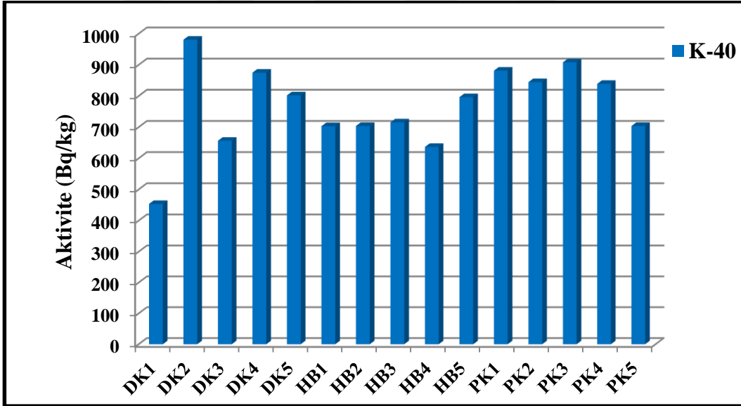
Şekil 4.5: Toprak örneklerindeki ^{40}\text{K} konsantrasyonu.
