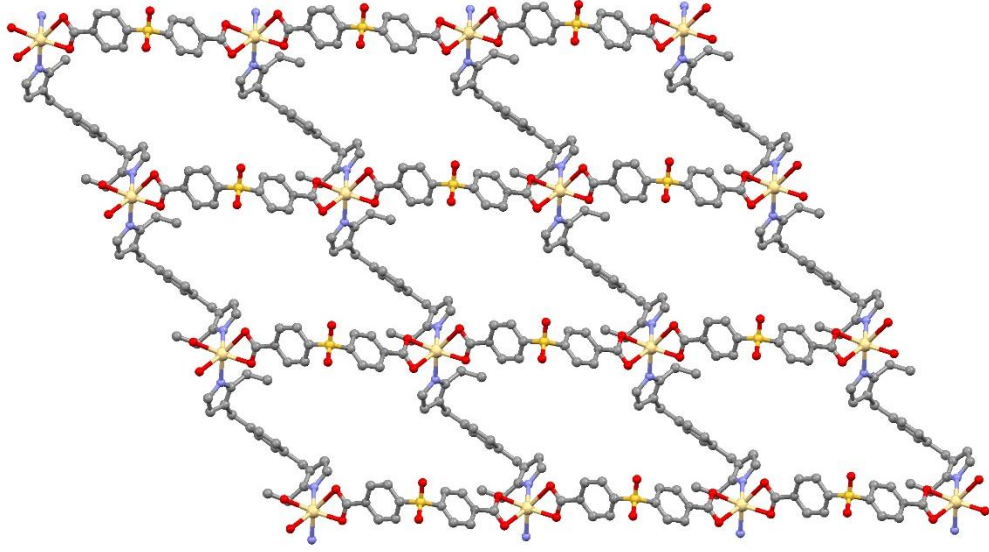
Şekil 4.4: [\text{Cd}(\text{sdba})(\text{pbetix})]_n ( 1 )'un iki boyutlu yapısı.
