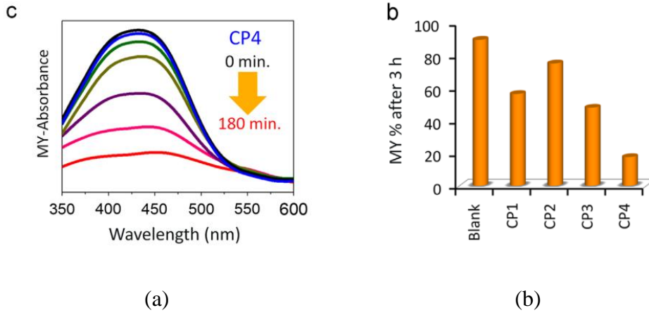
Şekil 2.3: (a) Co(II)-kompleksinin boya gideriminin UV/Vis spektroskopisinden takip edilmesi ve (b) tüm komplekslerin fotokatalitik boya giderim performansları (Bisht ve diğ, 2014).
