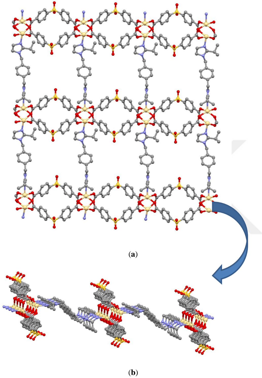
Şekil 4.8: [\text{Cd}_2(\text{sdba})_2(\text{pbisobix})] \cdot 2\text{H}_2\text{O} ( 2 )'nin (a) ve (b) iki boyutlu yapısı.
