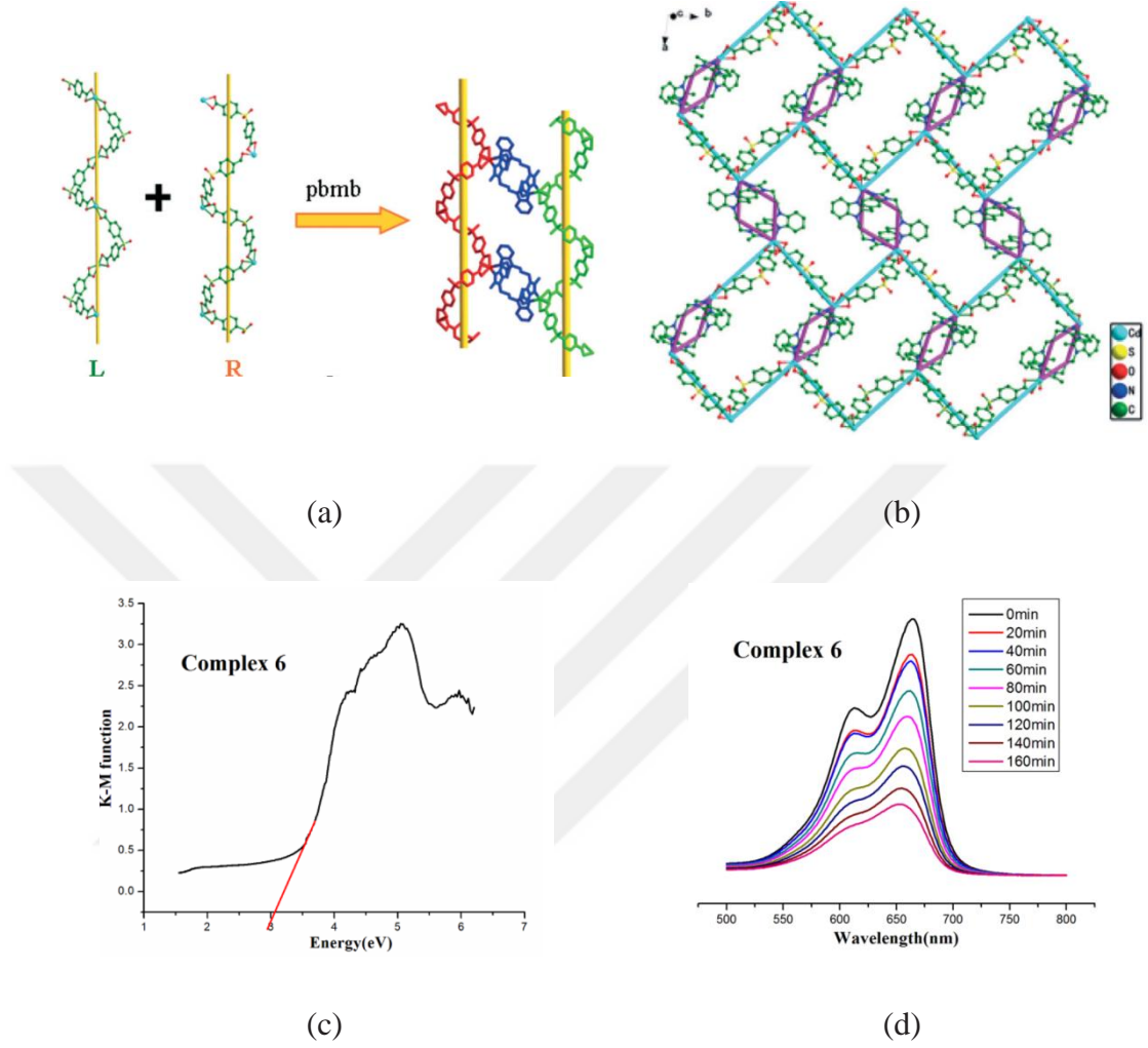
Şekil 2.8: (a) \{[Cd(sdba)(pbmb)] \cdot 2H_2O\}_n kompleksinin 1D sarmal zincirleri (b) zincirlerin birbirine bağlanmasıyla 2D yapının oluşması (c) kubelka-Munk denkleminin kullanılmasıyla kompleksin bant aralığının hesaplanması (d) kompleksin UV/Vis spektroskopisi ile MB'nin fotokatalitik bozunmasının takip edilmesi (Ming Li ve diğ., 2014).
