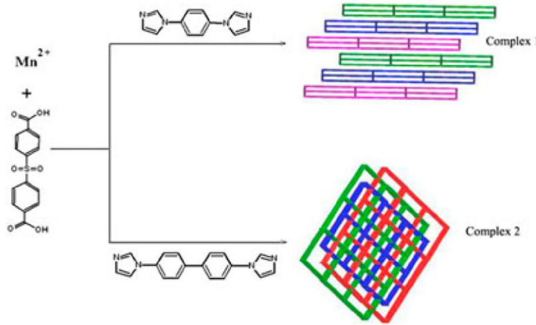
Şekil 2.12: {[Mn(sdba)(L15) 0.5 ]·0,5(L15)} n ve [Mn(sdba)(L16)] n komplekslerinin yapıları (Liu, 2015).
