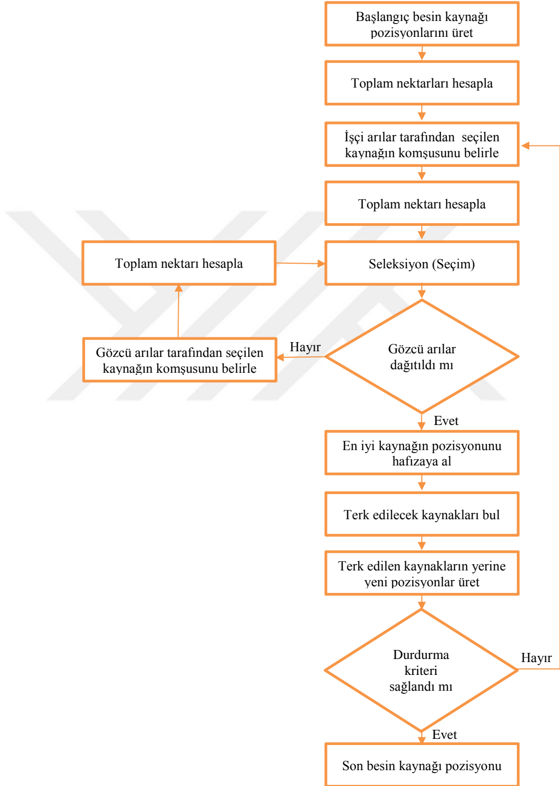
Şekil 4.7 : YAK algoritmasının akış diyagramı (Akay ve Karaboğa, 2012).
