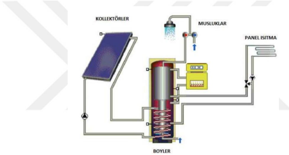
Şekil 2.5 : Düzlemsel güneş kolektörü sisteminin araçları (Url 2).
