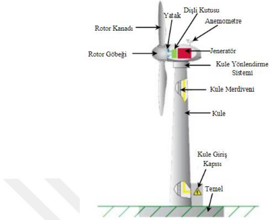
Şekil 2.14 : Yatay eksenli rüzgar türbininin yapısı (Koç ve Şenel, 2011).
