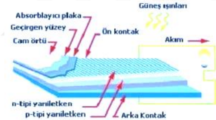
Şekil 3.3 : Fotovoltaik pil (Url 12).
