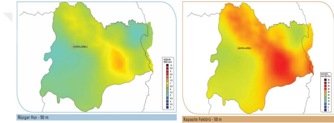
Şekil 2.13 : Kırklareline ait rüzgar hızı ve kapasite faktörü dağılımı (Url 9).
