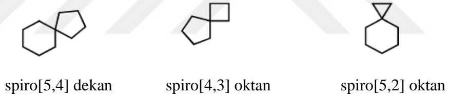
Şekil 2.1: Spiro yapıli bileşik örnekleri.
