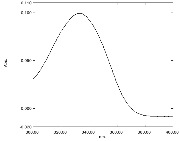
Şekil4.26: Bileşik 6'nın UV-Vis spektrumu ( 1 \times 10^{-5} M).
