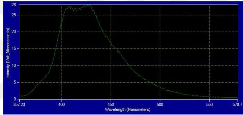
Şekil 4.47: Bileşik 10'un floresans spektrumu ( 1 \times 10^{-5} M ).
