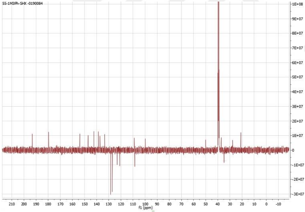
Şekil 4.30: Bileşik 6'nın 13 C (APT) NMR spektrumu.
