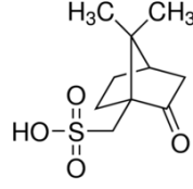
Şekil 2.3:Kamfor sülfonik asit yapısı.
