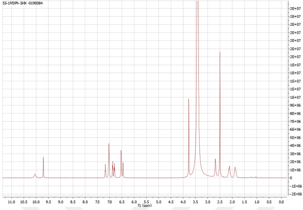
Şekil 4.29: Bileşik 6'nın 1 H NMR spektrumu.
