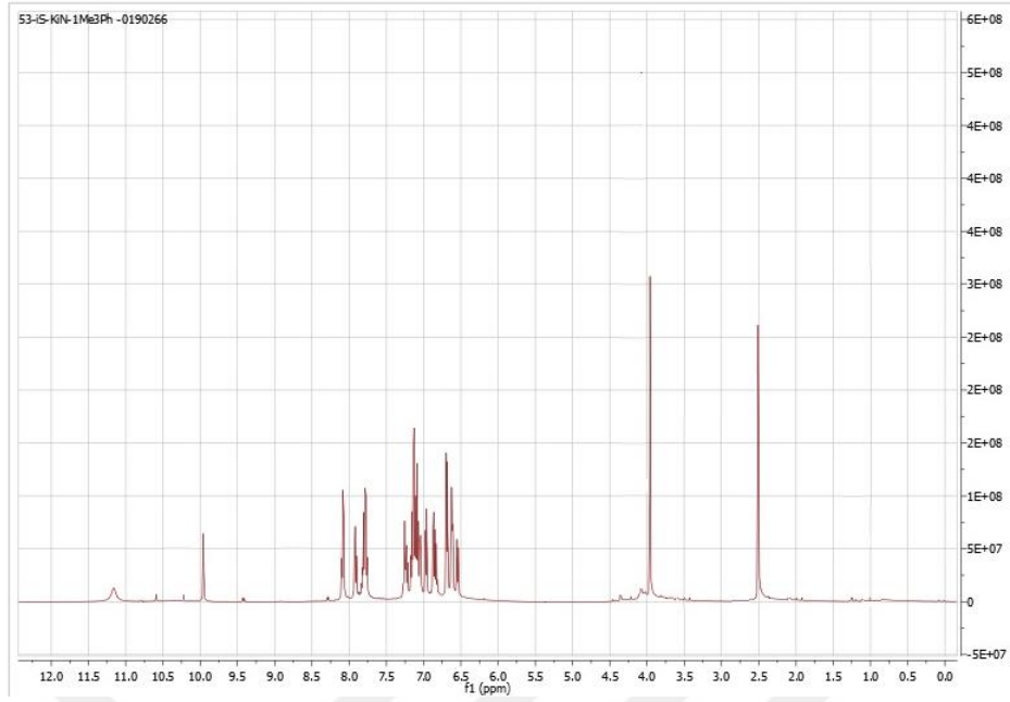
Şekil 4.44: Bileşik 9'un 1 H NMR spektrumu.
