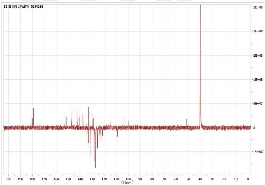
Şekil 4.45: Bileşik 9'un 13 C (APT) NMR spektrumu.
