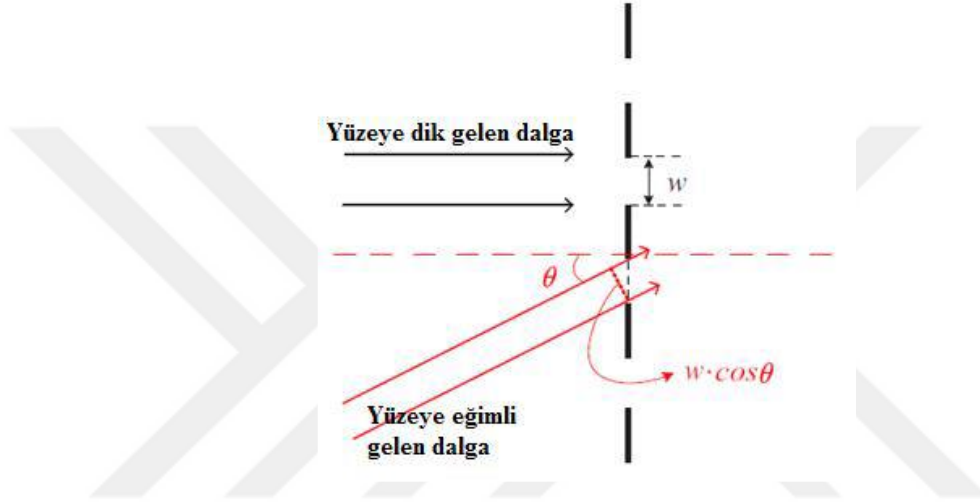
Şekil 3.16 : Elektromanyetik dalganın geliş açısına göre periyodik elemanlar arasındaki mesafenin değişimi [35].
