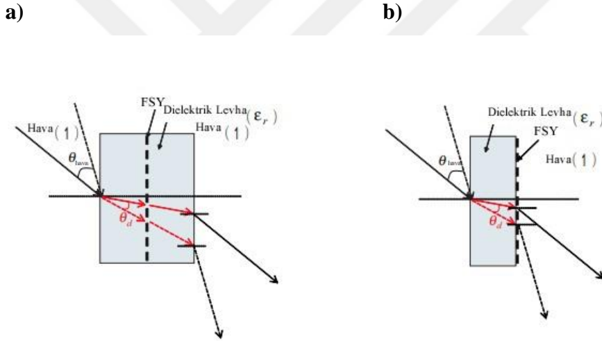
Şekil 3.15 : Dielektrik levhaların içindeki ve üzerindeki FSY (a) Dielektrik levhaların içindeki FSY, \epsilon_{eff} = \epsilon_r [12]. (b) Dielektrik levhanın üzerindeki FSY, \epsilon_{eff} = (\epsilon_r + 1)/2 [35].
