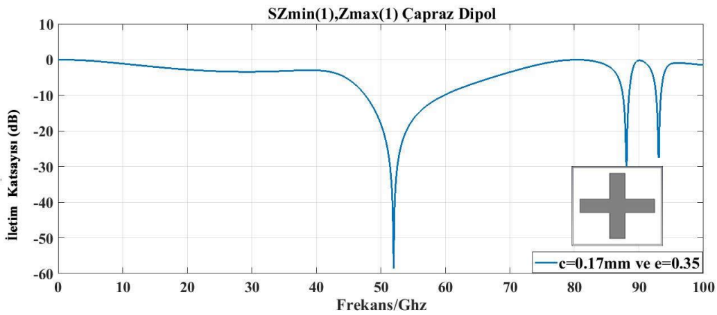
Şekil 4.5 : Çapraz dipol için iletim katsayıları [dB].
