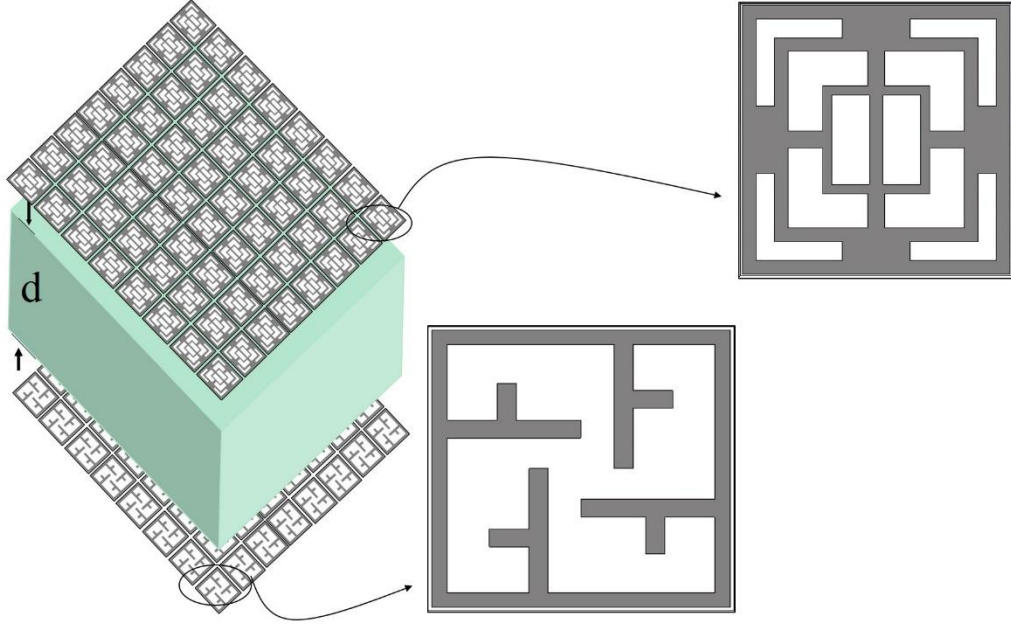
Şekil 4.13 : Ultra geniş bant frekans seçici yüzeyi oluşturan II ve F Şekillerinin birleşimi.
