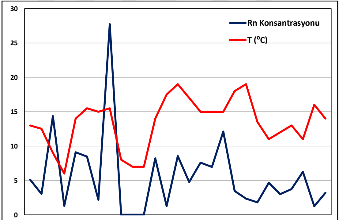
Şekil 4.67 : Kış mevsimi ^{222}\text{Rn} aktivite konsantrasyonu değerlerinin toprak sıcaklığa bağlı değişimi.
