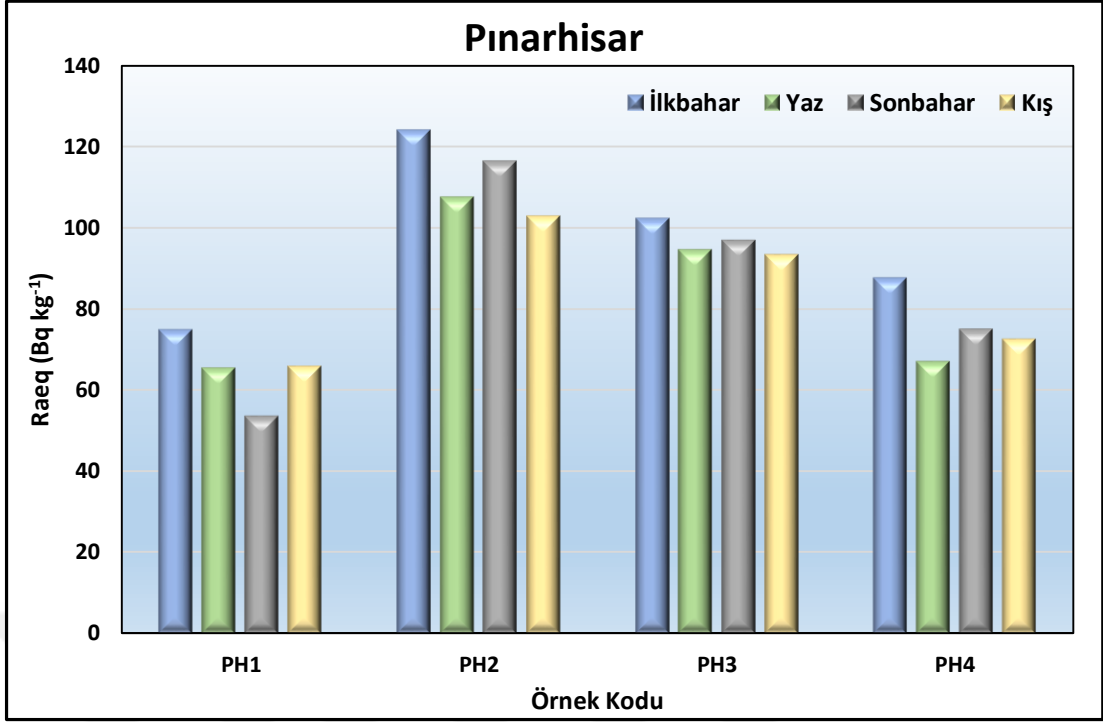
Şekil 4.42 : Kırklareli ili Pınarhisar ilçesinde mevsimlere göre radyum eşdeğer aktiviteleri.
