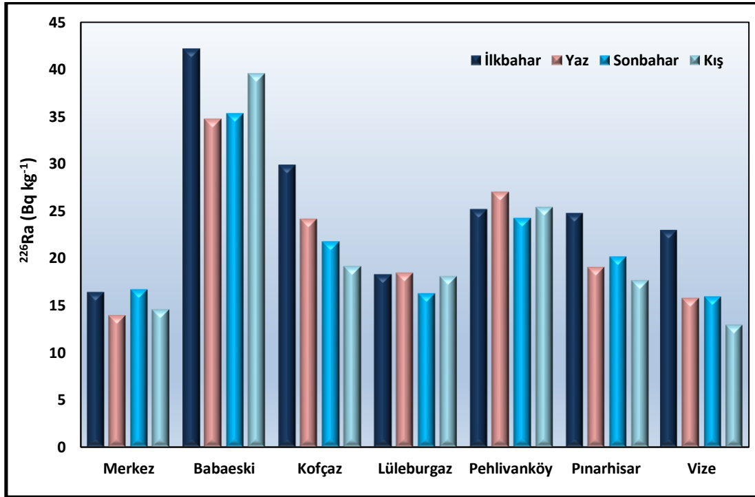
Şekil 4.17 : Ortalama 226 Ra aktivite konsantrasyonunun ilçelere göre değişimi.
