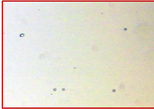
Şekil 2.18 : CR-39 dedektörü ile radon ölçümünde oluşan alfa parçacıklarının bıraktığı izlerin mikroskop görüntüsü (Banjanac, 2006).
