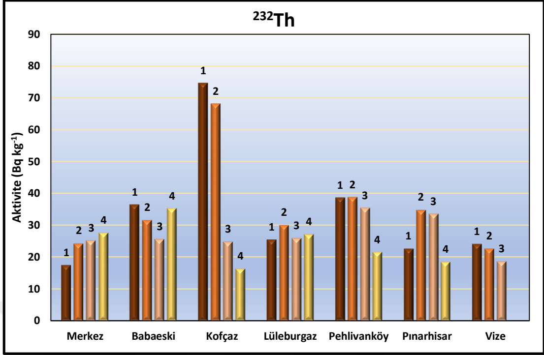
Şekil 4.14 : Kış mevsimi için toprak örneklerinin 232 Th aktivite konsantrasyonları.
