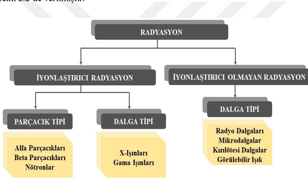
Şekil 2.2 : Radyasyon çeşitleri.
