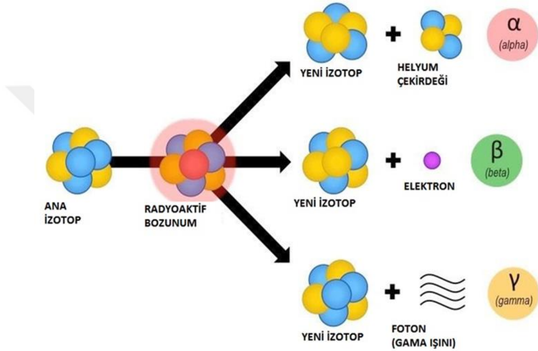
Şekil 2.6 : Radyoaktif bozunum türleri.
