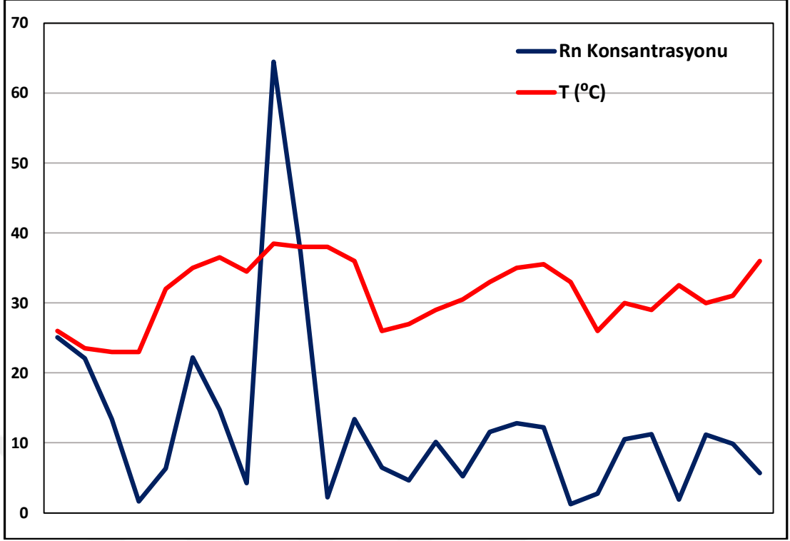
Şekil 4.66 : Yaz mevsimi ^{222}\text{Rn} aktivite konsantrasyonu değerlerinin toprak sıcaklığa bağlı değişimi.
