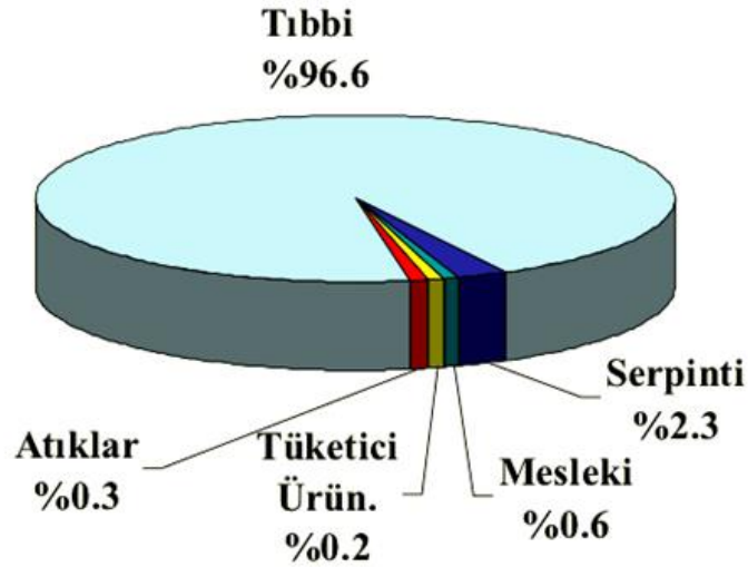
Şekil 2.22 : Dünya genelinde yapay radyasyon kaynaklarından maruz kalınan ortalama radyasyon doz oranları (Url-4).
