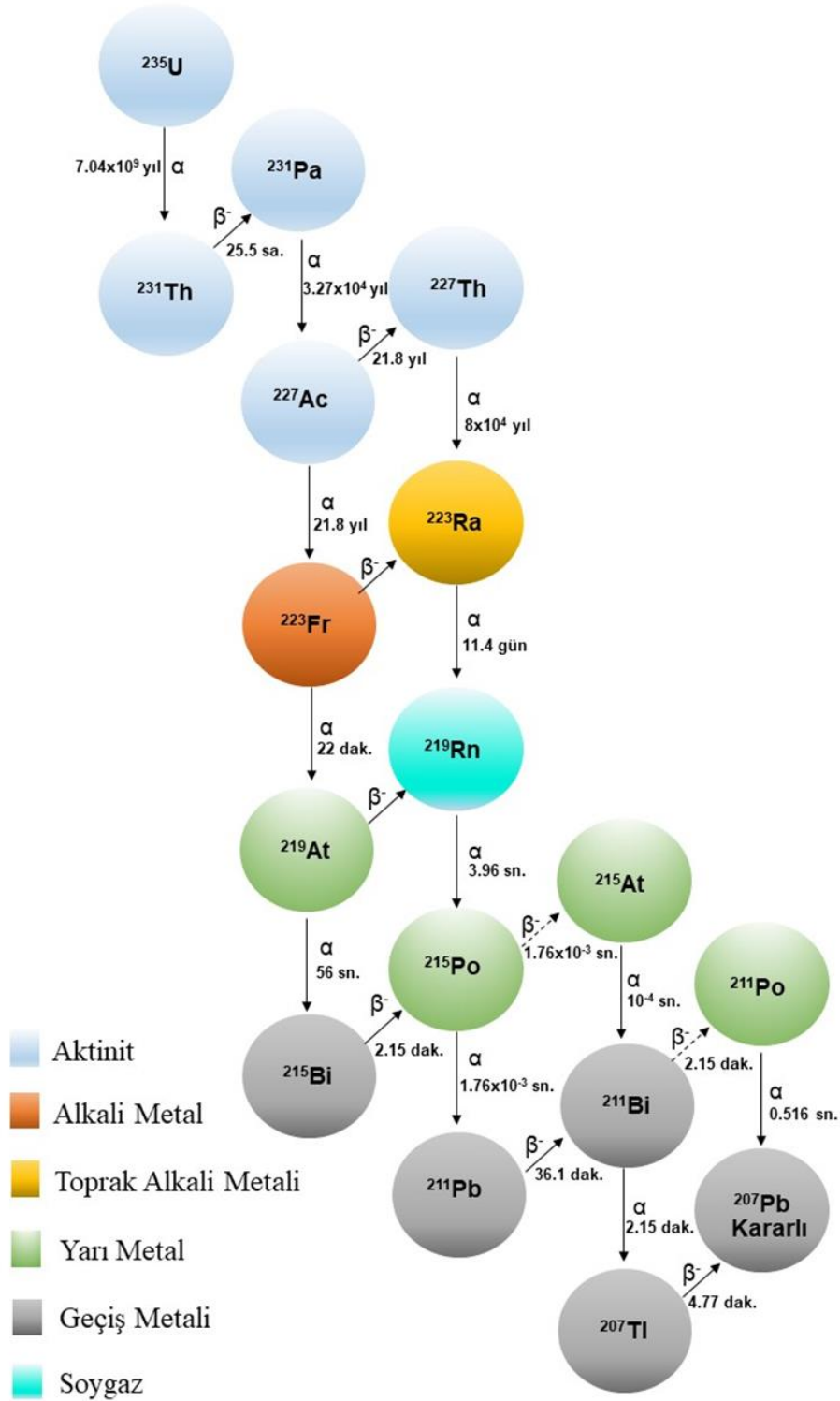
Şekil 2.9 : Aktinyum bozunma ürünleri şeması.
