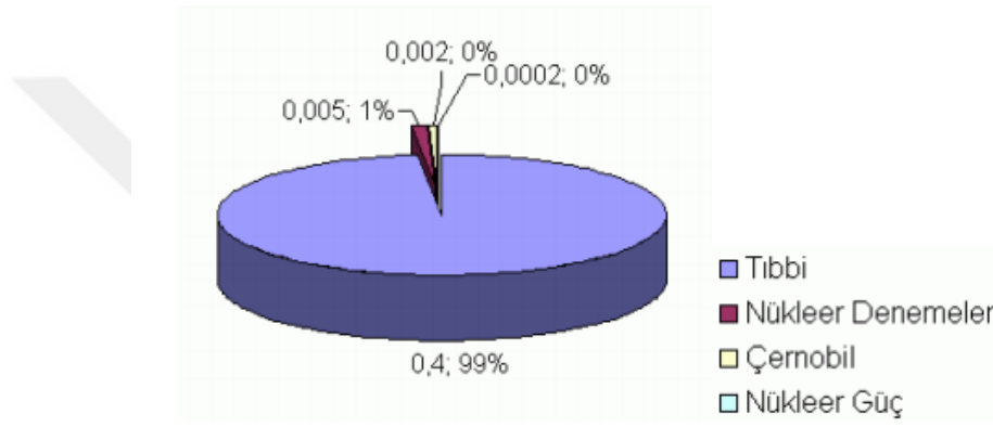
Şekil 2.9: Yapay radyasyon kaynakları (Davutoğlu, 2008)
