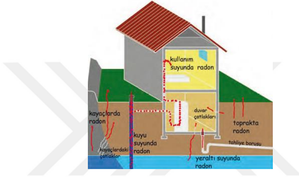
Şekil 2.17: ^{222}\text{Rn} 'nin binaya giriş yolları (Url-11)
