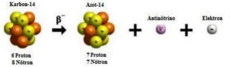
Şekil 2. 3: \beta^- bozunumu (Özkan, 2011)
