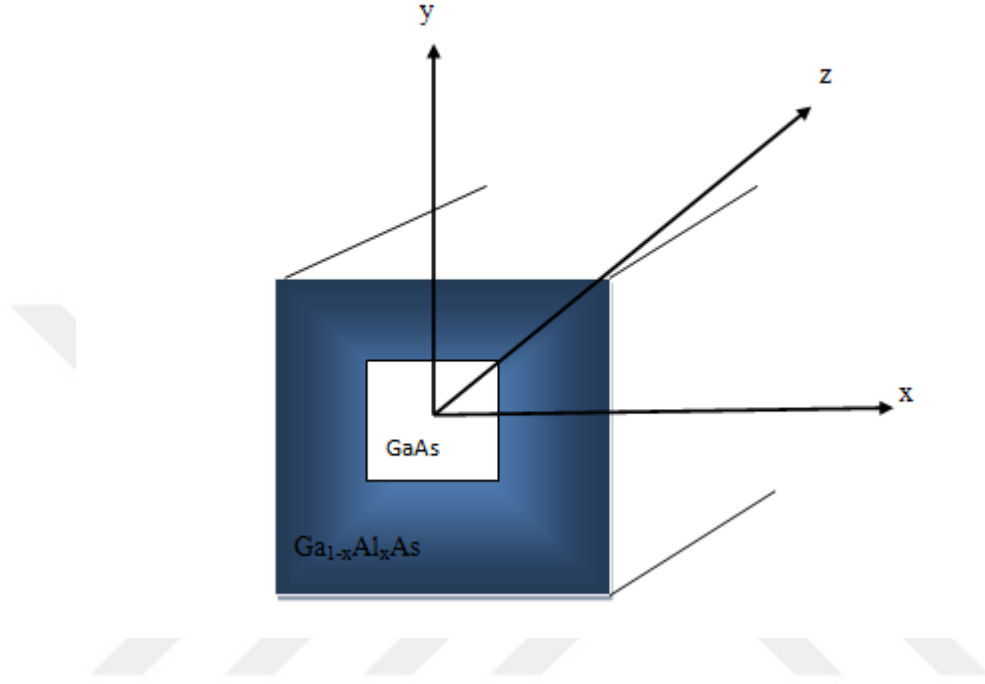
Şekil 2.4: Kuantum telinin şematik gösterimi.
