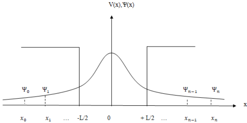
Şekil 4.2: Sonlu farklar yönteminin kuantum kuyularına uygulaması.
