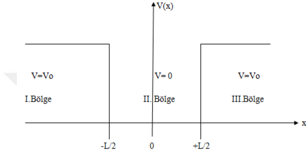
Şekil 2.3: Sonlu kuantum kuyusunun şemantik gösterimi.
