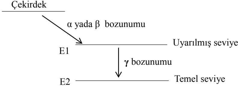
Şekil 2.4. Gama bozunumu
