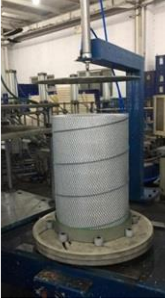
Resim 4.9. Otomatik döner tabla
