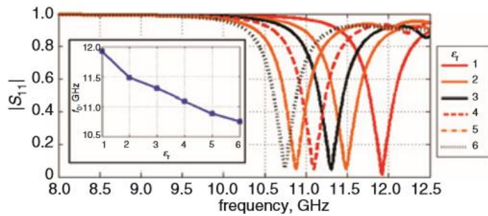
Şekil 1.2. S11 yansıma ve lineerlik grafiği [15]
