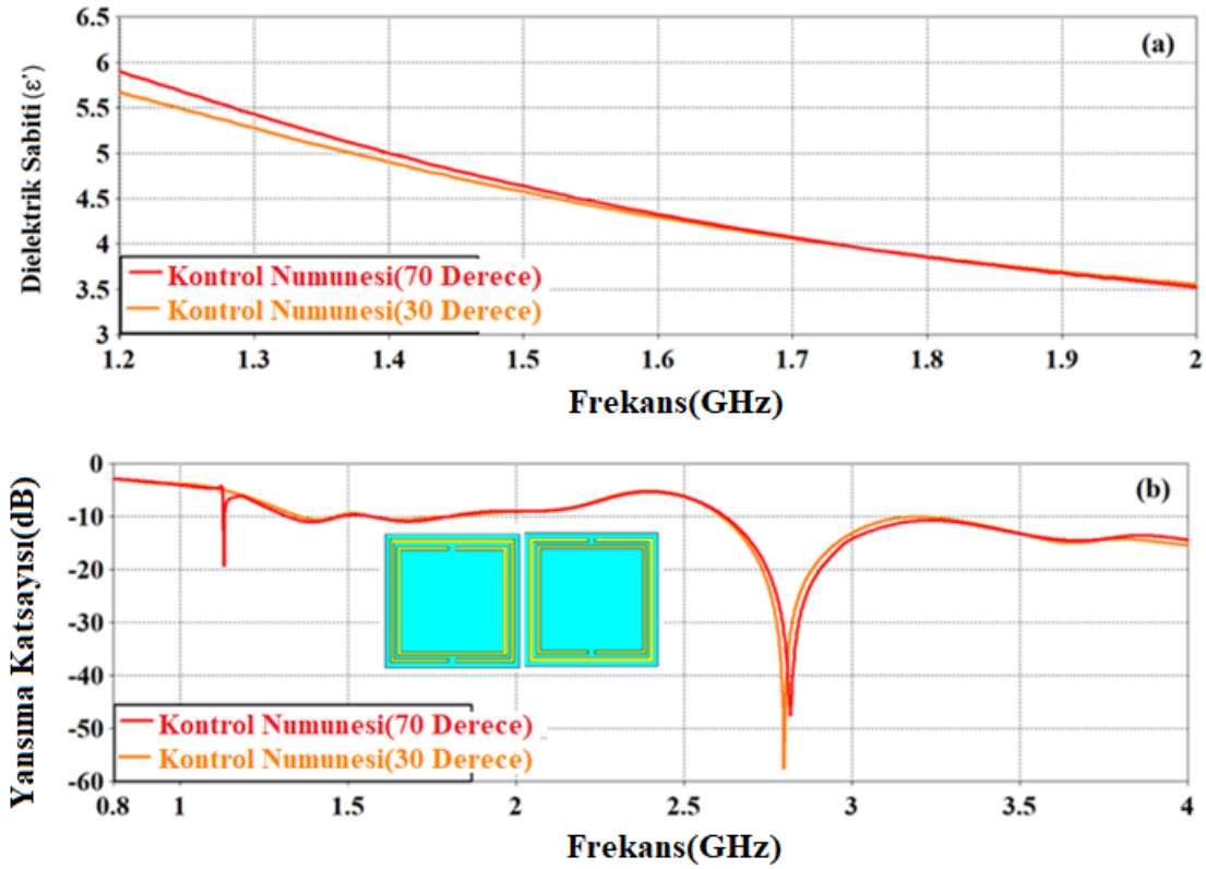
Şekil 4.56. Kontrol numunesinin farklı sıcaklıklardaki dielektrik sabiti grafiği (a) ve yansımaya katsayısı grafiği (b)
