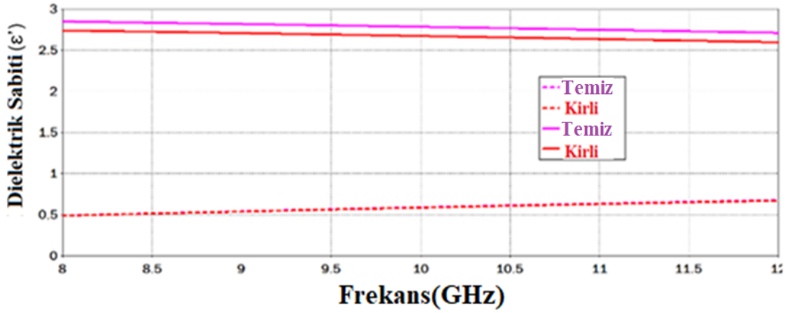
Şekil 4.27. Temiz ve kirli trafo yağının dielektrik sabiti grafiği
