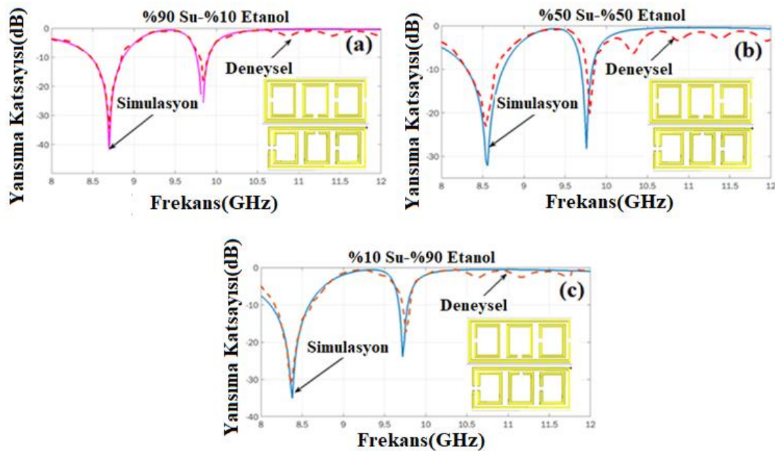
Şekil 4.62. %10, %50 ve %90 yoğunluktaki numunelerin yansımaya katsayısı grafiği
