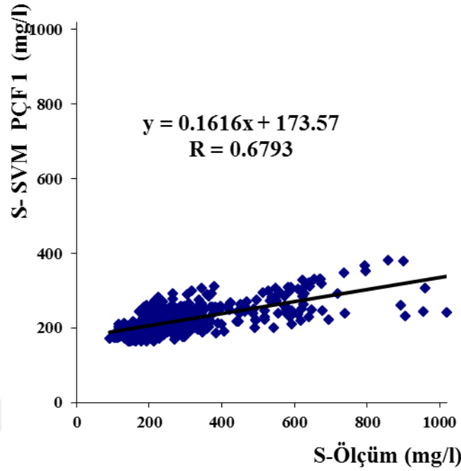
Şekil 4.28. Askıdaki sediment miktarı test verileri için DVM-PÇF 1'e ait saçılım grafiği
