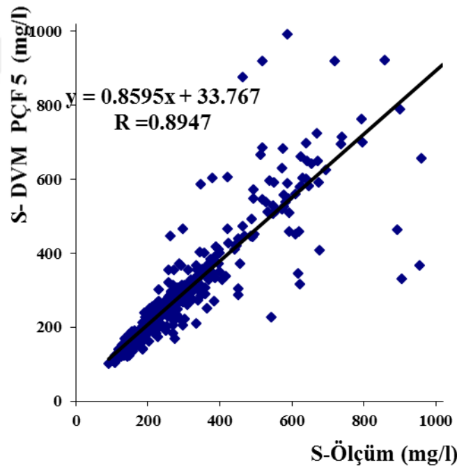
Şekil 4.43. Askıdaki sediment miktarı eğitim verileri için DVM-PÇF 5'e ait ölçüm ve dağılım grafiği
