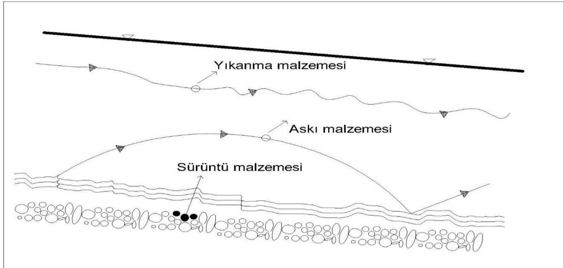
Şekil 1.2. Akarsudaki katı maddelerin hareket ve taşınım türleri
