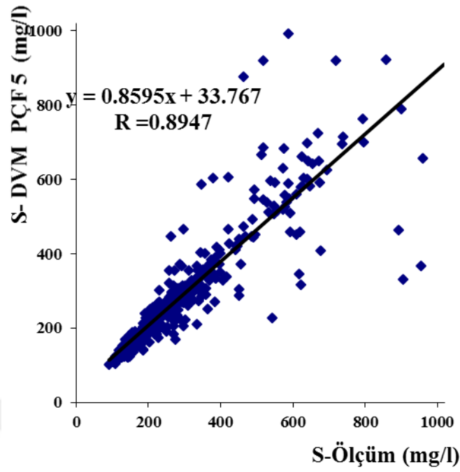
Şekil 4.44. Askıdaki sediment miktarı test verileri için DVM-PÇF 5'e ait saçılım grafiği
