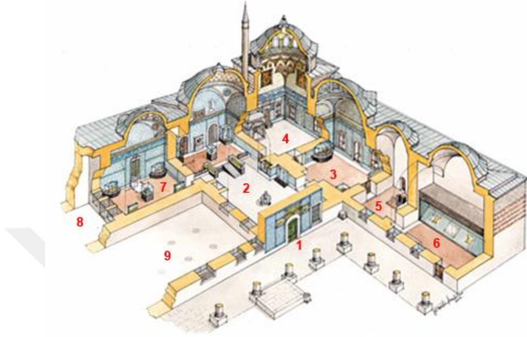
Resim-30 Has Oda Dairesi Üst Kat Perspektif Çizimi
