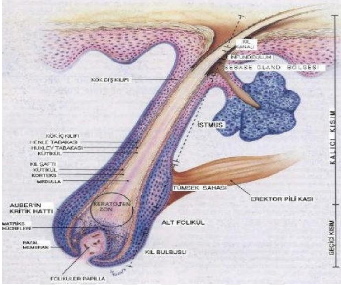
Şekil 1. Kılın yapısı.
