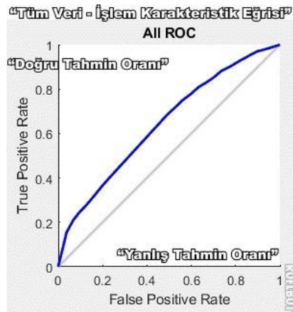
Grafik 10: Tüm Veri - İşlem Karakteristik Eğrisi
