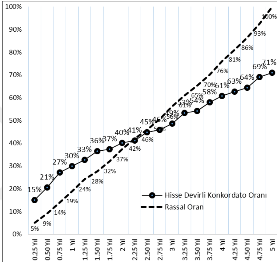
Grafik 2: Gözlem Dönemi Karşılaştırmalı Olasılık Grafiği
