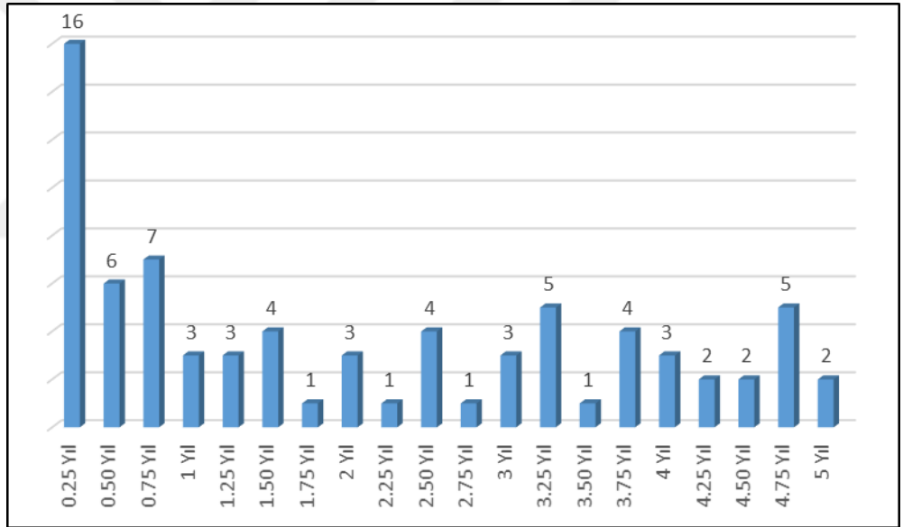
Grafik 1: Gözlem Dönemi Hisse Devirli Konkordatolar Grafiği
