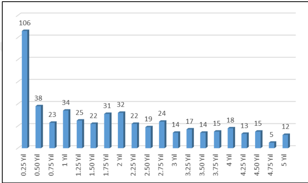
Grafik 3: Sınama dönemi - Hisse Devirli Konkordatolar Grafiği
