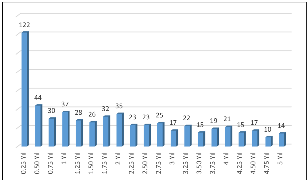
Grafik 5: Gözlem + Sınama Dönemi Hisse Devirli Konkordatolar Grafiği
