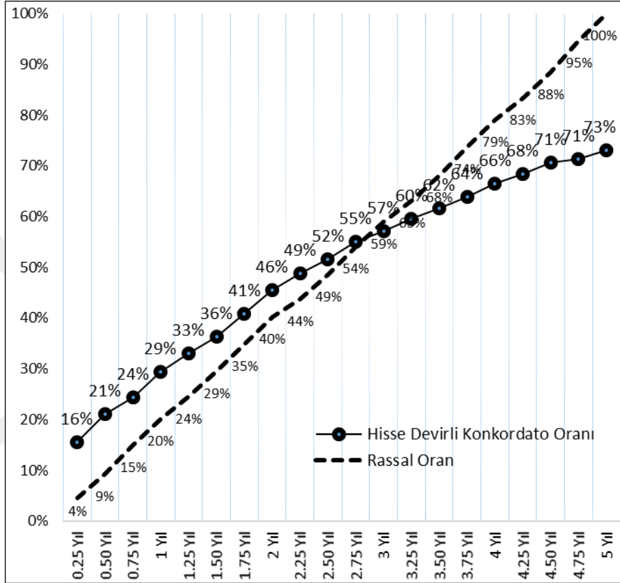
Grafik 4: Sınama Dönemi Karşılaştırmalı Olasılık Grafiği
