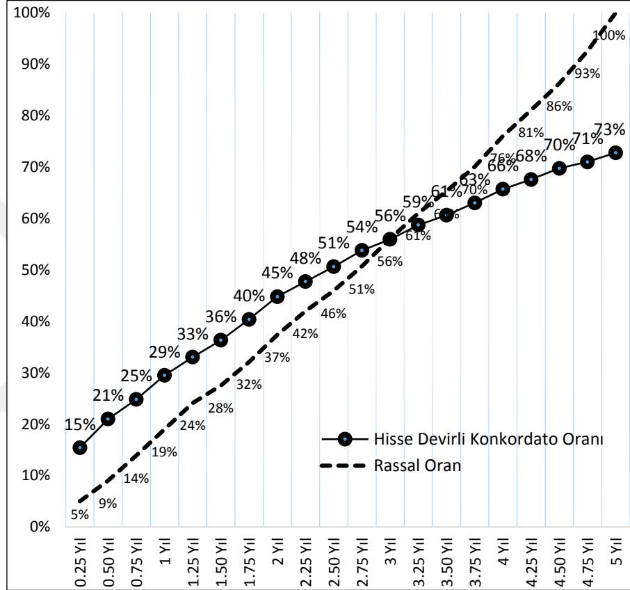
Grafik 6: Gözlem + Sınama Dönemi Karşılaştırmalı Olasılık Grafiği
