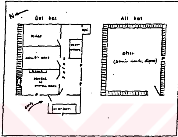
Şekil 15 Semen kışlakında çift katlı bir evin planı. Evin yapı tarzı yayla-oba evlerinden farklıdır; birer fazla odalar, üst katın bölümleri ve zemin ahşap malzeme ile yapılmış, içinde yiyeceklerin depolandığı bölümler vardır.
