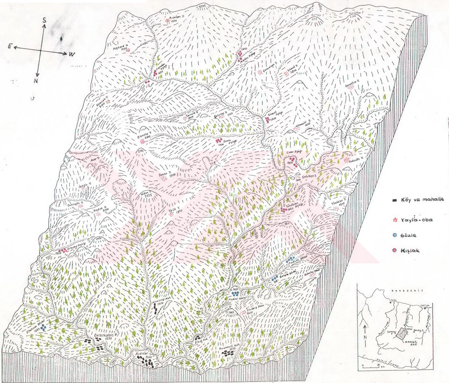
Sekil 4 – Pazarsuyu vadisinin yukarı kısmında yer alan devamlı ve geçici yerleşmeleri gösteren blokdiyagram.
