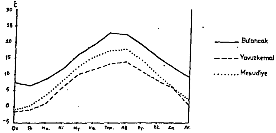
Şekil 1 - Ortalama Sıcaklık Grafiği
