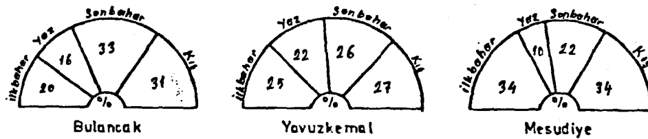
Şekil 3 - Mevsimlere Göre Yağışın Dağılışı
