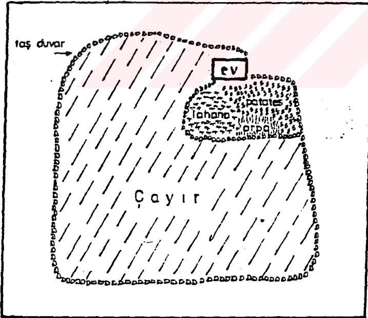
Şekil 16 - Melense yaylasında bir yaylacının kullandığı arazi: Burada, evin yakınında etrafı taş duvarla çevrili "bağlak" adı verilen geniş bir alan ot üretimine ayrılmıştır. Bir kenarında daha çok patates ve lahana ile nadiren arpa ekilidir.
