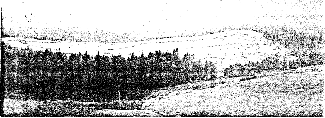
Resim 9- Yaylaların çoğunluğu orman içi veya orman yakınındadır. Resimde, tamamen orman içinde kurulu Karatepe yaylası ile ikinci planda , Büyükdüz ve Dereyatak obaları yer alıyor.
