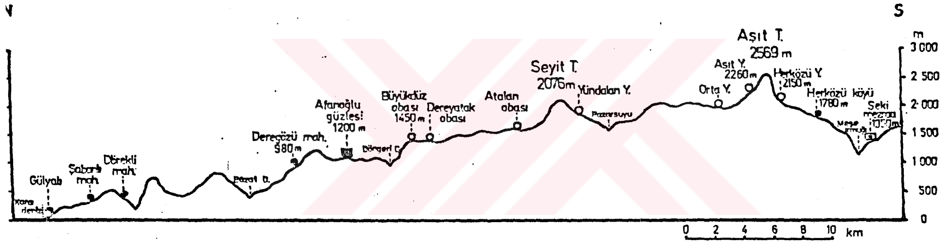
Şekil 6-Gülyalı ilçesi ile Meşe ırmağı arasında kuzey-güney yönünde alınmış bir profil.
