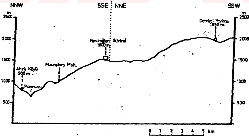
Şekil 10 Pazarısu vadisinde Ahırlı köyünden güzle ve yayla alanına doğru NNW-SSE ve NNE-SSW yönünde alınmış bir profil.
