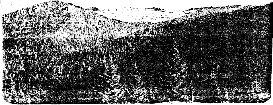
Resim:20- Yaylaya gıkny ve dörüste bir süne ka- lıca "güzle" ger'ıneleclı, orman içındı bo- şluklarda kızıdır. Resimde geri olıada, fanık- ođlan güzlesı görülmektedir.
