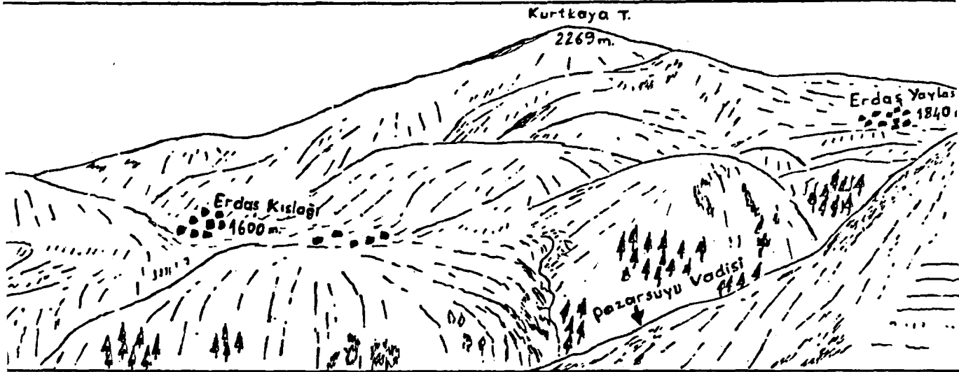
Şekil 8-Pazarsuyu vadisinin yukarı çığırında Erdaş kışlağı ile Erdaş yaylasını gösterir diyagram.
