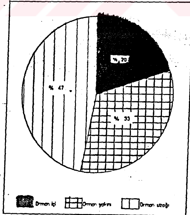
Şekil 5- Yayla-oba yerleşim yerleri ve orman ilişkileri
