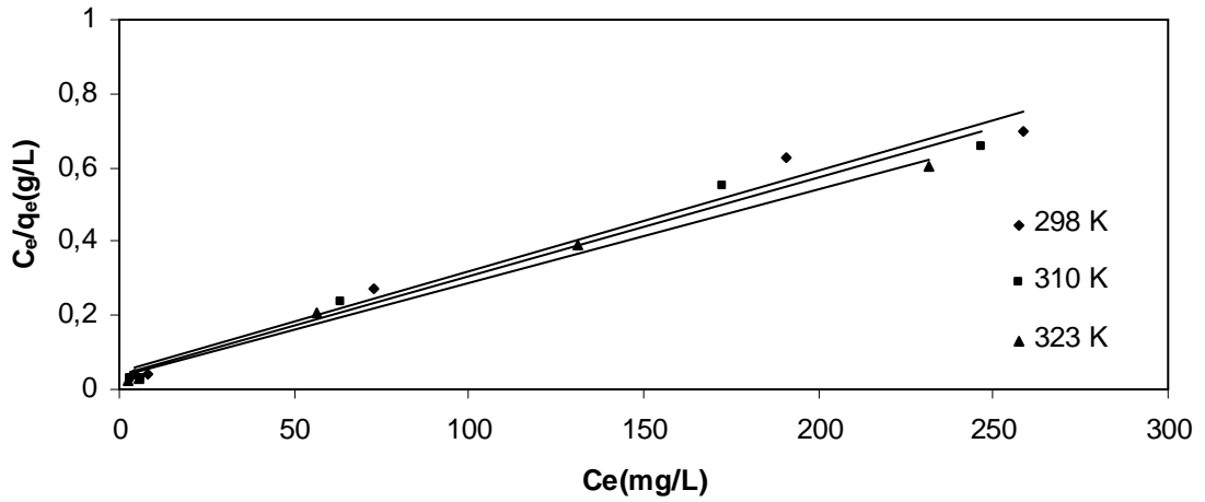
Şekil.4.30. Farklı sıcaklıklarda BK481 aktif karbonu ile kafein adsorpsiyonu için Langmuir İzotermi.
