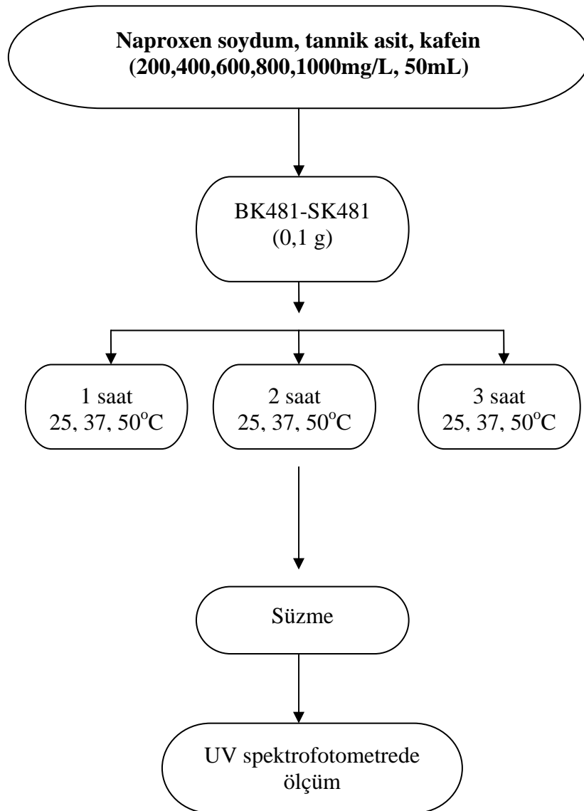
Şekil 3.1. Naproxen sodyum, tannik asit ve kafein için BK481 ve SK481 aktif karbonları ile izoterm çalışması akış şeması.
