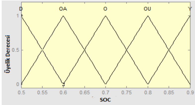
Şekil 3.12. ECE-15 sürüş çevrimi için SOC üyelik fonksiyonu
