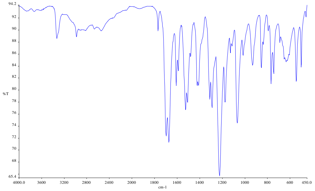
Şekil 4.1.3.b. 4-(Propoksikarbonilamino)benzoik Asidin FTIR Spektrumu
