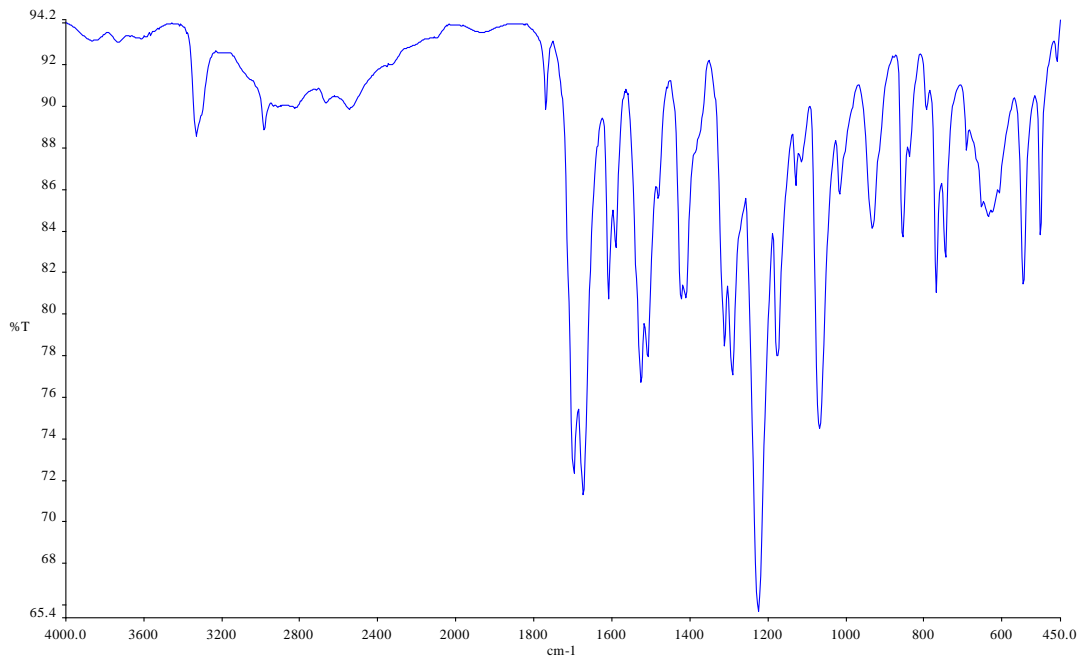
Şekil 4.1.4.b. 4-(Bütoksikarbonilamino)benzoik Asidin FTIR Spektrumu
