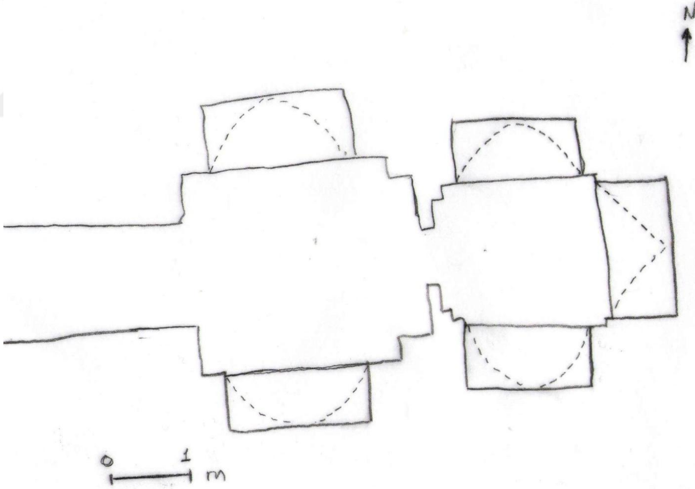
Çizim 29. 15 numaralı mezar, plan
