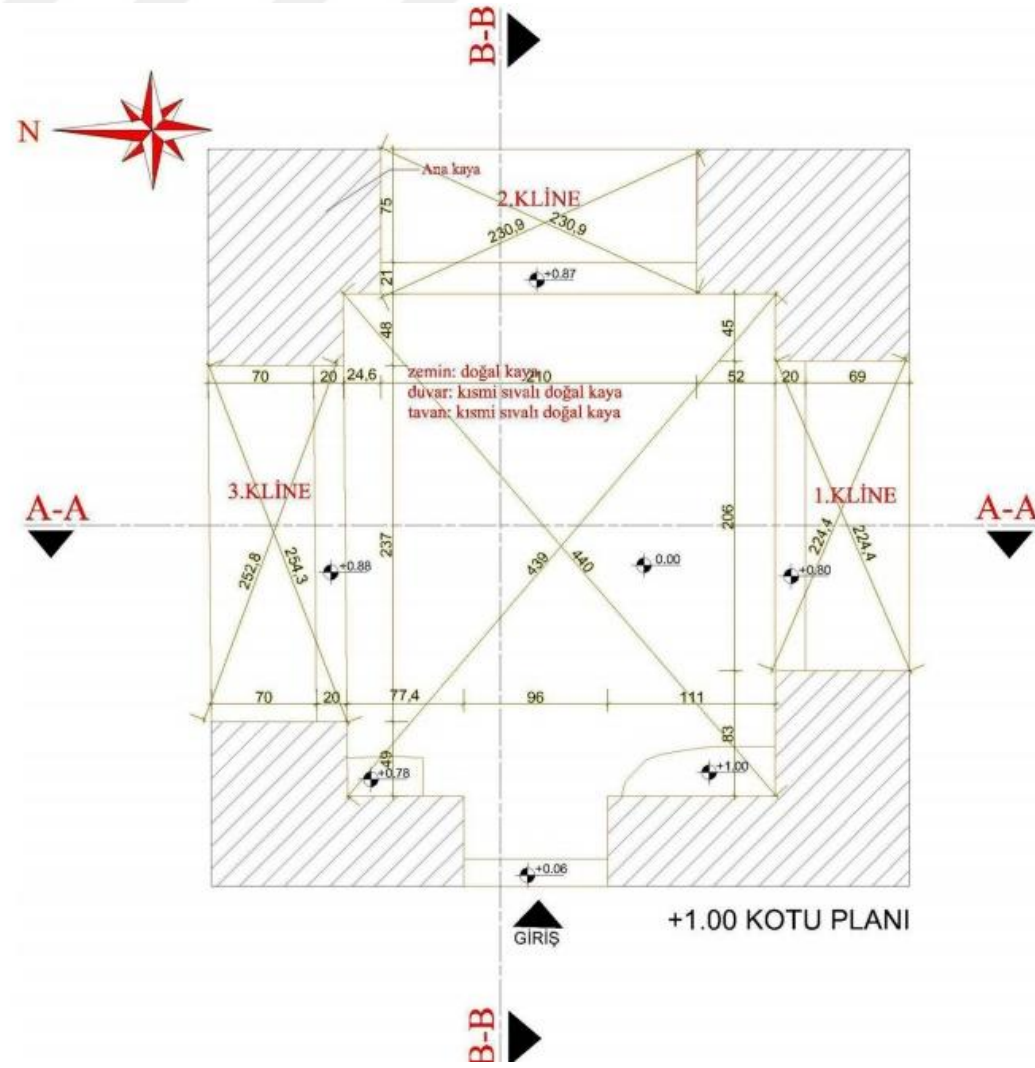
Çizim 41. 21 numaralı mezar, plan
