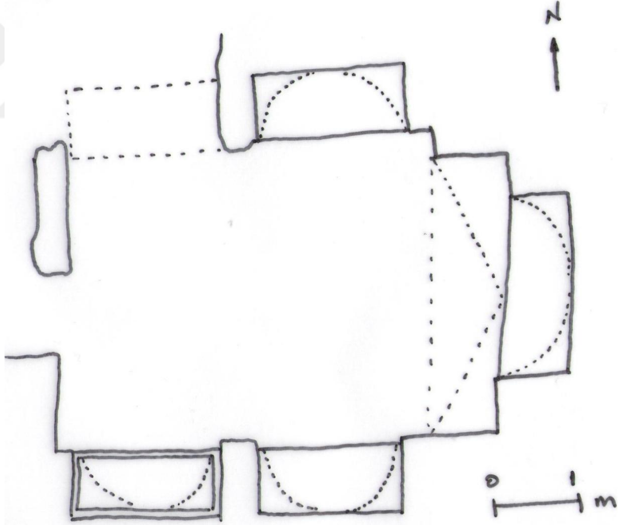
Çizim 17. 9 numaralı mezar planı
