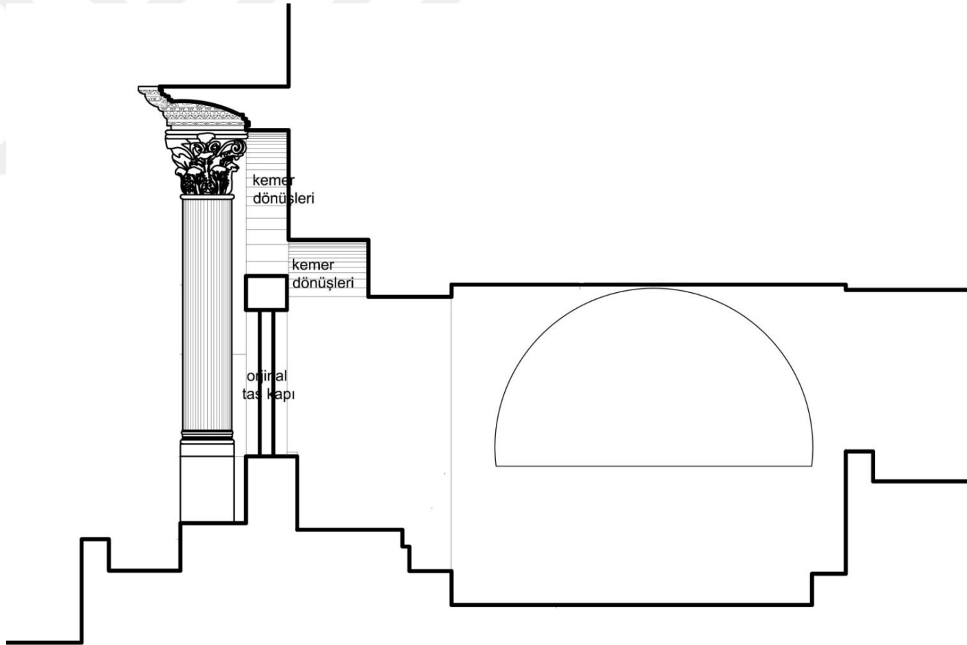
Çizim46. 22 numaralı mezar odası batı-doğu kesiti
