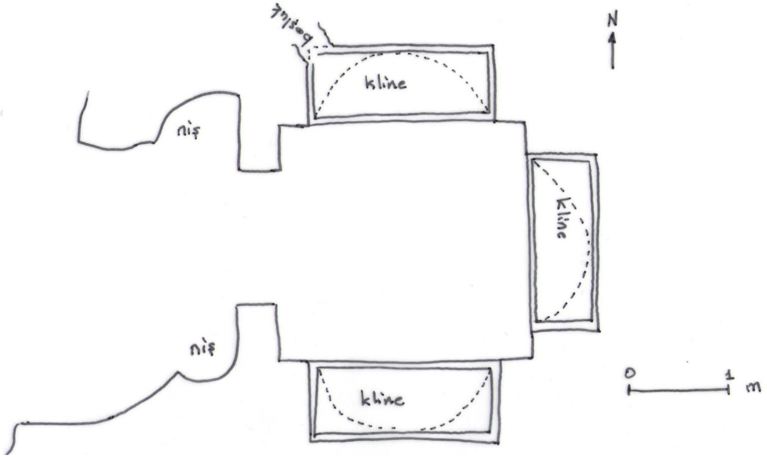
Çizim 3. 2 numaralı mezar, plan
