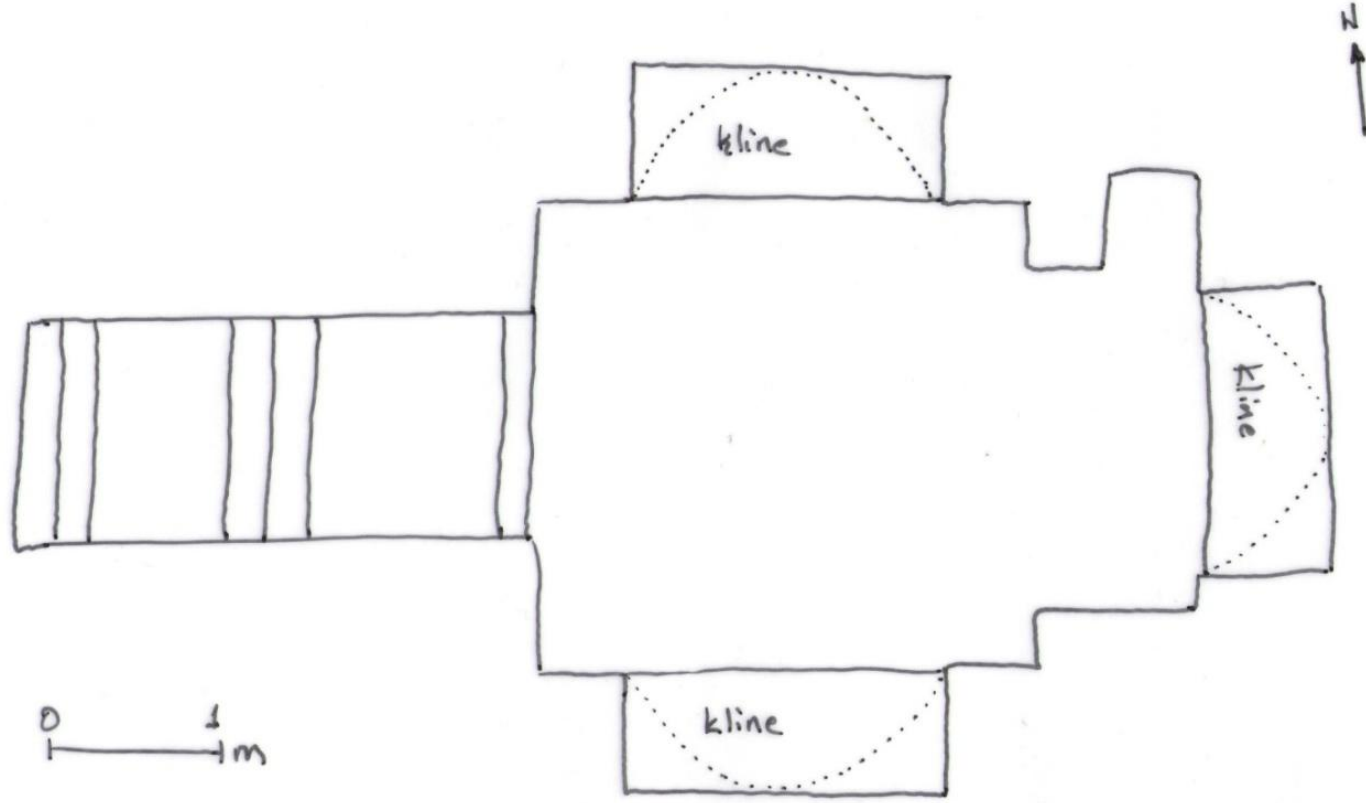
Çizim 7. 4 numaralı mezar, plan
