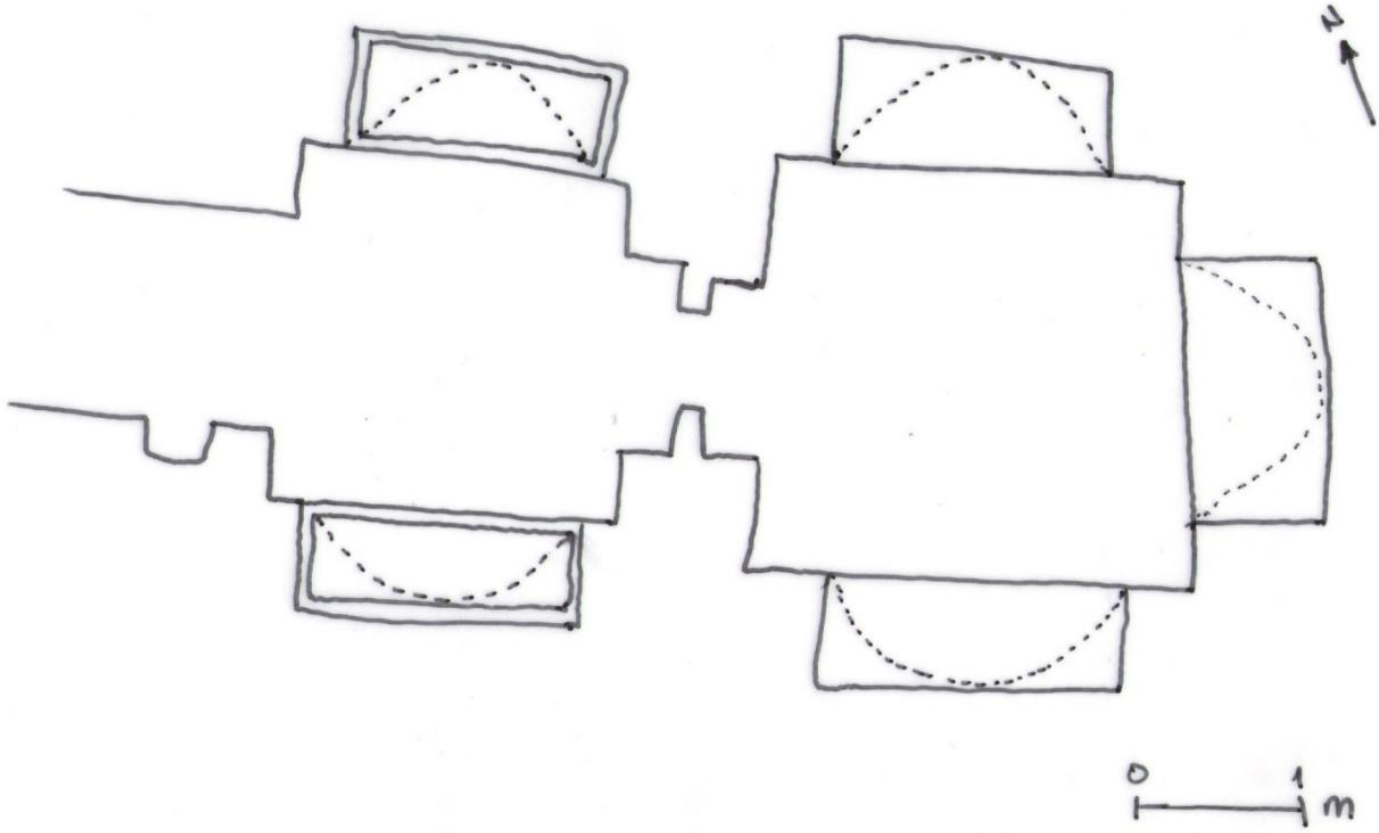
Çizim 9. 5 numaralı mezar, plan
