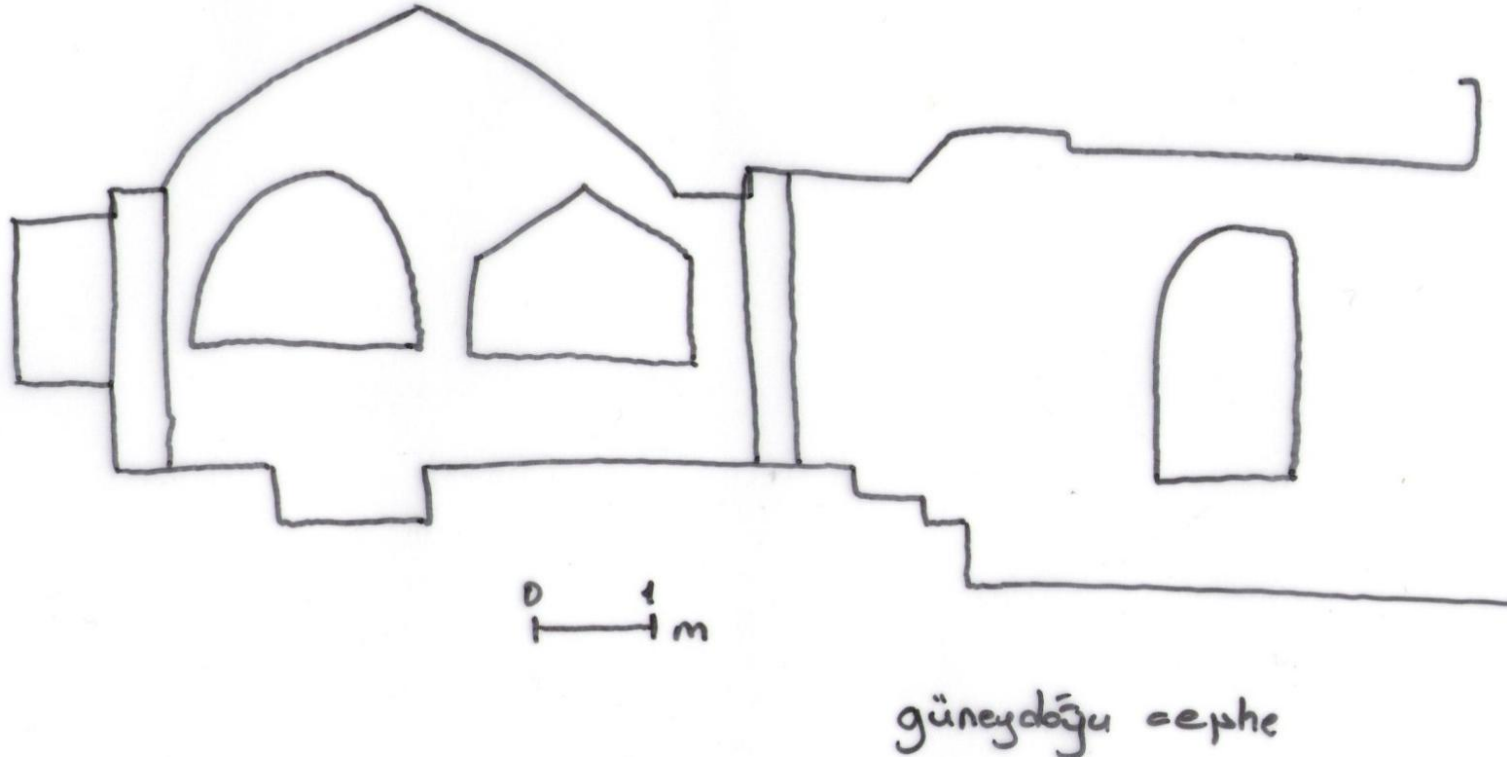
Çizim 16. 8 numaralı mezar-kesit
