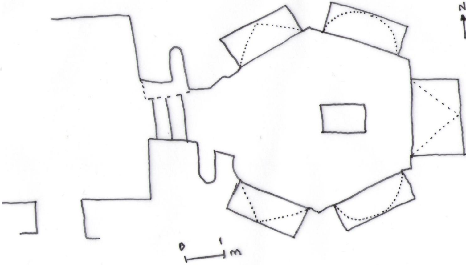
Çizim 15. 8 numaralı mezar planı
