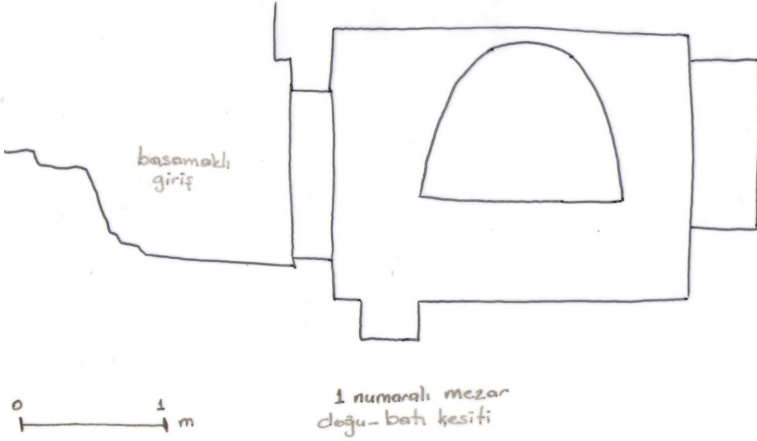
Çizim2. 1 numaralı mezar, kesit
