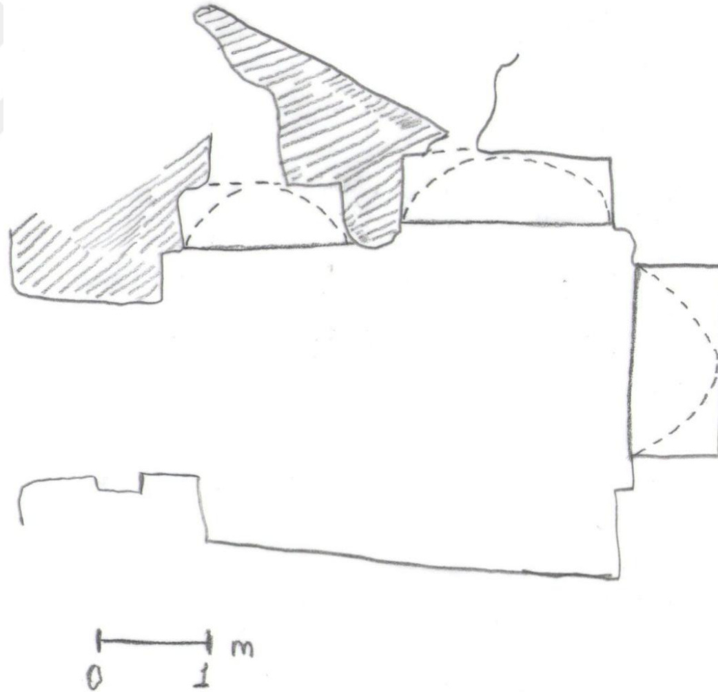
Çizim35. 18 numaralı mezar, plan
