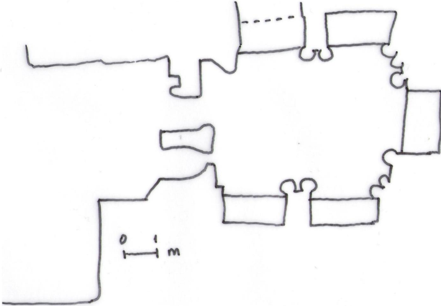
Çizim 19. 10 Numaralı mezar, plan
