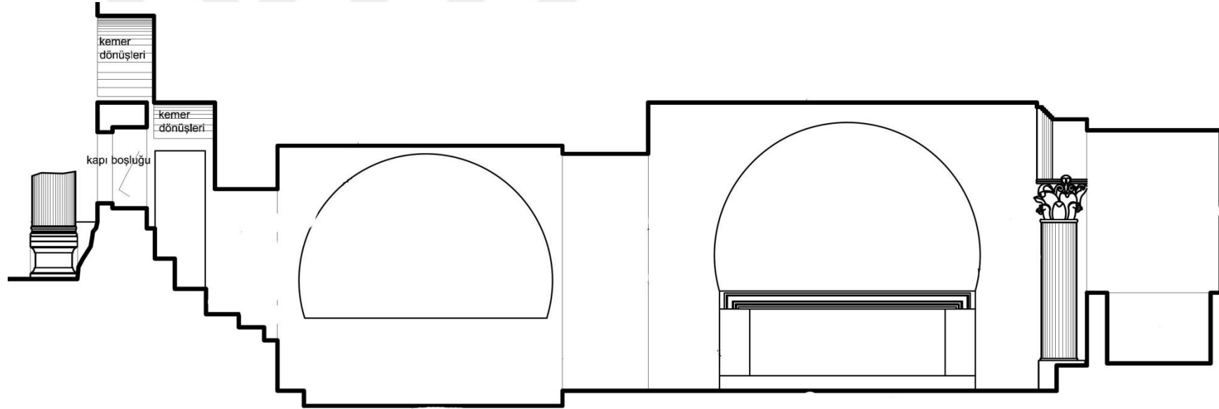
Çizim49. 23 numaralı mezar, batı-doğu kesiti
