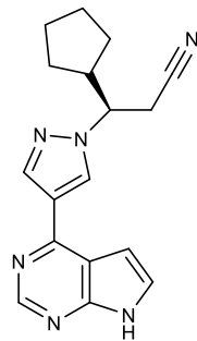
Ruksolitininib
