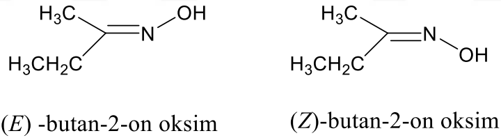
Şekil 2.22. E-Z oksim izomer örnekleri
