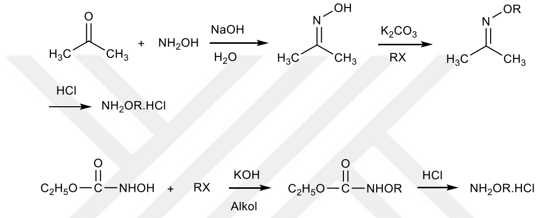
Şekil 2.48. Hidroksilaminin amin grubunun korunmasından sonra O-alkil hidroksil amin eldesi
