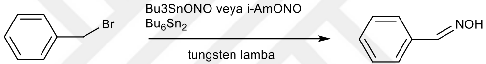
Şekil 2.34. Benzil bromürden benzaldoksim sentezi
