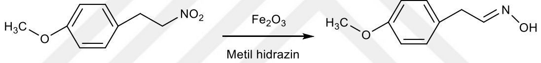
Şekil 2.28. Fe 2 O 3 eşliğinde oksim sentezi
