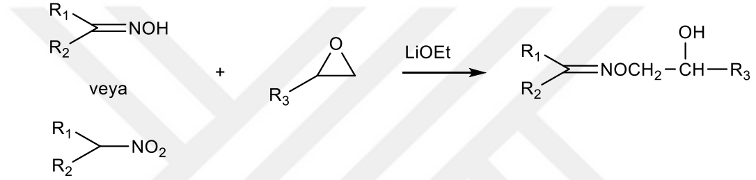
Şekil 2.39. O-Alkilasyon reaksiyonu ile oksim eter sentezi
