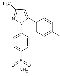
Selekoksib
