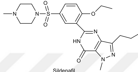
Sildenafil
