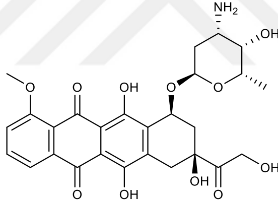
Şekil 2.62. Doksorubisin
