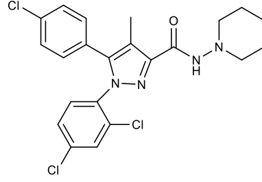
Rimonabant
