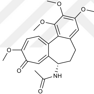
Şekil 2.59. Kolşisin
