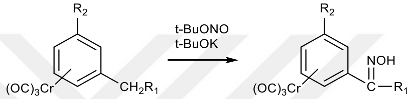
Şekil 2.37. Benzilik pozisyonundan nitorlanması ile oksim sentezi
