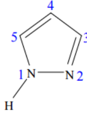
Şekil 2.1. Pirazol halkası
