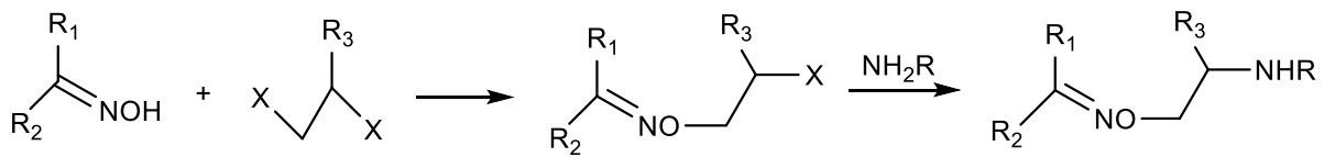
Şekil 2.44. Dihaloalkanlarla alkilasyon ile oksim eter sentezi
