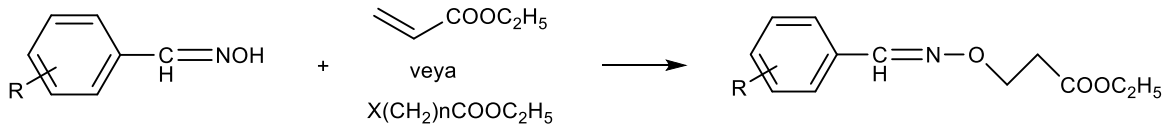
Şekil 2.43. Michael tipi katım reaksiyonu ile oksim eterler sentezi
