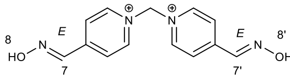
Şekil 2.53. ( E )-1-((4-(( E )-(hidroksiimino)metil)-1,4-piridin-1-il)metil)-1,4-piridin-4-karbaldehit oksim (b)
