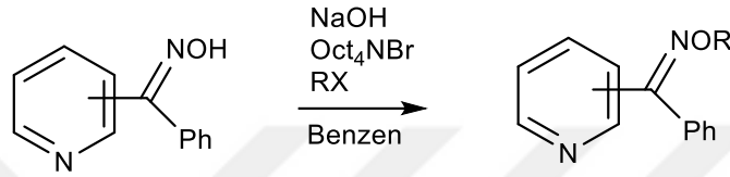
Şekil 2.42. Alkil halojenürlerle oksim eter sentezi
