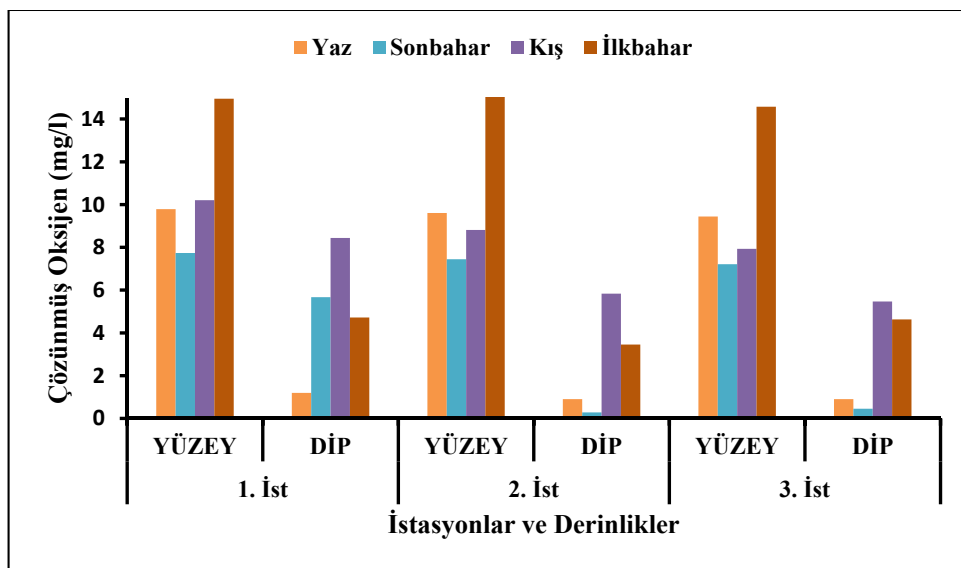
Şekil 3.4.1: İstasyonlarda mevsimsel olarak belirlenen ortalama ÇO değişimleri (mg/l).
