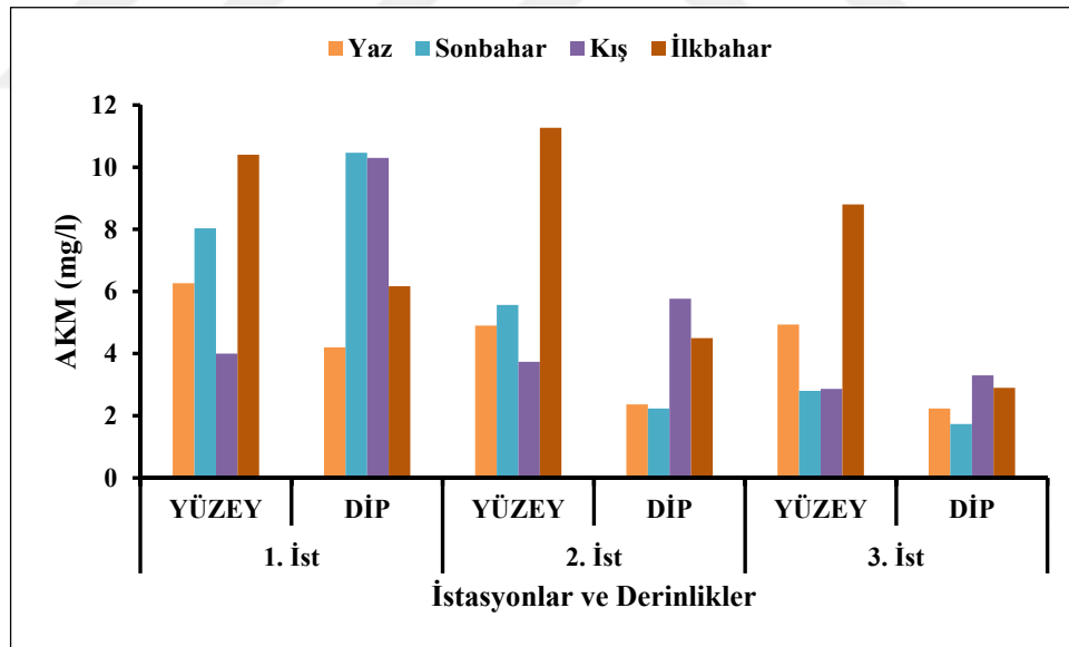
Şekil 3.9.1: İstasyonlarda mevsimsel olarak belirlenen ortalama AKM değışimleri (mg/l).
