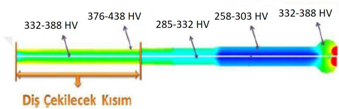
Şekil 4.24 : Simülasyon sonucunda elde edilen sertlik tahminleri
