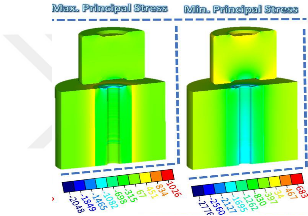
Şekil 4.21 : M6x30 DIN 933 2.istasyon kalıplarının gerilme dağılımı
