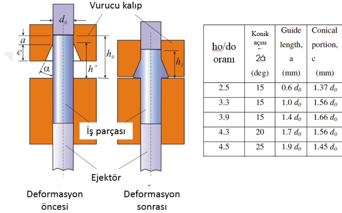
Şekil 3.14 : Armudi işlemi
