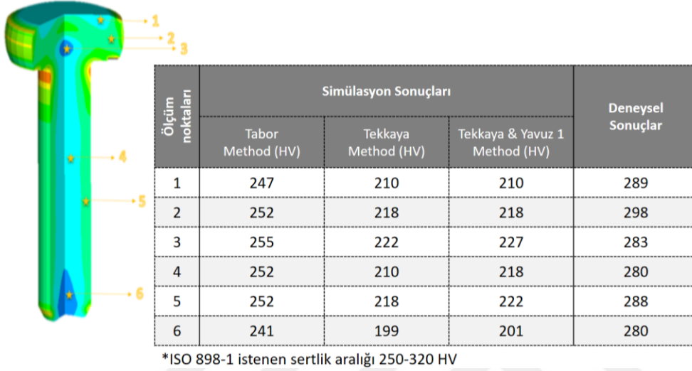
Şekil 5.16 : M6x30 DIN 933 22MnB5Ti malzemesi ürün sertlik tahmini
