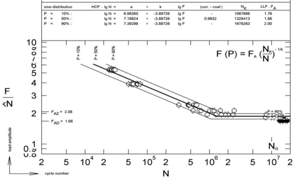
Şekil 5.31 : 35V1 wöhler eğrisi
