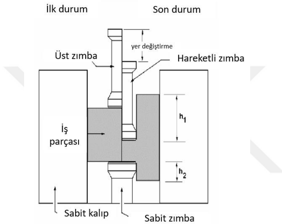
Şekil 3.8 : Geriye bardak akıtma test düzeneği
