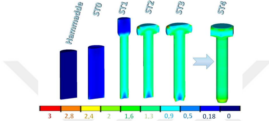
Şekil 4.19 : M6DIN933(22MnB5Ti) istasyonlara göre eşdeğer plastik genleme dağılımı
