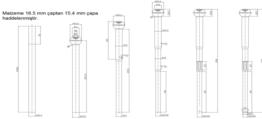
Şekil 4.22 : İstasyon tasarımı
