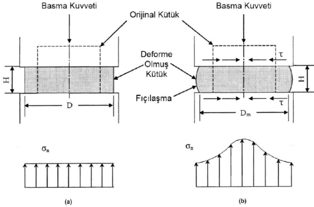
Şekil 3.5 : Silindirik iş parçasına uygulanan yığıma işlemi. a) Sürtünmesiz. b) Sürtümlü. [20]
