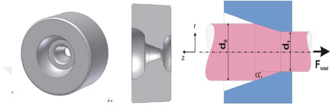
Şekil 2.4 : Hadde kalıbı
