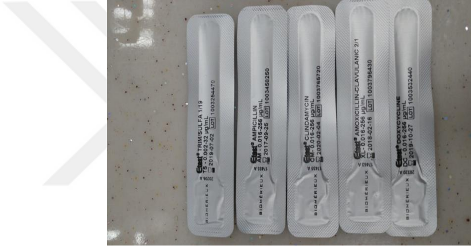
Şekil 5.2: E-test stripleri.
