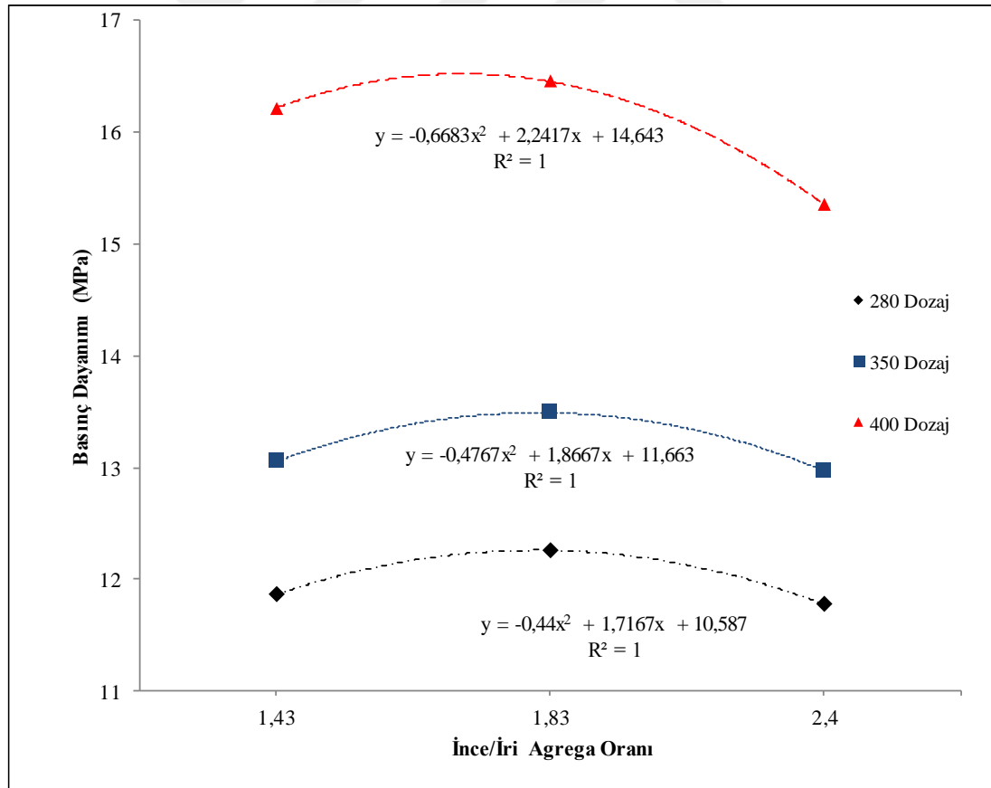
Şekil 4.4 : Basınç dayanımı agregada incelik oranı ilişkisi.
