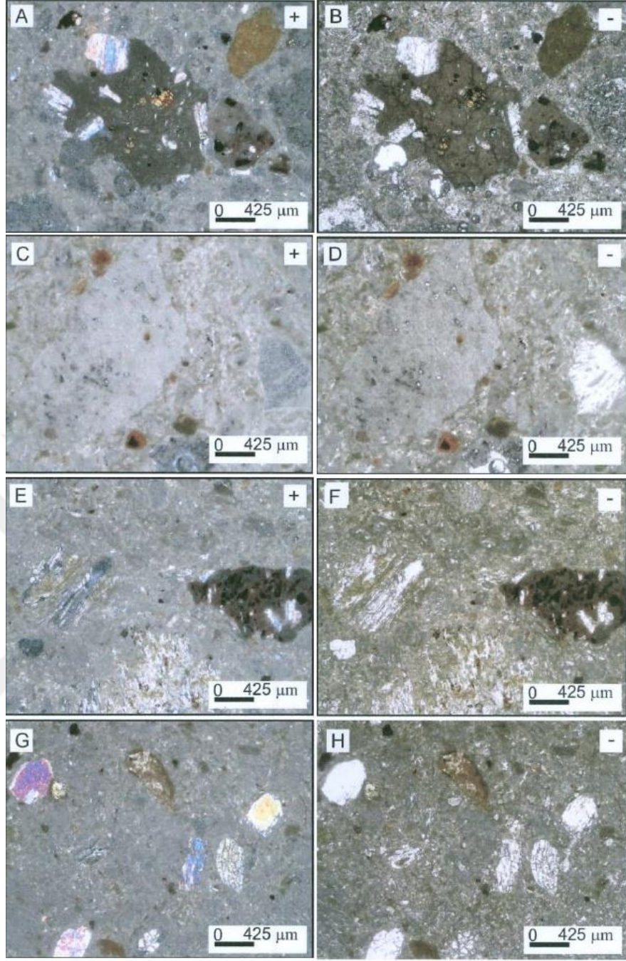
Şekil 3.2 : İzmir-Alaçatı taşı kayaç yapısına ilişkin mikroskobik görünümler [22].
