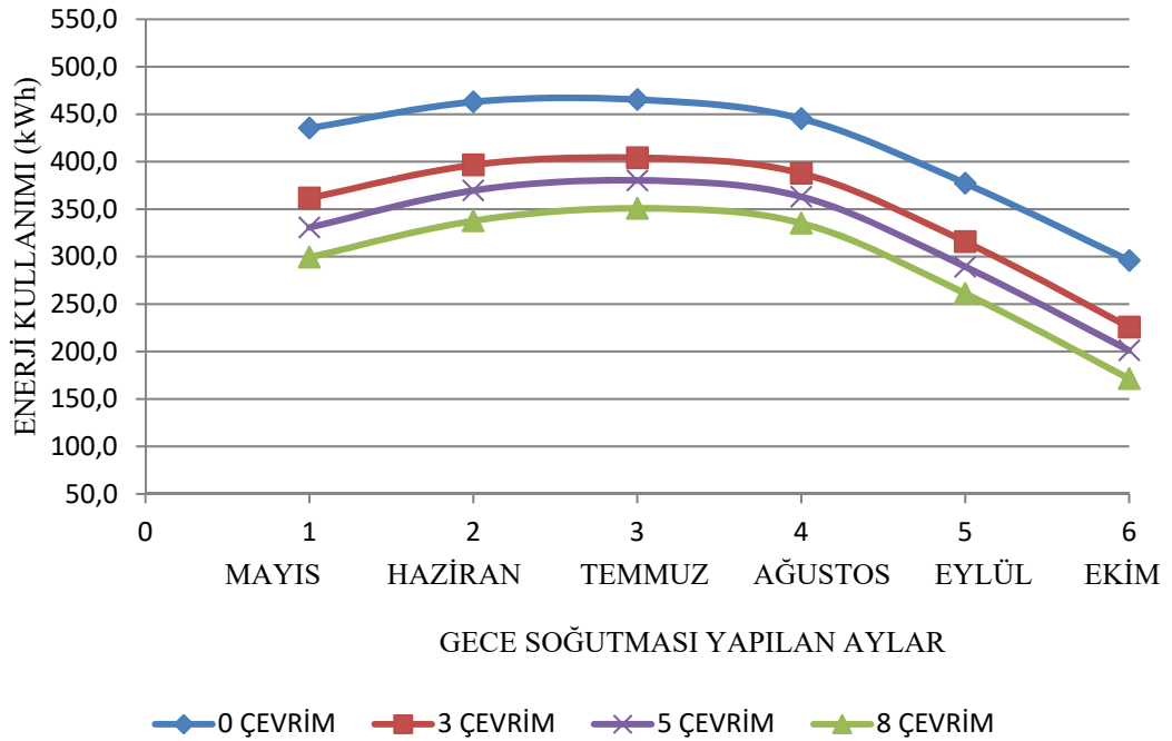
Şekil 6.3 : İstanbul için aylık enerji ihtiyacı.
