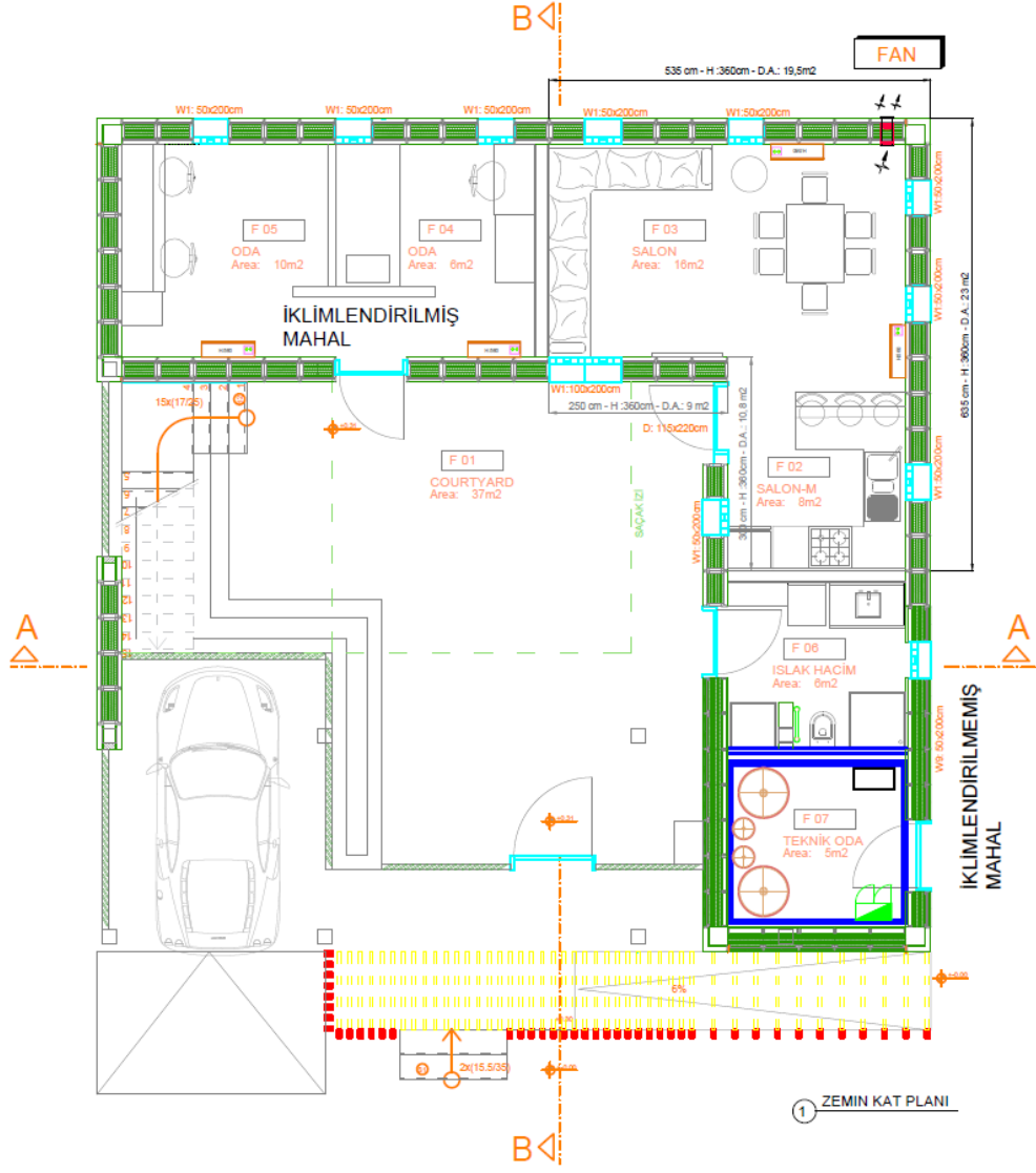
Şekil A. 1 : Örnek yapının mimarisi.
