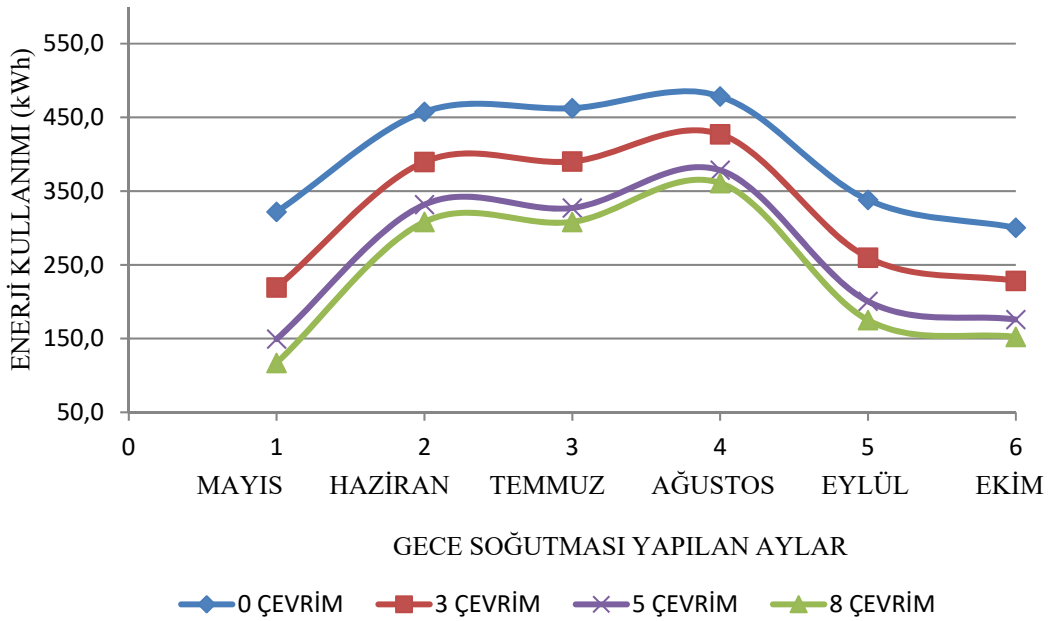
Şekil 6.9 : 27°C set değeri için Ben Guerir için aylık enerji ihtiyacı.
