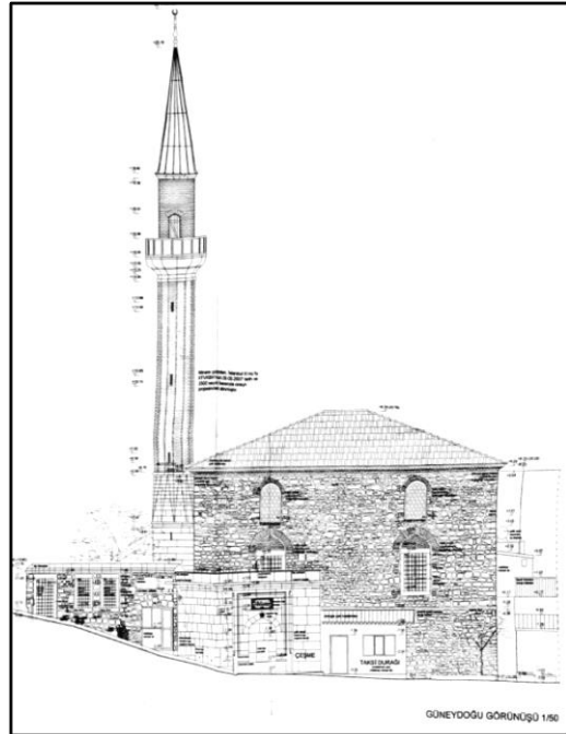
Resim 75- 6. Caminin Tadilatına ait Kesitler ve Görünüřler. (Vakıflar Genel Müdürlüğü)
