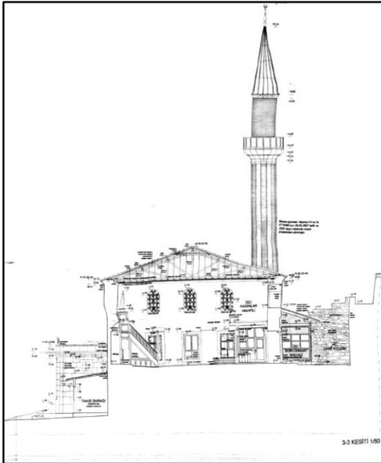
Resim 75- 6. Caminin Tadilatına ait Kesitler ve Görünüřler. (Vakıflar Genel Müdürlüğü)
