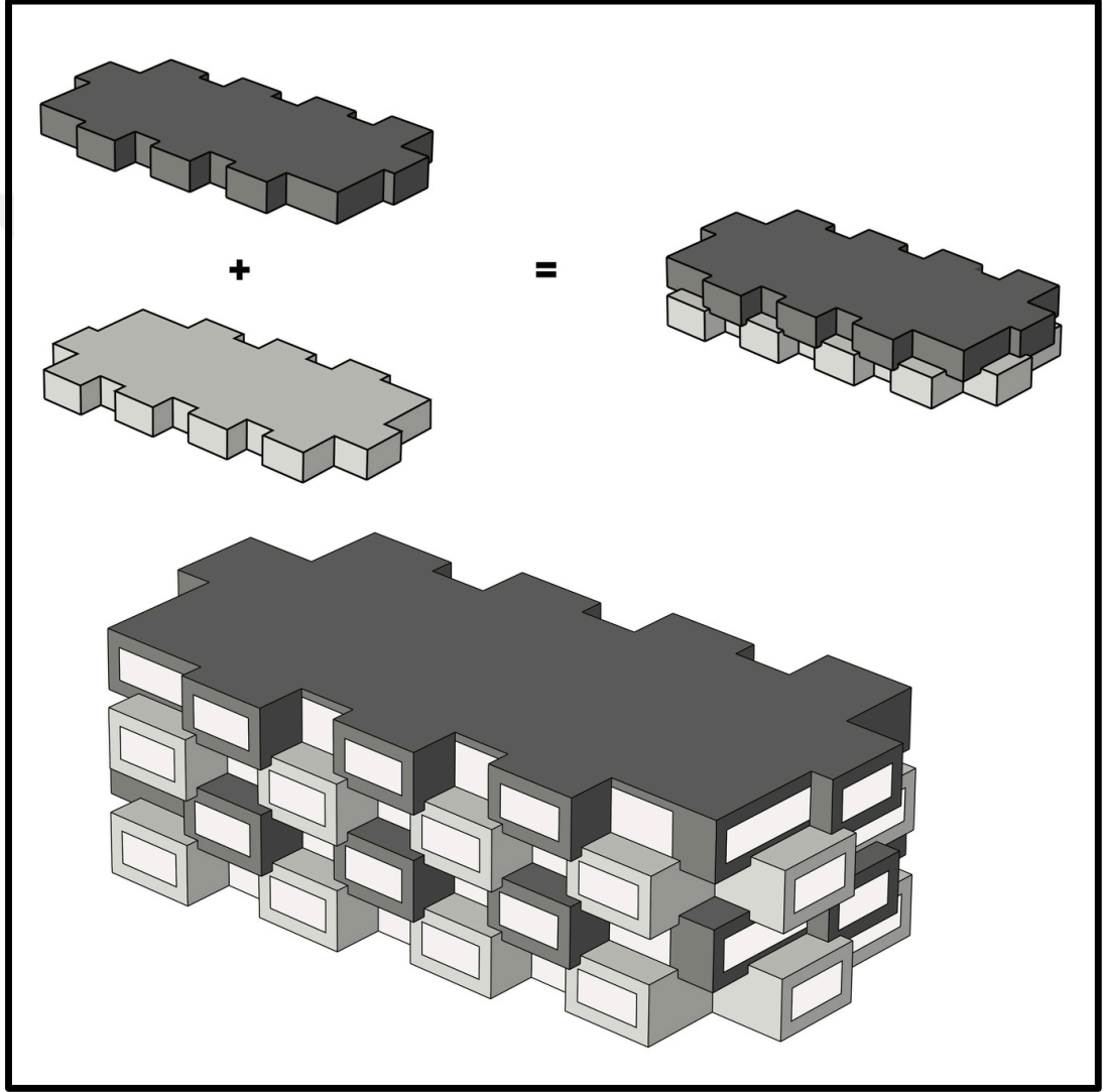
Şekil 5.31: Norra Tornen Innovationen Kat Birleşim Detayı (URL- 52)
