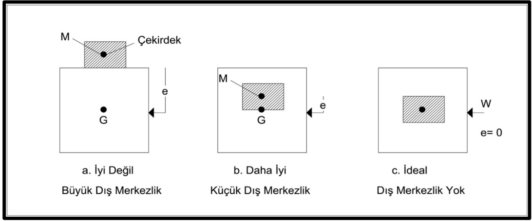
Őekil 4.16: a) B6y6k Dıřmerkezlik b) K66k Dıřmerkezlik c) Dıřmerkezlik Yok (6zgen ve Sev, 2000)
