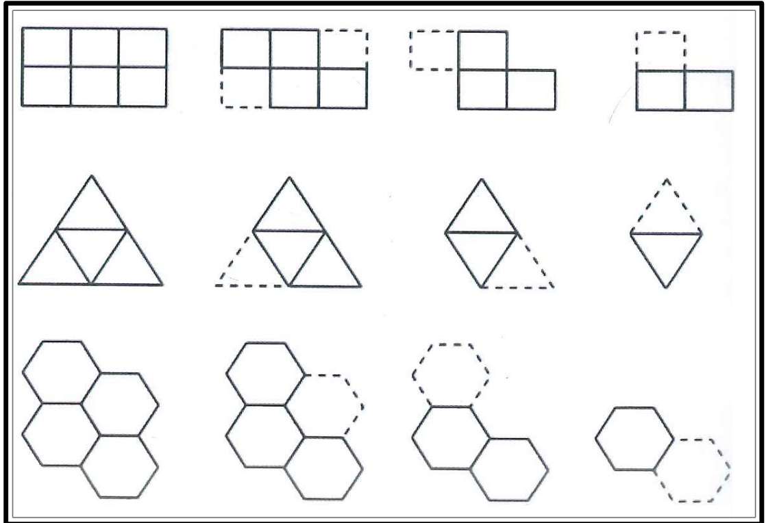
Şekil 3.73: Modüler Tüp Sistemleri Geometrik Şekilleri (Plan)
