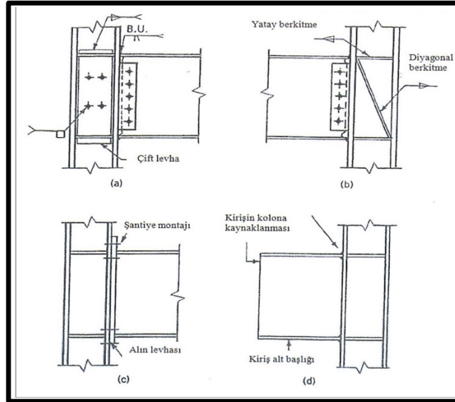
Şekil 3.14: Rijit Çerçevelerde Kolon Kiriş Birleşimleri: a - Bulonlu ve Kaynaklı, b - Bulonlu ve Kaynaklı - Köşegen Berkitmeli, c - Bulonlu ve Alın Levhalı, d - Kiriş alt başlığı Kiriş Kolona Kaynaklı (Sağlam, 2016)
