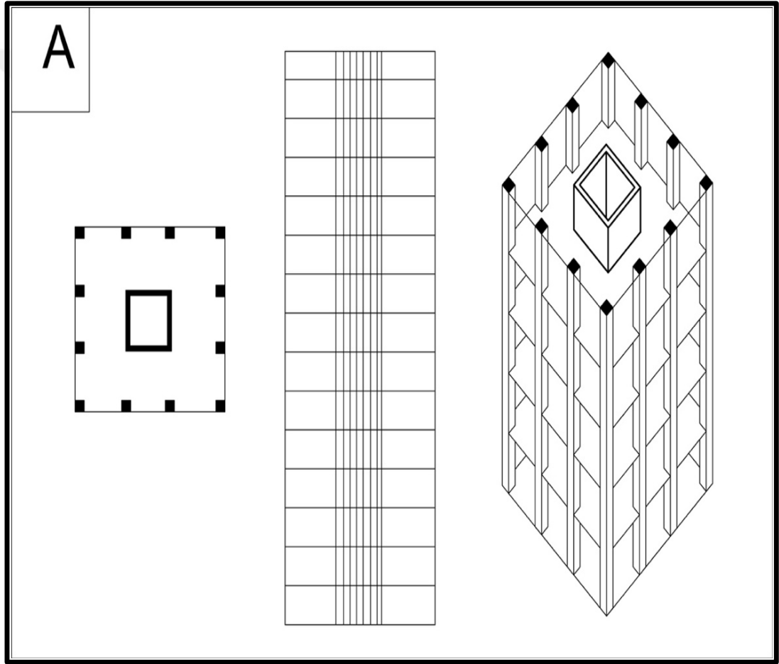
Şekil 4.27: Çekirdek ve Dış Kolonlu Sistem (Şekil 4. 25A)
