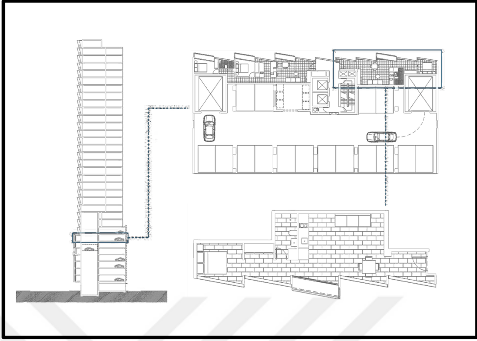
Şekil 5.19: A' Beckett Tower Sistem Detayı (URL- 49)
