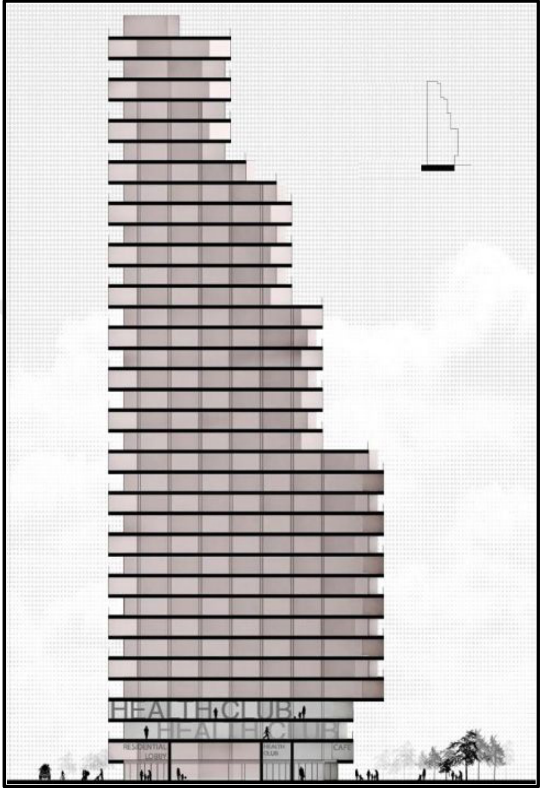
Şekil 5.32: Norra Tornen Innovationen Kesit (URL- 53)
