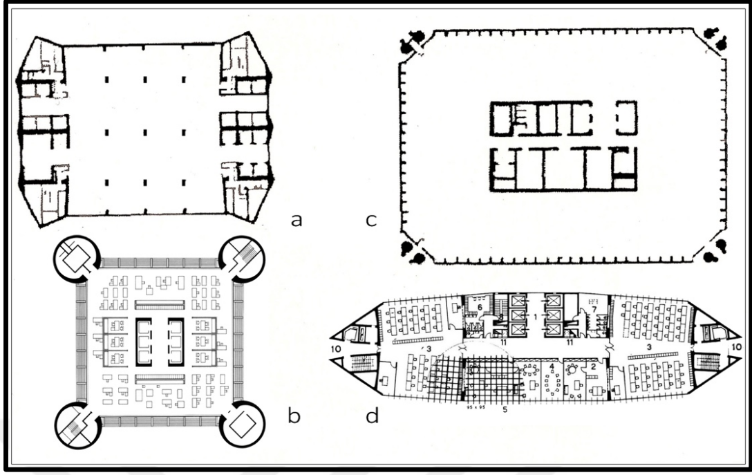
Şekil 4.5: a. Tour PB b. Knights of Columbus Building c. Tour de Bureaux d. Pirelli Binası
