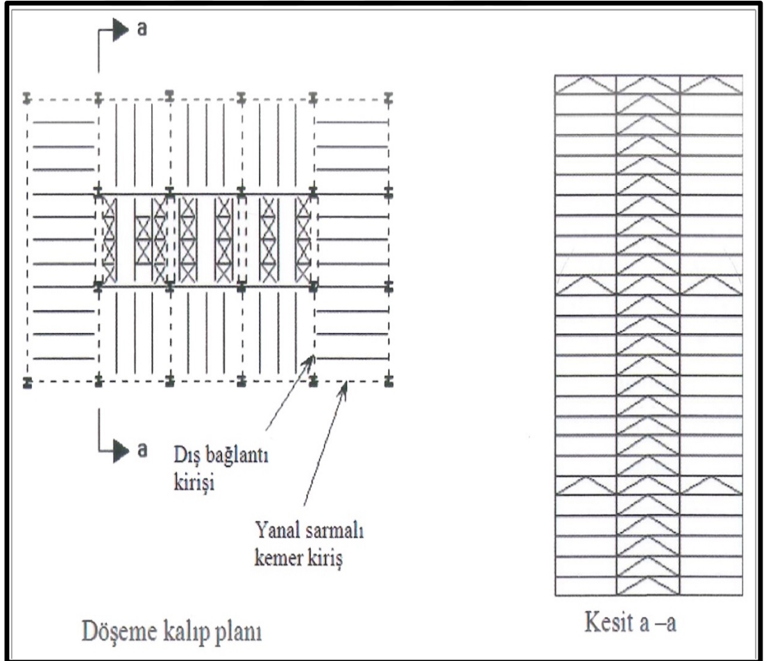
Şekil 3.45: Çekirdek ve Yanal Sarmalı Sistemin Plan ve Kesitinden Bir Örnek (Çelik inşaat için) (Sağlam, 2016)
