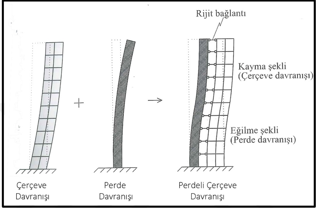
Şekil 3.24: Perdeli Çerçeve Sistemin Yanal Yükler Altında Davranışı
