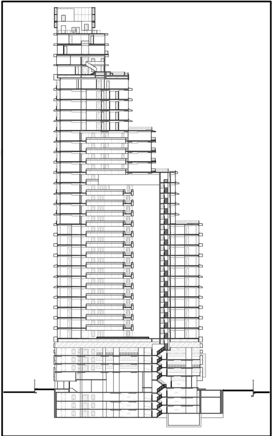
Şekil 5.53: Saladaeng One Kesit (URL- 55)
