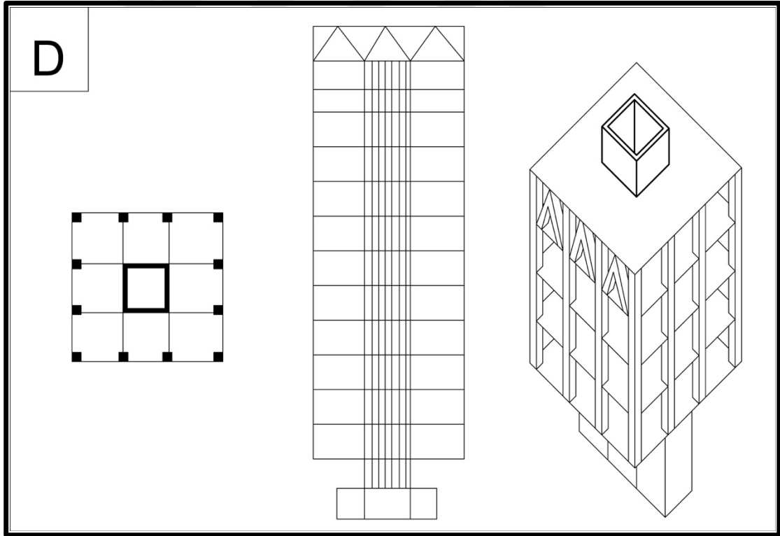
Şekil 4.34: Çekirdek ve Asma Sistem (Özgen ve Sev, 2000) (Şekil 4. 25D)
