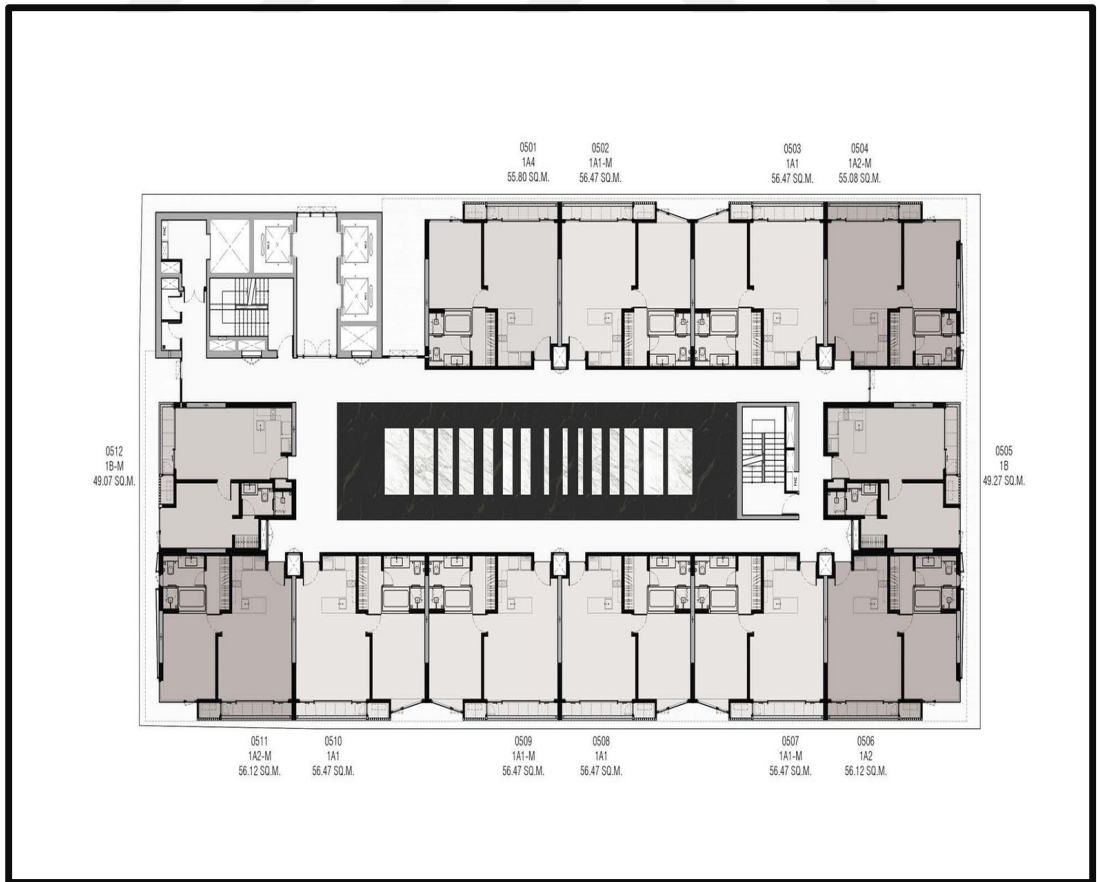
Şekil 5.49: Saladaeng One Normal Kat Planı (URL- 55)
