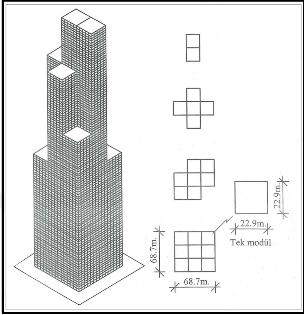
Şekil 3.75: Tüp Sistem
