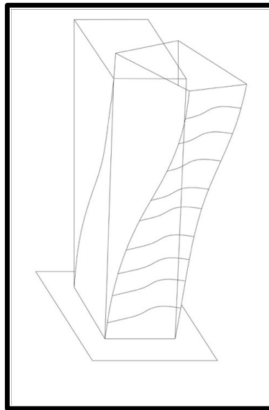
Őekil 4.17: ekirdek Burulması
