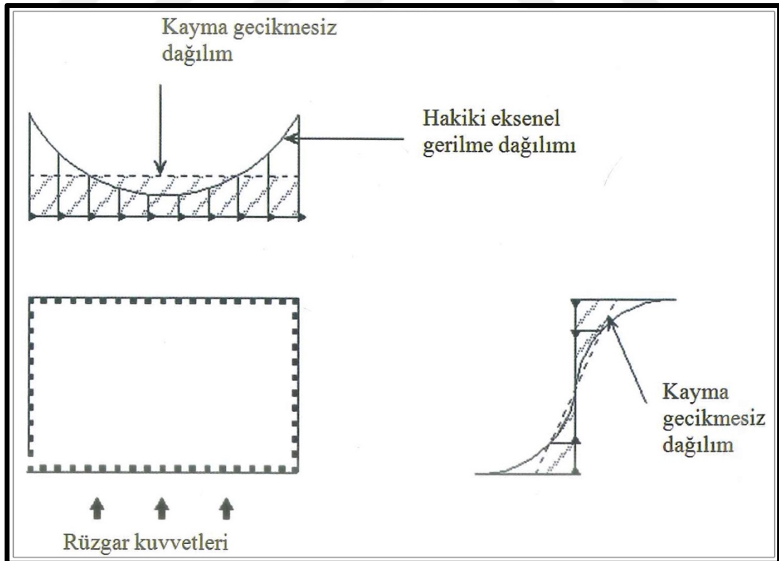
Şekil 3.64: Çerçeve Tüp' teki çevre kolonlarında aksenal kuvvetin dağılımı (Günel, Ilgın, 2010)
