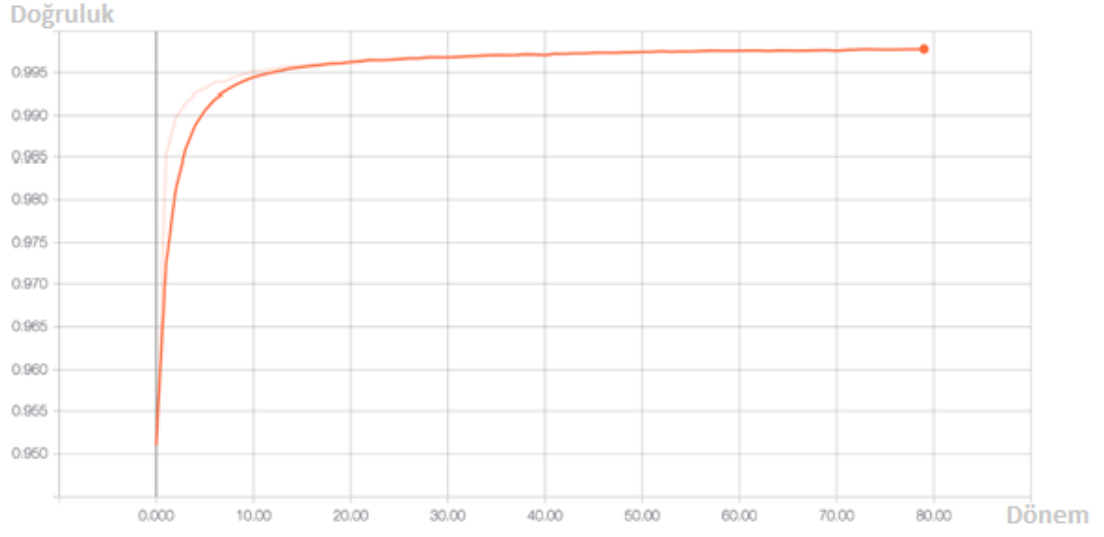
Şekil 3.28: CNN, Mnist test verileri dönem bazında doğruluk grafik sonucu
