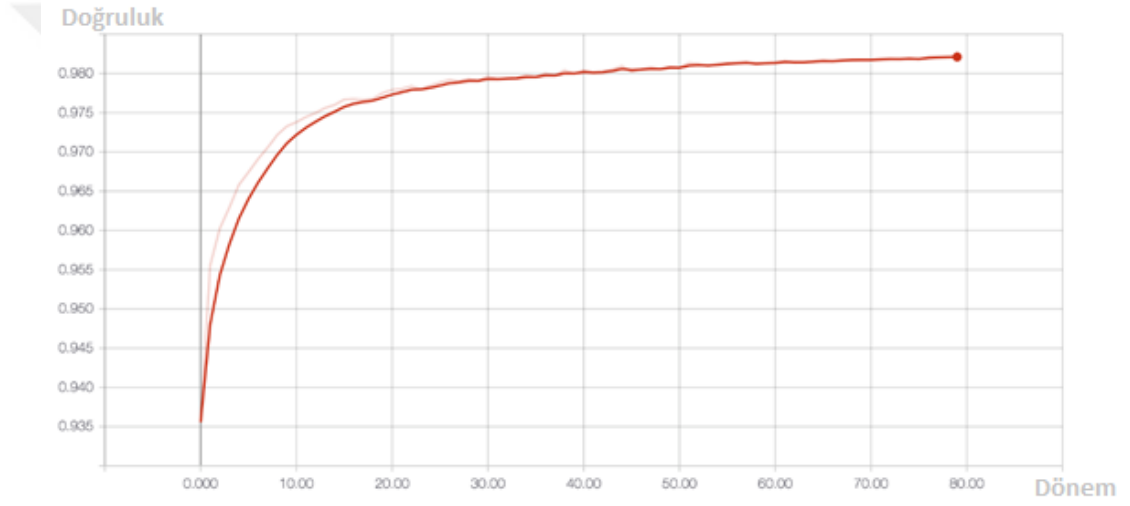
Şekil 3.20: CNN, Fashion-Mnist test verileri dönem bazında doğruluk grafik sonucu
