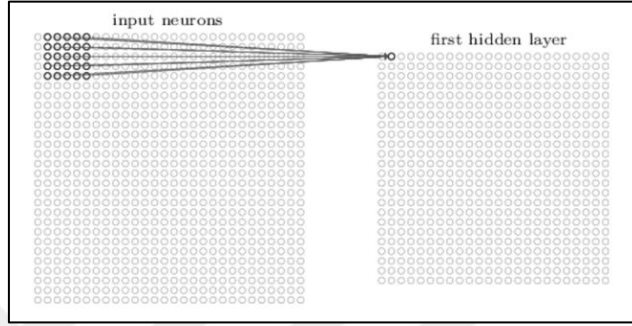
Şekil 2.7: İlk gizli katmandaki ikinci bölgesel nöron karşılığı
