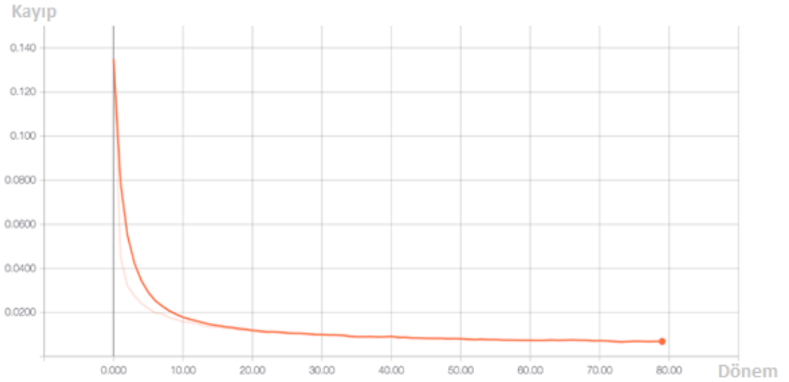
Şekil 3.29: CNN, Mnist test verileri dönem bazında kayıp grafik sonucu
