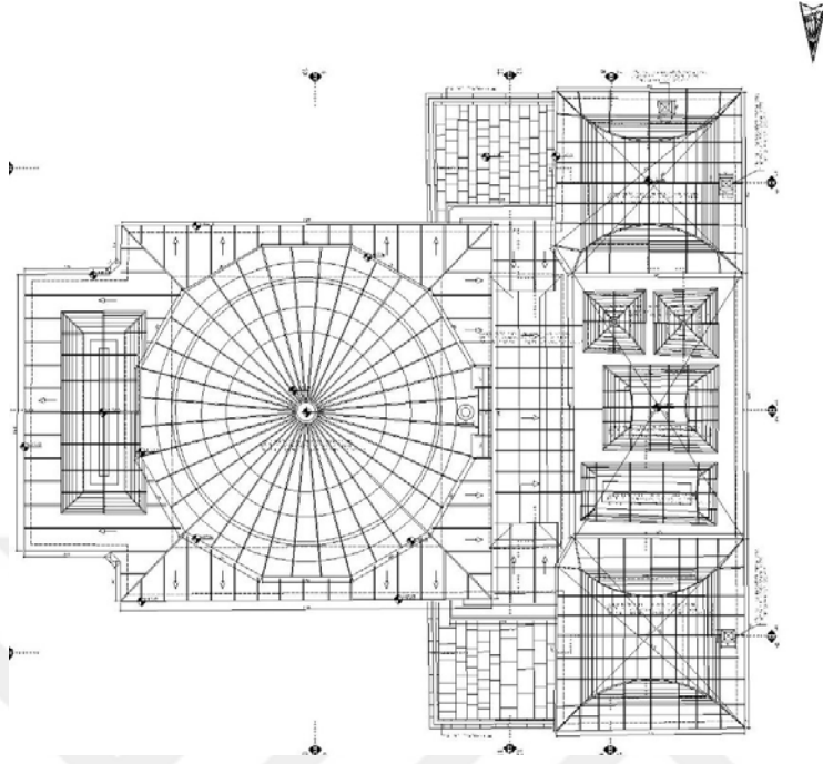
EK 2-A: Hünkâr Kasrı, Çatı Planı. (2010 yılı restorasyon çizimleri, Y. T. Ü.- Yapı İşleri ve Teknik Daire Başkanlığı, Mimari Büro' nun Proje Arşivinden)
