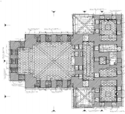
Şekil 3.26.Hünkâr Kasrı, Zemin Kat Planı. (2010 yılı restorasyon çizimleri, Y. T. Ü.- Yapı İşleri ve Teknik Daire Başkanlığı, Mimari Büro' nun Proje Arşivinden)
