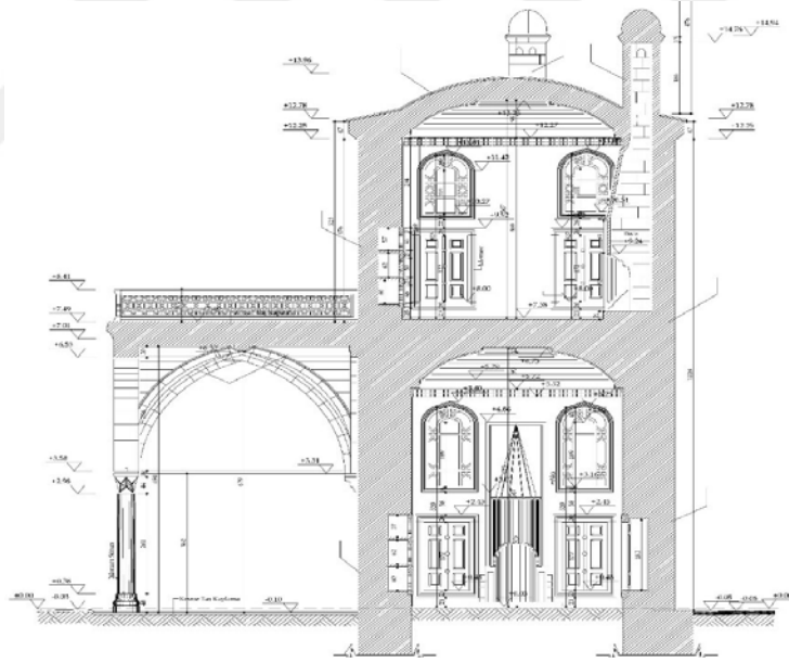
EK 2-Ç: Hünkâr Kasrı, 3-3 Kesiti. (2010 yılı restorasyon çizimleri, Y. T. Ü.- Yapı İşleri ve Teknik Daire Başkanlığı, Mimari Büro' nun Proje Arşivinden)
